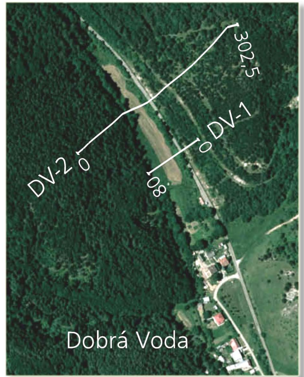
Situácia profilov DV-1 a DV-2, M 1 : 5 000
