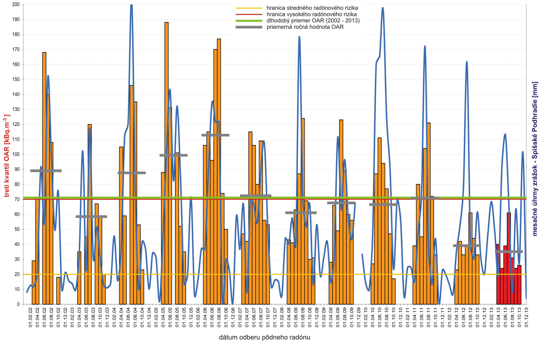
Obr. č. 2 Pôdny radón: monitorovanie objemovej aktivity radónu (OAR) v rokoch 2002 - 2013 Lokalita: Novoveská Huta
