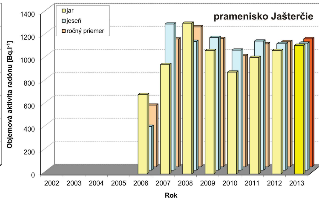
Obr. č. 8 Radón vo vodách: monitorovanie objemovej aktivity radónu (OAR) v rokoch 2002 - 2013 Lokality: Bratislava - pramene Mária, Himligárka, Zbojníčka; Oravice - pramenisko Jašterčie
