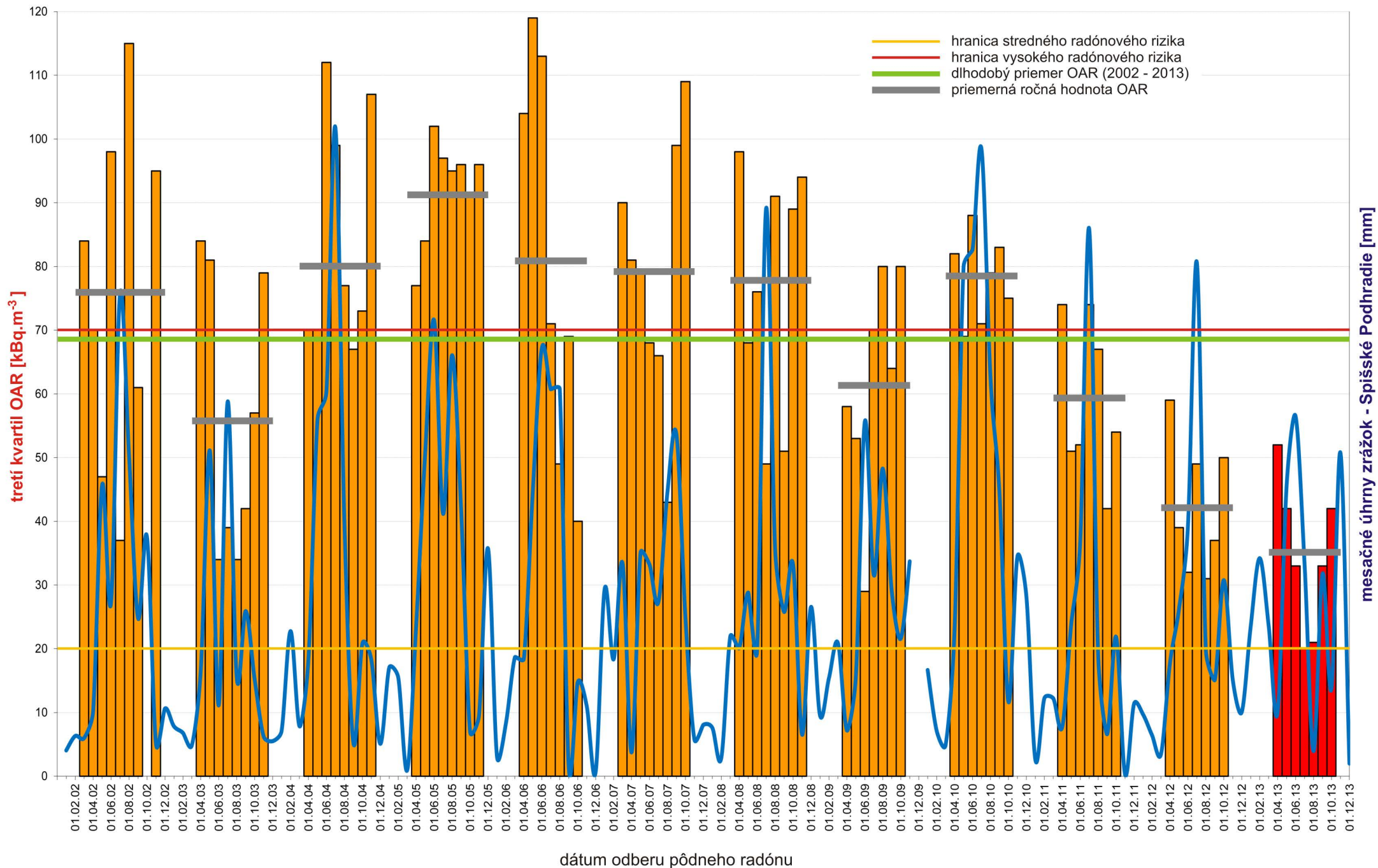
Obr. č. 3 Pôdny radón: monitorovanie objemovej aktivity radónu (OAR) v rokoch 2002 - 2013 Lokalita: Teplička
