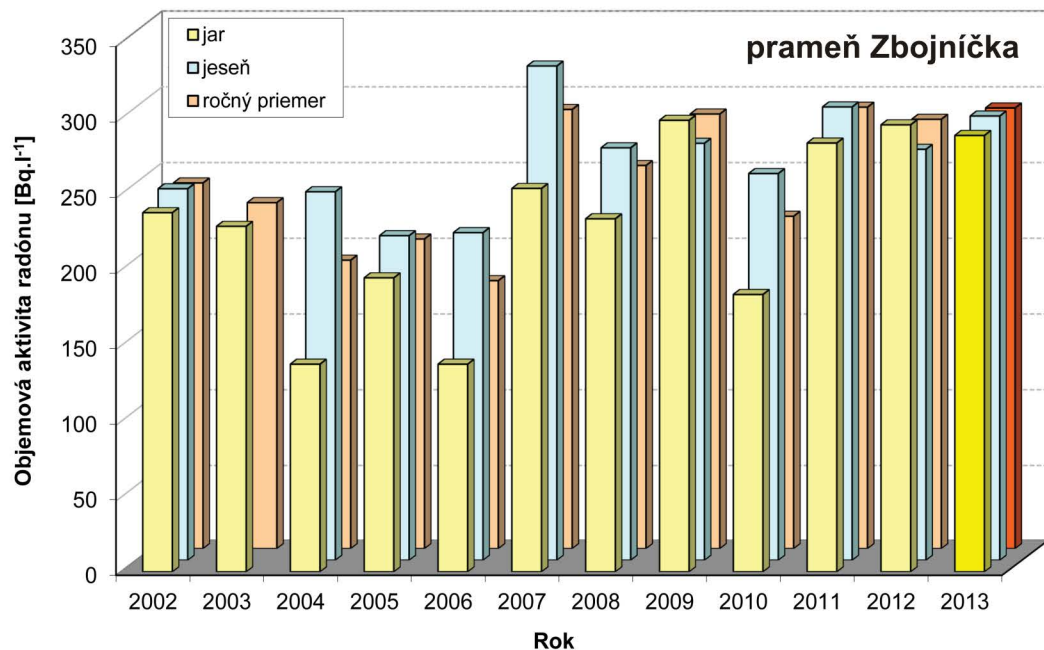
Obr. č. 8 Radón vo vodách: monitorovanie objemovej aktivity radónu (OAR) v rokoch 2002 - 2013 Lokality: Bratislava - pramene Mária, Himligárka, Zbojníčka; Oravice - pramenisko Jašterčie
