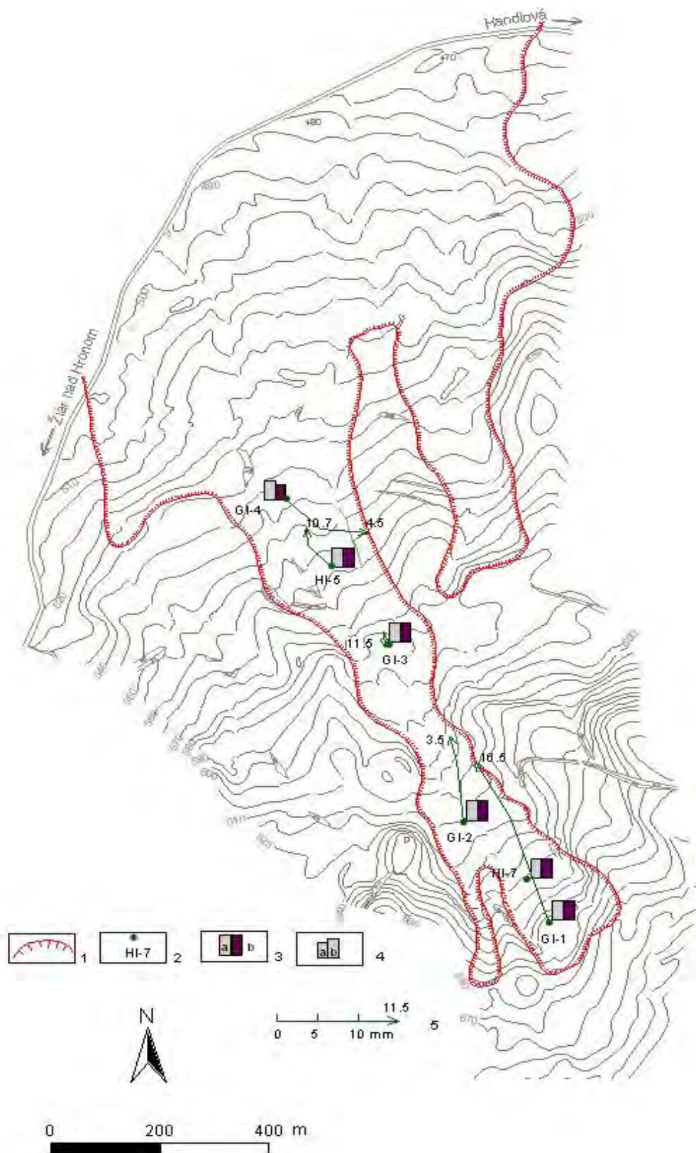
Obr. 2.1.39: Lokalita Handlová – zosuv z roku 1960 – výsledky inklinometrických meraní a merania poľa PEE v roku 2006. 1 – ohraničenie zosuvu, 2 – inklinometrické vrty v reprezentatívnom profile, 3 – aktivita poľa PEE v rokoch: a – 2005, b – 2006, 4 – hodnotenie poľa PEE podľa kritérií, zhrnutých v tab. 2.1.4: a – nízka aktivita poľa PEE (stupeň 1), b – stredná aktivita poľa PEE (stupeň 2), 5 – mierka vektora deformácie inklinometrickej pažnice za obdobie IV.03-V. 05-IX.06 (číslo označuje hĺbku zaznamenatej deformácie od povrchu terénu v m)
