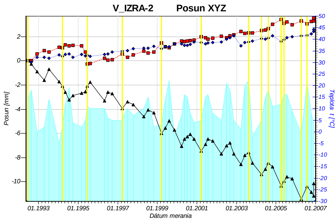
Obr. 2.1.83: Výsledky dlhodobého merania posunov horninových blokov dilatometrami TM-71 na lokalite Veľká Izra
