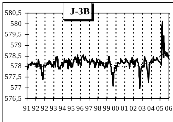
Obr. 2.1.57: Maximá hladiny podzemnej vody v roku 2006 v niektorých piezometroch
