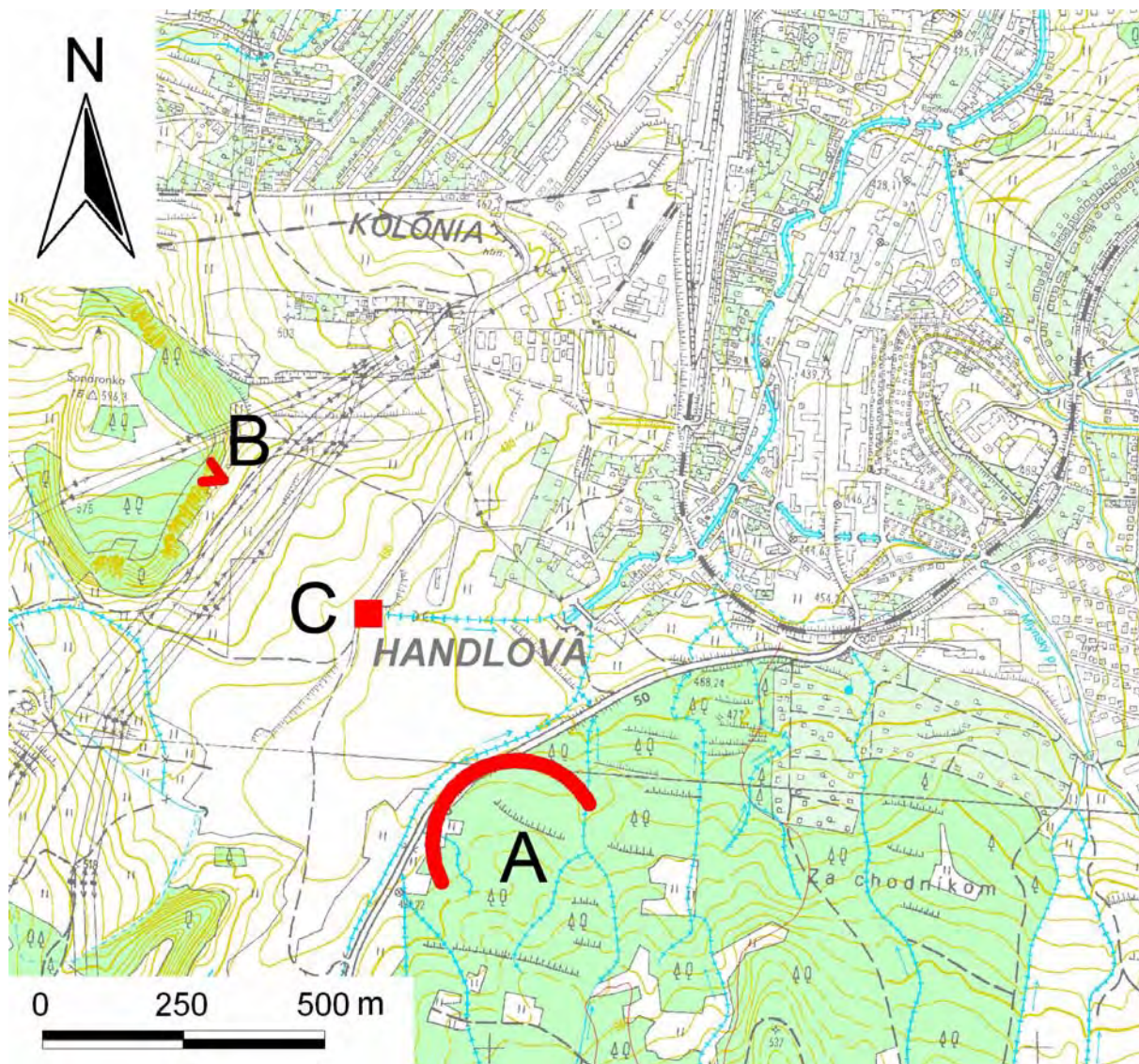
Obr. 2.1.38: Lokalizácia monitorovaných objektov na južnom okraji mesta Handlová. A – katastrofálny handlovský zosuv; zosuvná značka je v čele zosuvnej akumulácie, B – stanovisko pre monitorovanie rýchlosti zvetrávania a rozpadu horninového masívu, C – čelo Stabilizačného násypu
