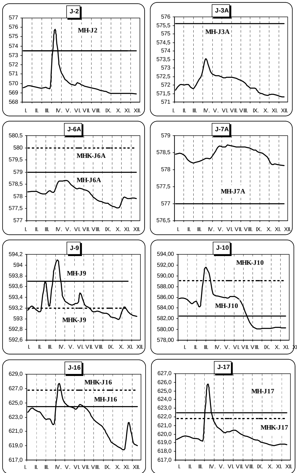
Obr. 2.1.58: Kolísanie hladín podzemných vôd (m.n.m) vo vybraných piezometroch v roku 2006 a ich vzťah k medznej hodnote MH podľa HYCO (1980) a MHK podľa Kopecký (2002)
