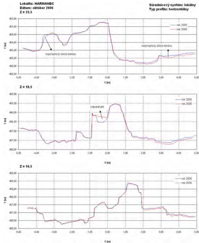
Obr. 2.1.108: Porovnanie konfigurácie steny v profiloch PF2 (23,5 m), PF6 (18,5 m), a PF8 (16,5 m), zameraných v rokoch 2005 a 2006 stereofotogrametrickou metódou na lokalite Harmanec
