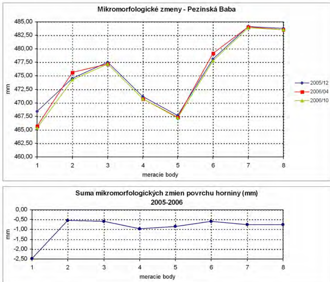
Obr. 2.1. 118: Výsledky merania mikromorfologických zmien povrchu skalnej steny na lokalite Pezinská Baba
