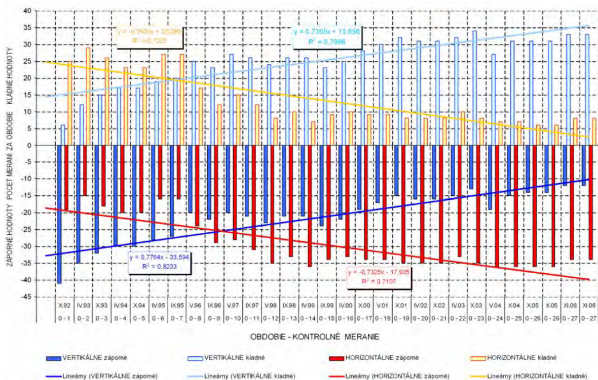
Obr.2.1.124: Štatistické vyhodnotenie výsledkov merania deformácií potrubia SN za obdobie rokov 1992 až 2006
