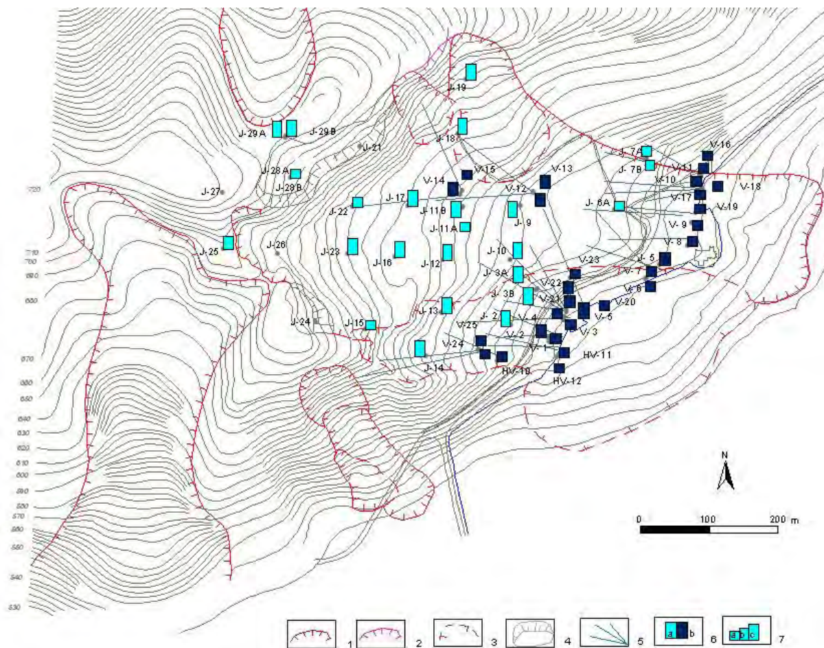
Obr. 2.1.54: Lokalita Liptovská Mara – výsledky režimových pozorovaní v rokoch 2005 a 2006. 1 – ohraničenie aktívnych zosuvov, 2 – staršie potenciálne zosuvy, 3 – ohraničenie mladších dielčích zosuvov, 4 – blokové polia, 5 – horizontálne odvodňovacie vrty, 6 – režimové pozorovania v roku 2006: a – zmeny hĺbky hladiny podzemnej vody, b – výdatnosť odvodňovacích zariadení, 7 – hodnotenie režimových pozorovaní podľa kritérií, zhrnutých v tab. 2.1.5: a – stav priaznivý (stupeň 1) pri vertikálnych vrtoch, resp. priem. výdatnosť do 1 \text{ l.min}^{-1} horizontálnych vrtoch, b – náznaky nepriaznivého stavu (2), resp. priem. výdatnosť 1 až 3 \text{ l.min}^{-1} , c – stav nepriaznivý (3)
