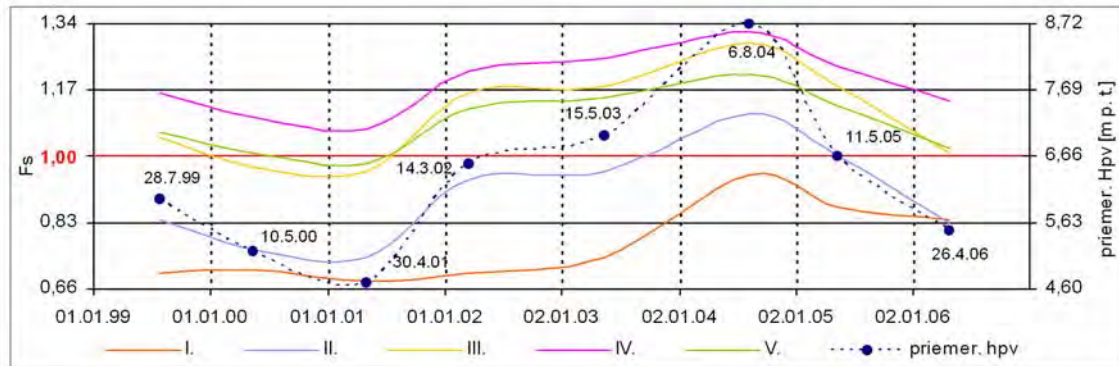
Obr. 2.1.49: Výsledky stabilitných výpočtov v profiloch 1-1' na lokalite Okoličné
