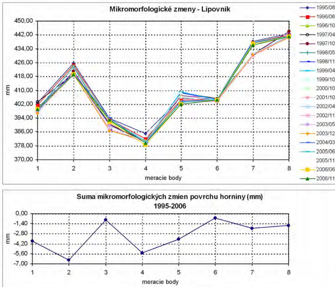
Obr. 2.1.121: Výsledky dlhodobého merania mikromorfologických zmien povrchu odkryvu na lokalite Lipovník
