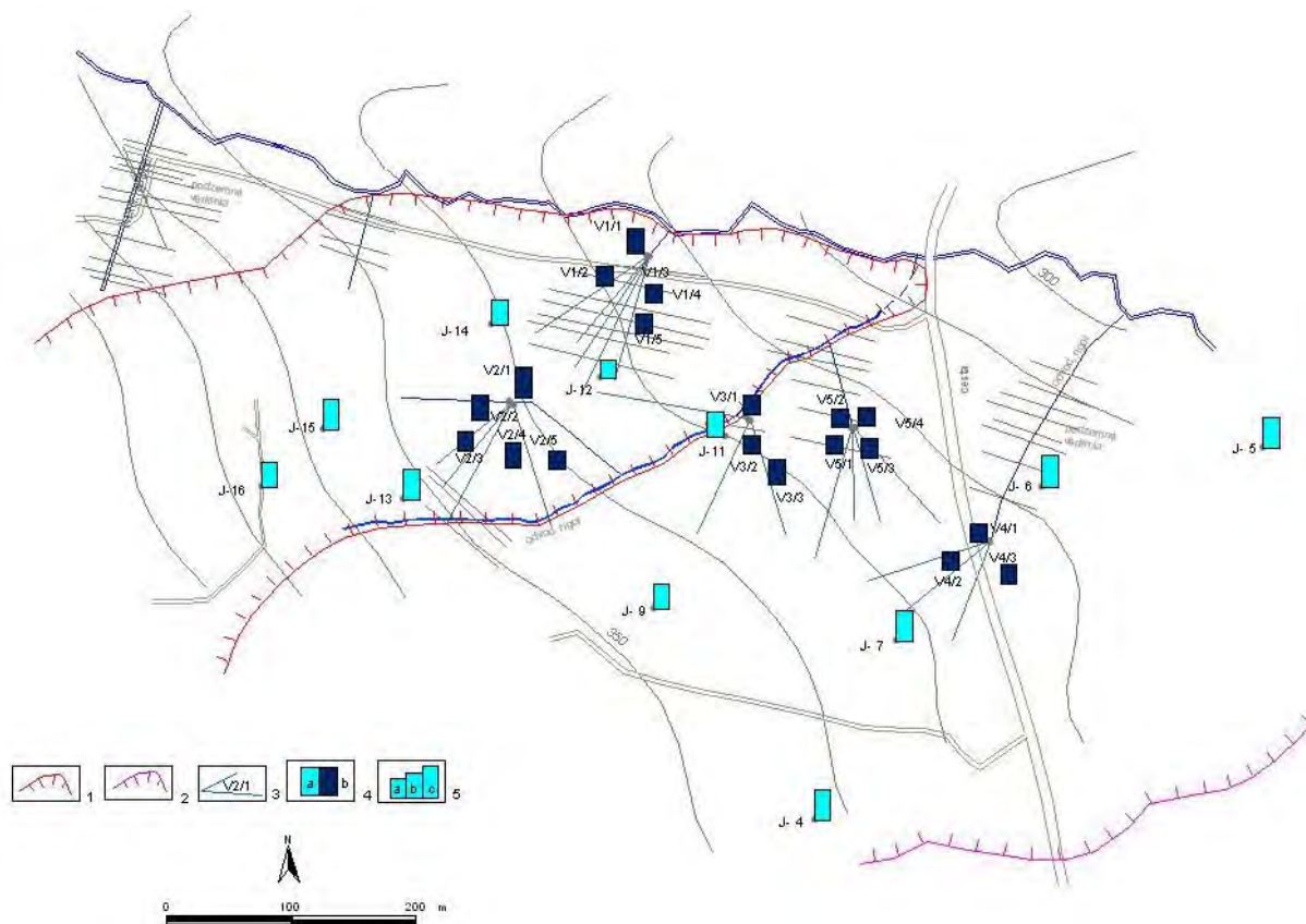
Obr. 2.1.36: Lokalita Slanec – TP. Situácia sanačných a monitorovacích objektov a výsledky režimových pozorovaní. 1 – ohraničenie časti aktívneho zosuvu, 2 – ohraničenie časti potenciálneho zosuvu, 3 – vejáre horizontálnych odvodňovacích vrtov, 4 – režimové pozorovania v roku 2006: a – zmeny hĺbky hladiny podzemnej vody, b – výdatnosť odvodňovacích zariadení, 5 – hodnotenie režimových pozorovaní podľa kritérií, zhrnutých v tab. 2.1.5: a – stav priaznivý (stupeň 1) vo vertikálnych vrtoch, resp. priem. výdatnosť do 1 l.min -1 v horizontálnych vrtoch, b – náznaky nepriaznivého stavu (stupeň 2), resp. priemerné výdatnosť 1 až 3 l.min -1 , c - stav nepriaznivý (stupeň 3), resp. priemerná výdatnosť nad 3 l.min -1
