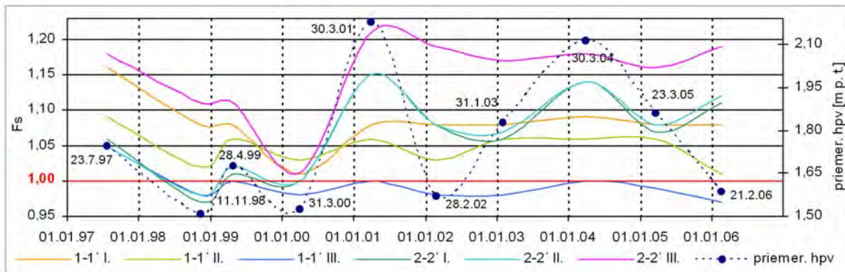
Obr. 2.1.67: Výsledky stabilitných výpočtov v profiloch 1-1' a 2-2' na lokalite Bojnice
