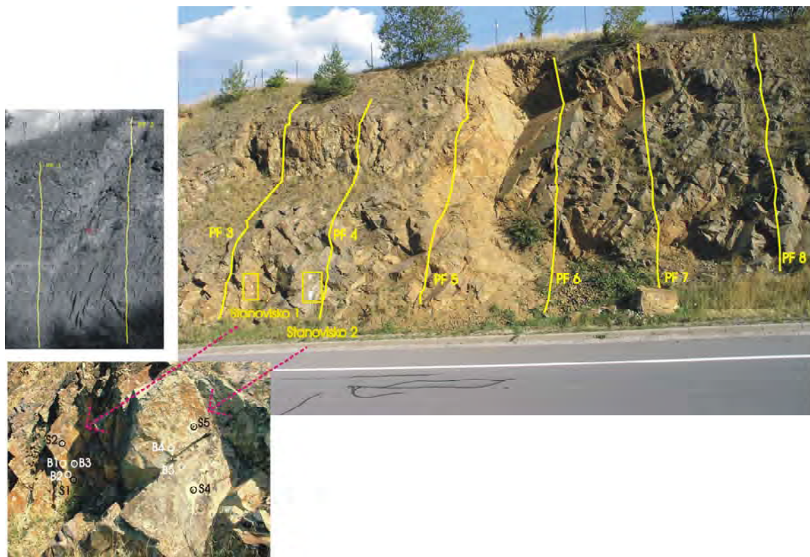
Obr. 2.1.91: Rozmiestnenie pozorovaných profilov a bodov na monitorovanom úseku zárezu cesty pri Banskej Štiavnici. PF1 až PF8 – profily pre stereofotogrametrické merania, B1 až B5 – pozorovacie body pre merania dilatometrom Somet, S1, S2, S4, S5 – pozorovacie body pre merania meradlom posuvov. Stanovisko merania mikromorfologických zmien povrchu skalnej steny sa nachádza cca 30 m V od profilu PF1
