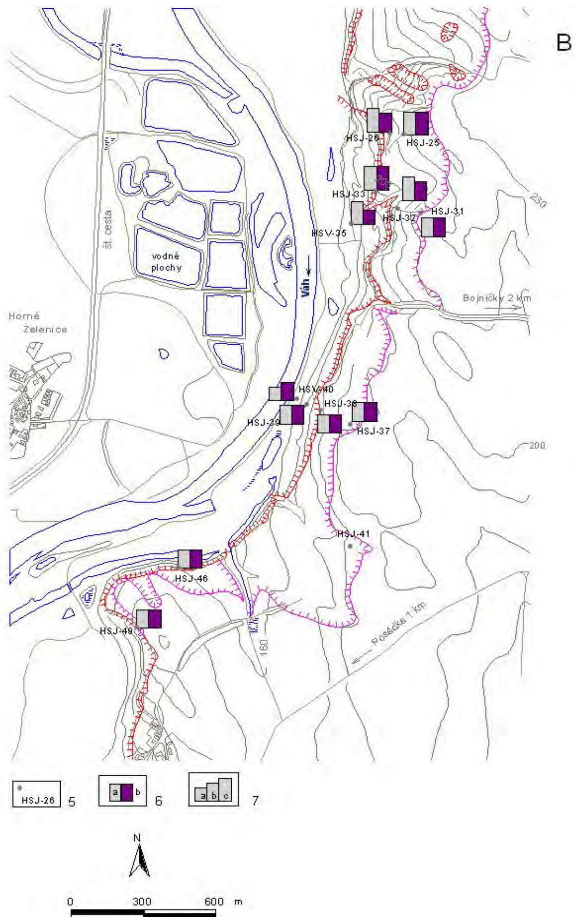
Obr. 2.1.73B: Lokalita Hlohovec-Posádka – výsledky merania poľa PEE. 5 – meracie vrty, 6 – aktivita poľa PEE v rokoch: a – 2005, b – 2006, 7 – hodnotenie aktivity poľa PEE podľa kritérií tab. 2.1.4: a – nízka aktivita poľa (stupeň 1), b - stredná aktivita poľa (stupeň 2), c – vysoká aktivita poľa (stupeň 3)
