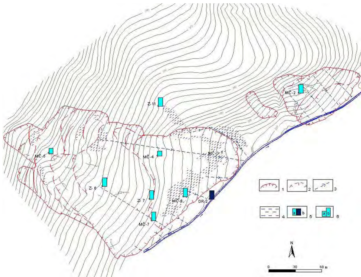
Obr. 2.1.79: Lokalita Malá Čausa – výsledky režimových pozorovaní v roku 2006. 1 – ohraničenie aktívnych zosuvov, 2 – dlhšie zosuvy a zátrhy, 3 – stabilizačno - odvodňovacie rebrá, 4 – zamokrené územia, 5 – režimové pozorovania v roku 2006: a – zmeny hĺbky hladiny podzemnej vody, b – výdatnosť odvodňovacieho zariadenia, 6 – hodnotenie režimových pozorovaní podľa kritérií, zhrnutých v tab. 2.1.5: a – stav priaznivý (stupeň 1) u vertikálnych vrtov, b – stav nepriaznivý (stupeň 3), resp. výdatnosť drénu nad 3 \text{ l.min}^{-1}
