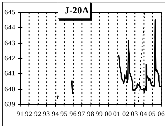
Obr. 2.1.57: Maximá hladiny podzemnej vody v roku 2006 v niektorých piezometroch
