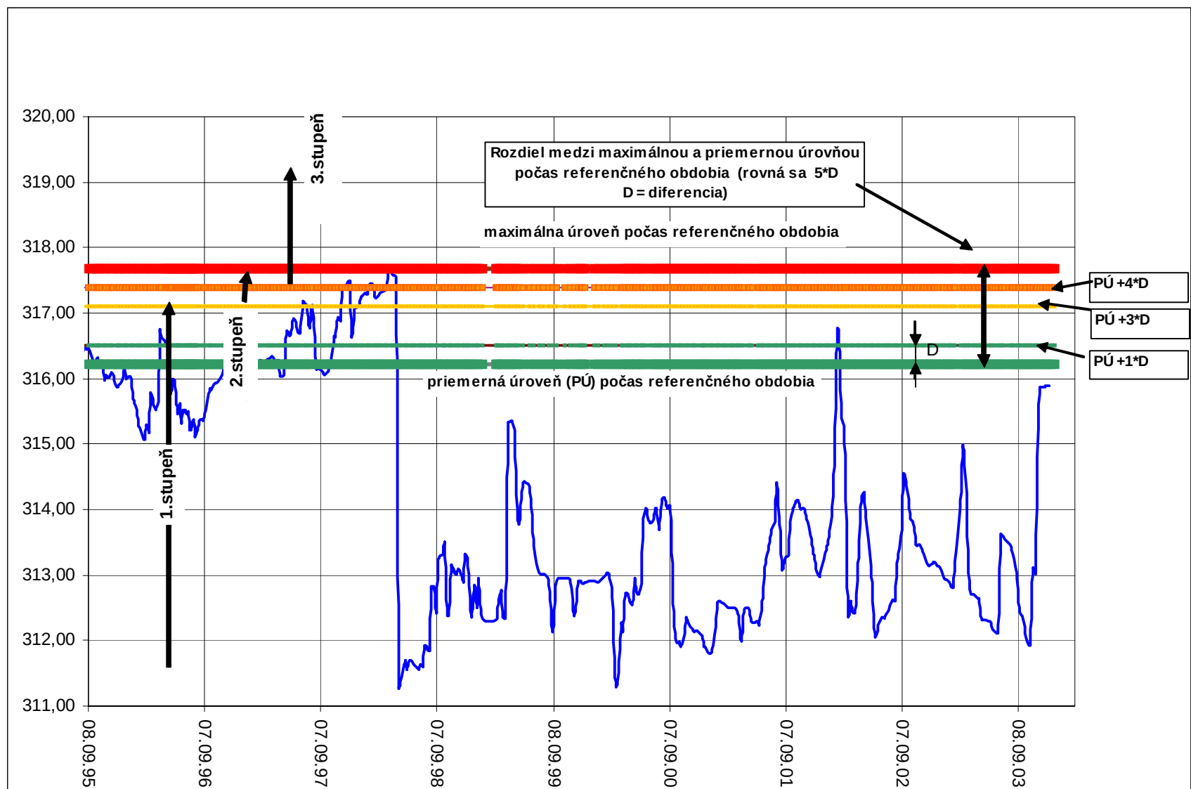
Obr. 2.1.2: Postup odvodenia referenčných hodnôt pre semikvantitatívne hodnotenie zmien úrovne hladiny podzemnej vody, obsiahnuté v tab. 2.1.5 (záznam z pozorovania hladiny podzemnej vody vo vrte VČ-4 z lokality Veľká Čausa - zostavil S. Scherer, 2004)
