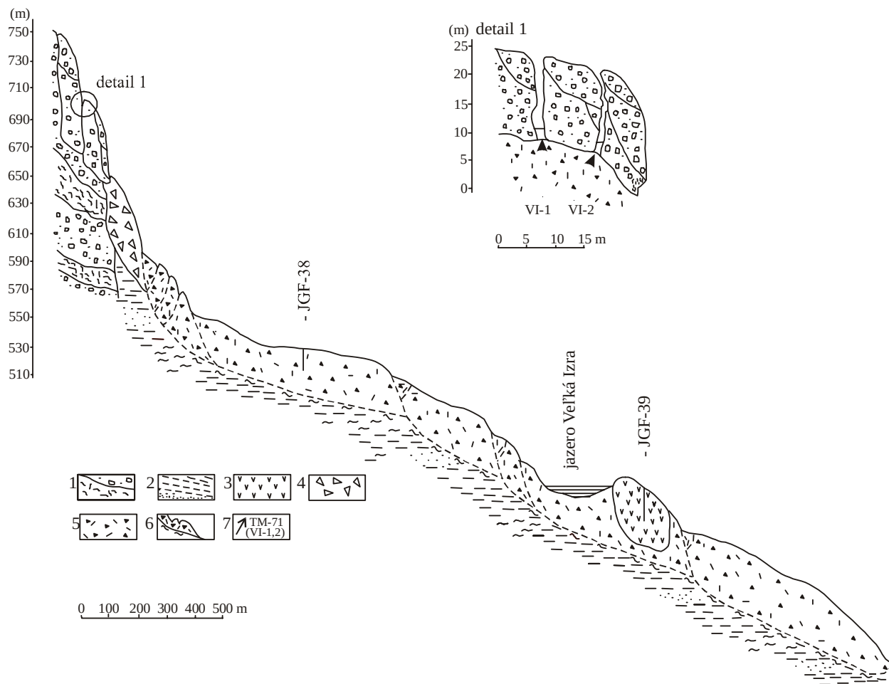
Obr. 2.1.82: Inžinierskogeologický rez svahovou deformáciou na lokalite Veľká Izra s vyznačením osadenia dilatometrov VI-1 a VI-2. 1 – striedanie andezitov a brekcií lávových prúdov s polohami autochtónnych pyroklastík, 2 – íl s polohami ílovitého piesku, 3 – ryolit (zosunutý blok), 4 – morfológicky nečlenené – blokové pole, 5 – balvanité a úlomkovito-ílovité svahové sedimenty (sute), 6 – priebeh šmykovej plochy 7 – lokalizácia dilatometrov TM-71 (VI-1 a VI-2).
