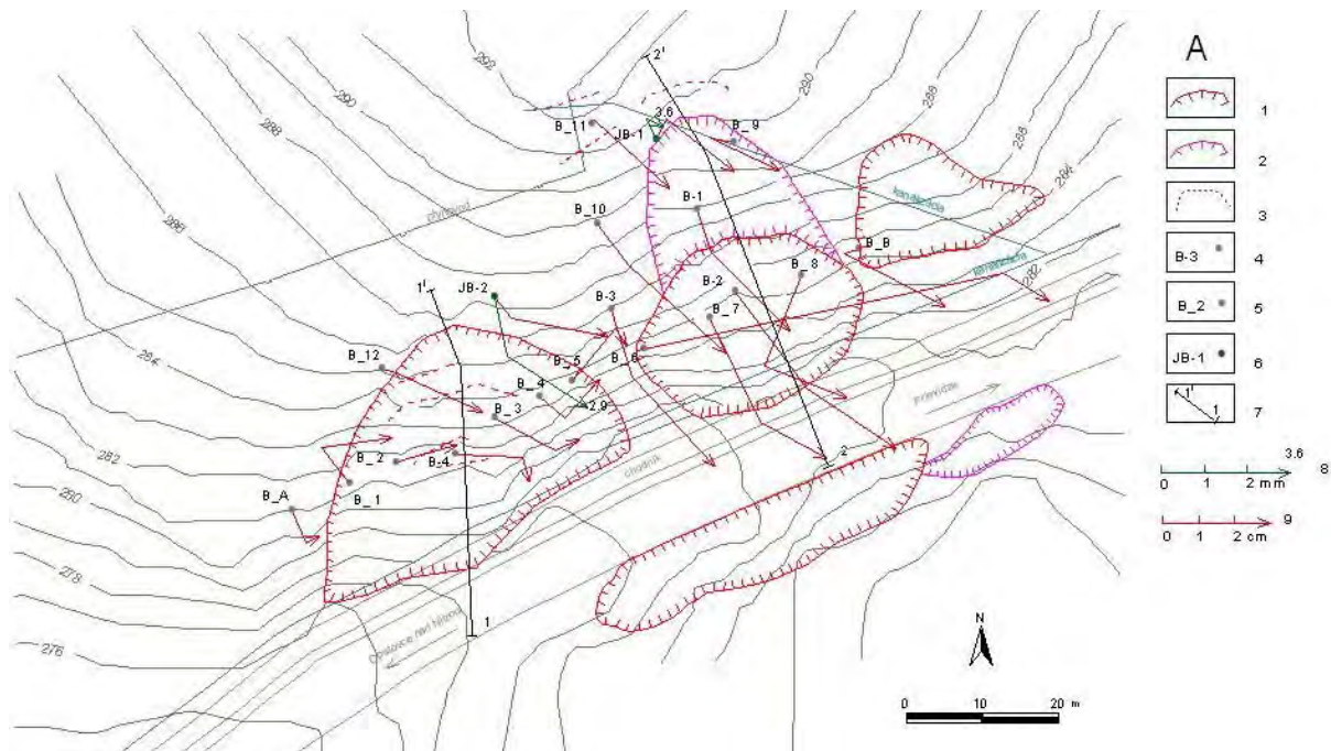
Obr. 2.1.63A: Lokalita Bojnice – výsledky geodetických a inklinometrických meraní v rokoch 2005 a 2006. 1 – ohraničenie aktívnych zosuvov z rokov 1995 až 1999, 2 – ohraničenie potenciálnych zosuvov, 3 – zosuvné trhliny, 4 – piezometrické vrty, 5 – geodetické pozorovacie body, 6 – inklinometrické vrty, 7 – línie profilov pre stabilné výpočty, 8 – mierka vektorov deformácie inklinometrickej pažnice za obdobie IV.04-V.05-V.06 (číslo označuje hĺbku zaznamenatej deformácie od povrchu terénu v m), 9 – mierka vektorov premiestnení geodetických bodov za obdobie V.04-V.05-VI.06
