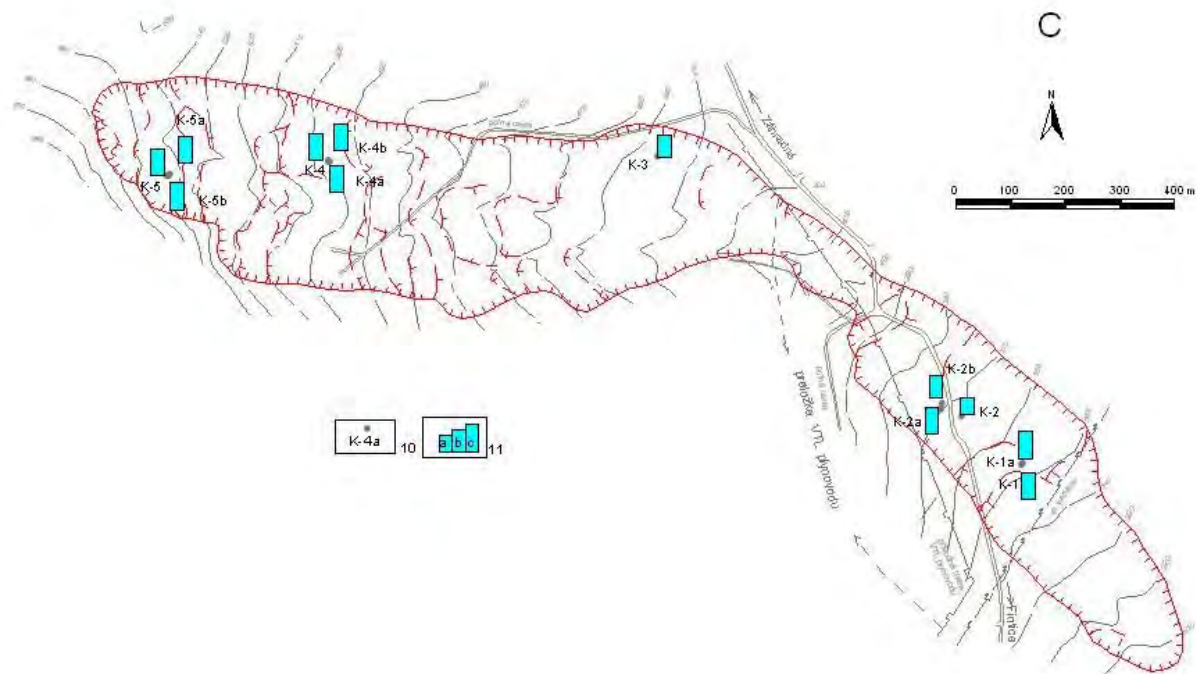
Obr. 2.1.21C: Lokalita Fintice – výsledky režimových pozorovaní. 10 – vrty v ktorých sa meria hĺbka hladiny podzemnej vody, 11 – hodnotenie zmien hĺbky hladiny podzemnej vody podľa kritérií, zhrnutých v tab. 2.1.5: a – stav priaznivý (stupeň 1), b – náznaky nepriaznivého stavu (2), c – stav nepriaznivý (stupeň 3)
