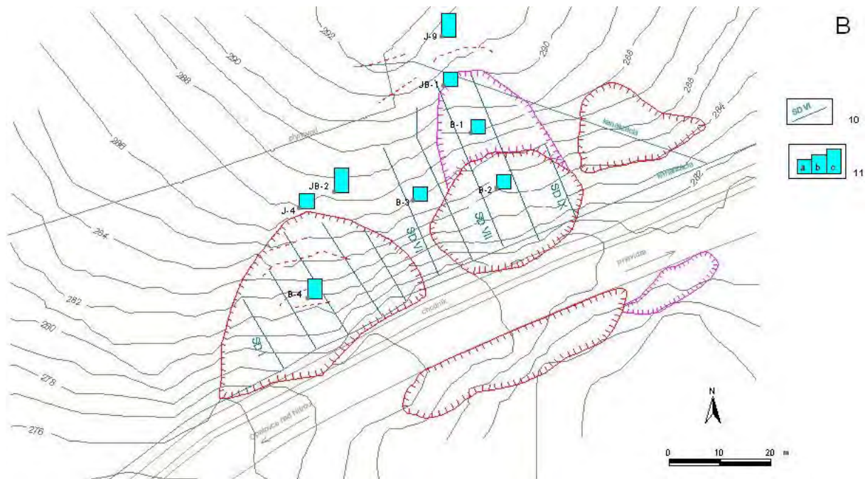
Obr. 2.1.63B: Lokalita Bojnice – výsledky režimových pozorovaní. 10 – odvodňovacie drény, 11 – hodnotenie zmien hĺbky hladiny podzemnej vody podľa kritérií, zhrnutých v tab. 2.1.5: a – stav priaznivý (stupeň 1), b – náznaky nepriaznivého stavu (stupeň 2), c – stav nepriaznivý (stupeň 3)
