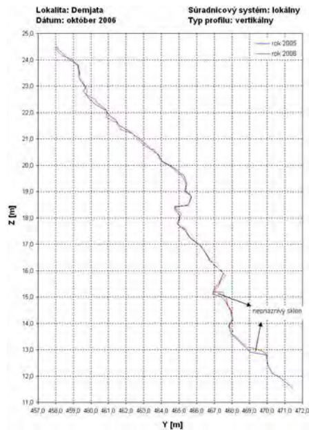
Obr. 2.1.97: Porovnanie konfigurácie steny v profile PF2, zameranom v rokoch 2005 a 2006 stereofotogrametrickou metódou na lokalite Demjata
