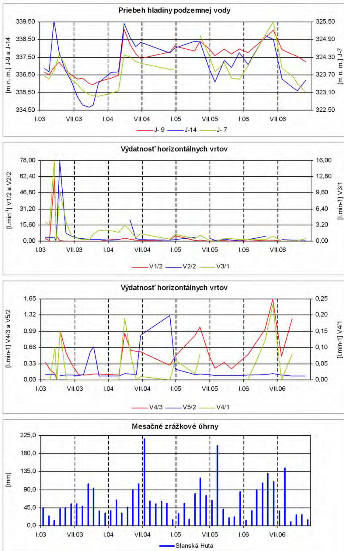
Obr. 2.1.37: Výsledky režimových pozorovaní vybraných objektov na lokalite Slanec v rokoch 2003 až 2006, znázornené spoločne s mesačnými úhrnmi zrážok zo stanice SHMÚ Slanská Huta
