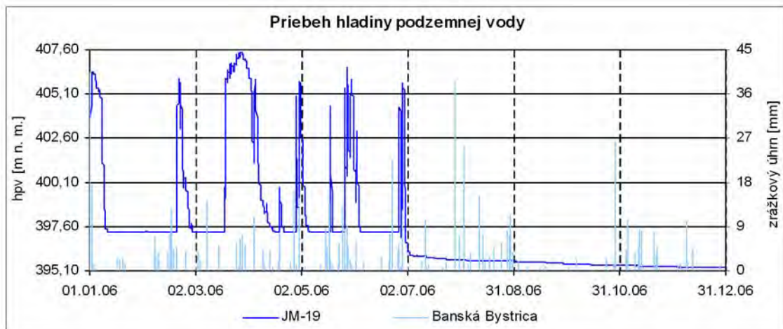
Obr. 2.1.30: Záznamy automatických hladinomerov umiestnených vo vrtoch JM-6 a JM-19 na lokalite Dolná Mičiná v roku 2006, znázornené spoločne s dennými úhrnmi zrážok zo stanice SHMÚ v Banskej Bystrici
