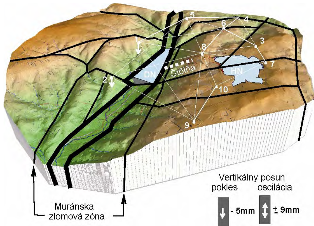
Obr. 2.1.128: Situácia bodov a tendencia pohybov zodpovedajúca súčtu hodnôt presahujúcich smerodajnú odchýlku za jednotlivé epochy. HN- horná nádrž, DN – dolná nádrž PVE (Korčák, 2004)
