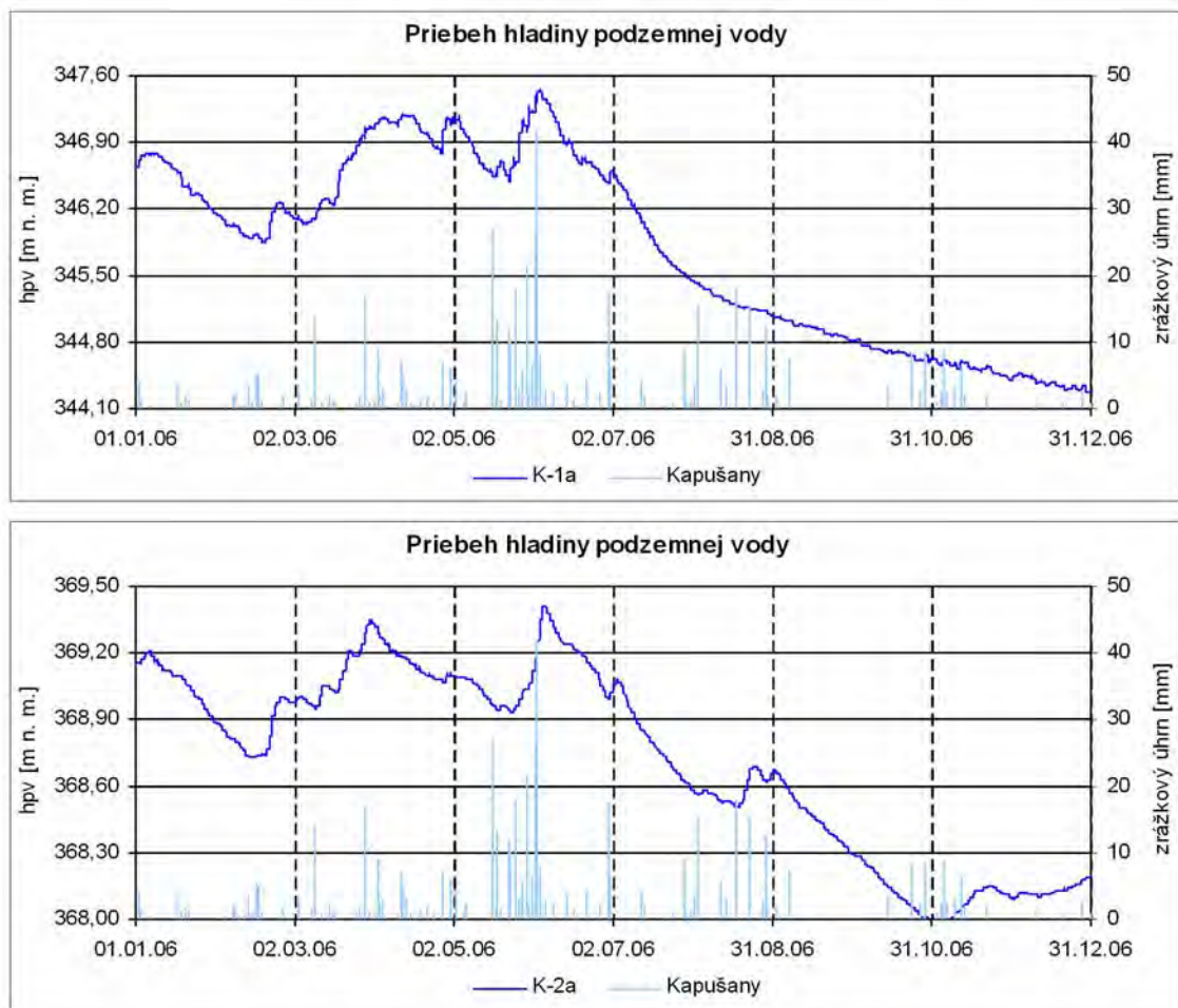
Obr. 2.1.23: Záznamy automatických hladinomerov umiestnených vo vrtoch K-1a a K-2a na lokalite Fintice v roku 2006, znázornené spoločne s dennými úhrnmi zrážok zo stanice SHMÚ Kapušany
