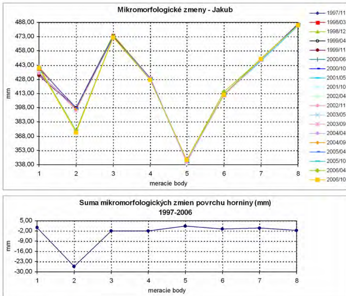
Obr. 2.1.112: Výsledky dlhodobého merania mikromorfologických zmien povrchu odkryvu na lokalite Jakub
