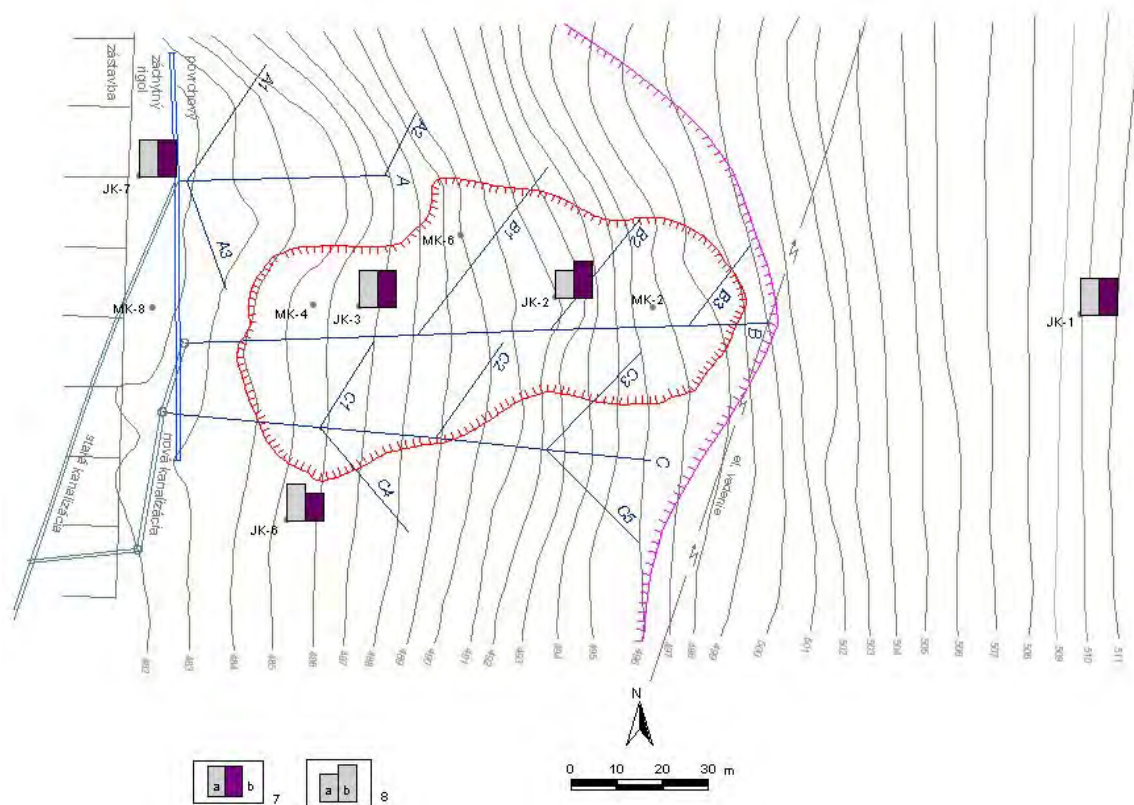
Obr. 2.1.17B – Lokalita Handlová – Kunešovská cesta. Výsledky merania poľa PEE. 7 – aktivita poľa PEE v rokoch: a – 2005, b – 2006, 8 – hodnotenie aktivity poľa PEE podľa kritérií tab. 2.1.4: a – nízka aktivita poľa (stupeň 1), b - stredná aktivita poľa (stupeň 2)
