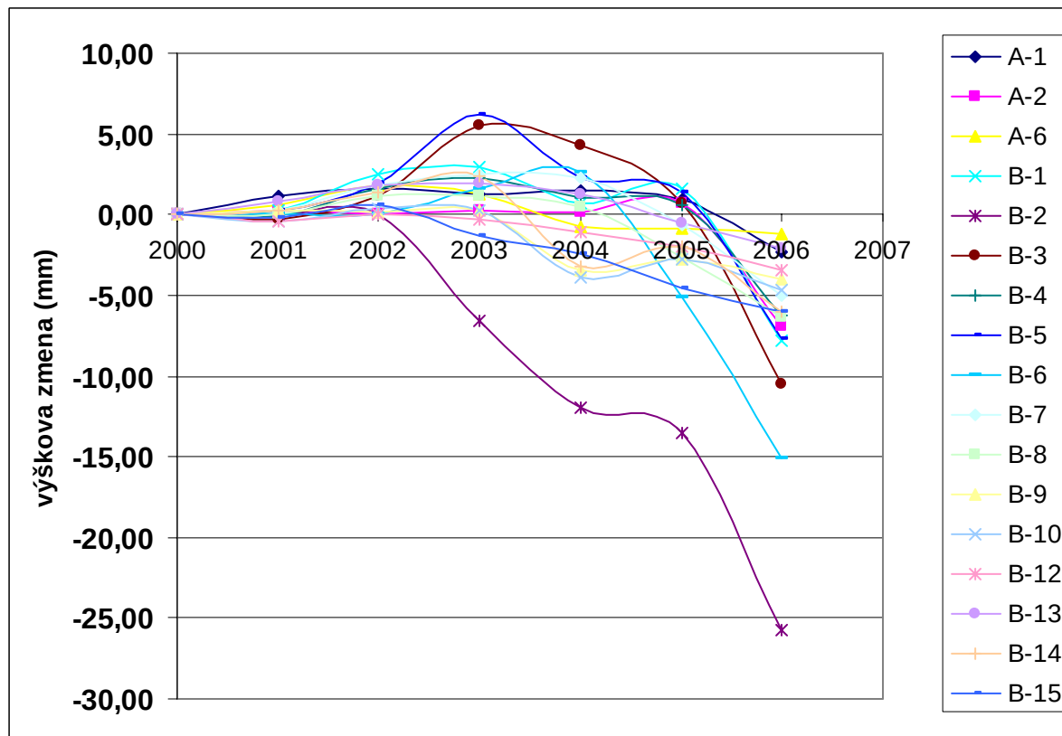
Obr. 2.1.53: Súčtové čiary výškových zmien pevných a pozorovaných bodoch za roky 2000 až 2006
