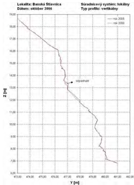
Obr. 2.1.92: Porovnanie konfigurácie steny v profile PF4, zameranom v rokoch 2005 a 2006 stereofotogrametrickou metódou na lokalite Banská Štiavnica
