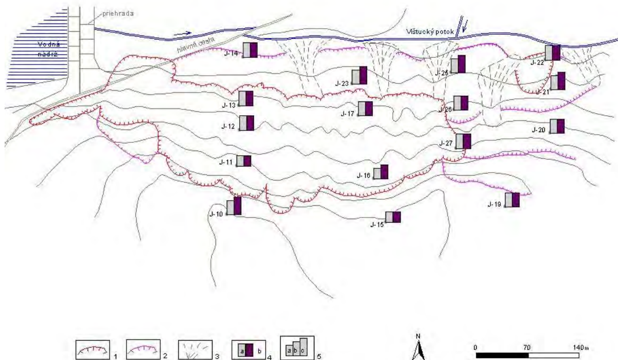
Obr. 2.1.76: Lokalita Vištuk – výsledky merania poľa PEE. 1 – ohraničenie aktívnych zosuvov, 2 – staršie potenciálne zosuvy, 3 – náplavové kužele, 4 – hodnotenie aktivity poľa PEE v rokoch: a – 2005, b – 2006, 5 – hodnotenie aktivity poľa PEE podľa kritérií tab. 2.1.4: a – nízka aktivita poľa (stupeň 1), b – stredná aktivita poľa (stupeň 2), c – vysoká aktivita poľa (stupeň 3)
