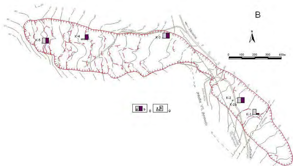
Obr. 2.1.21B: Lokalita Fintice – výsledky merania poľa PEE. 8 – aktivita poľa PEE v rokoch: a – 2005, b – 2006, 9 – hodnotenie poľa PEE podľa kritérií, zhrnutých v tab. 2.1.4: a – namerané, b – stredná aktivita poľa PEE (stupeň 2)
