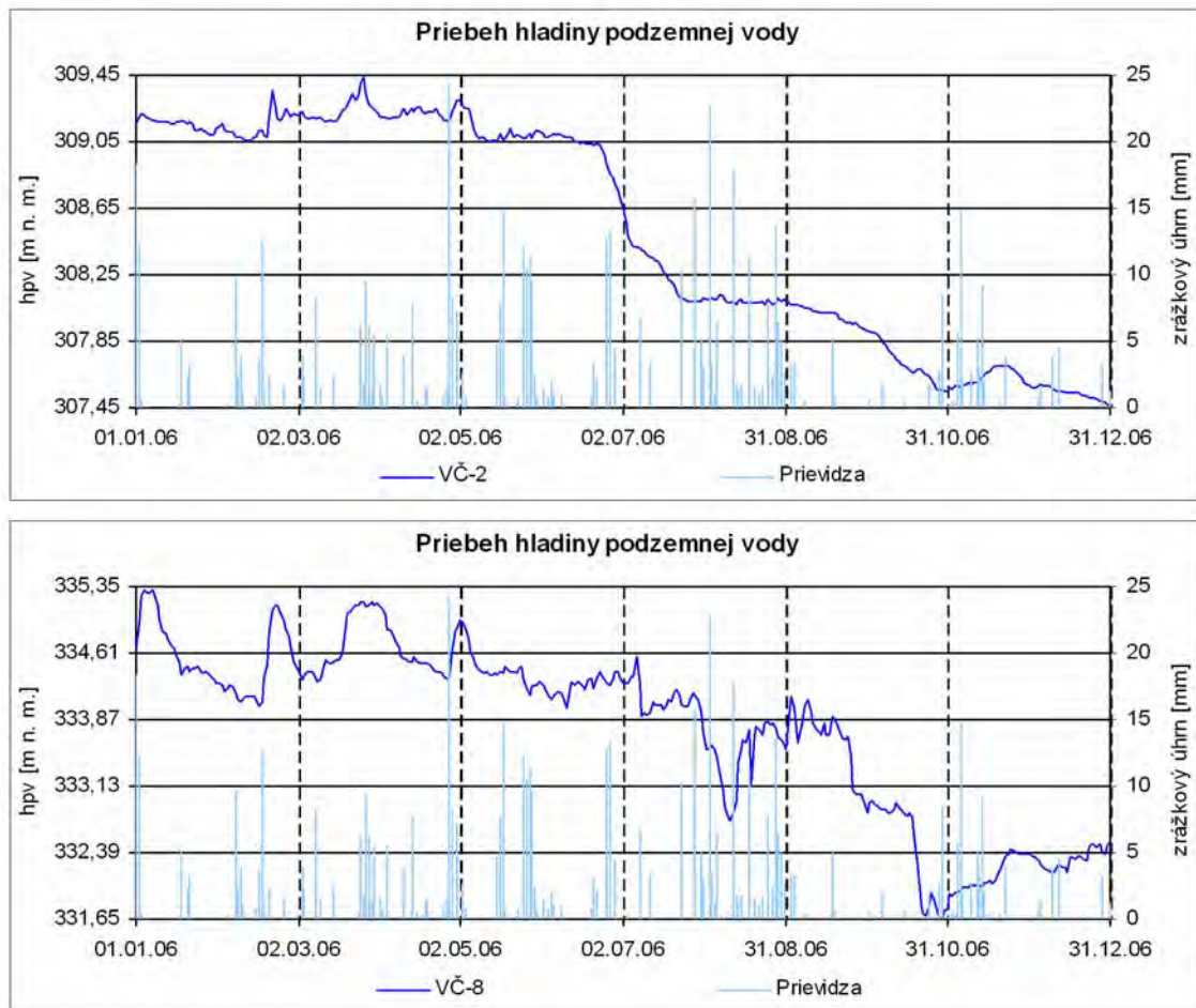
Obr. 2.1.6: Priebeh zmien úrovne hladiny podzemnej vody (HPV), zaznamenaný v roku 2006 automatickými hladinomerami, umiestnenými vo vrtoch VČ-2 a VČ-8 na lokalite Veľká Čausa spoločne so znázornením denných zrážkových úhrnov zo stanice SHMÚ v Prievidzi
