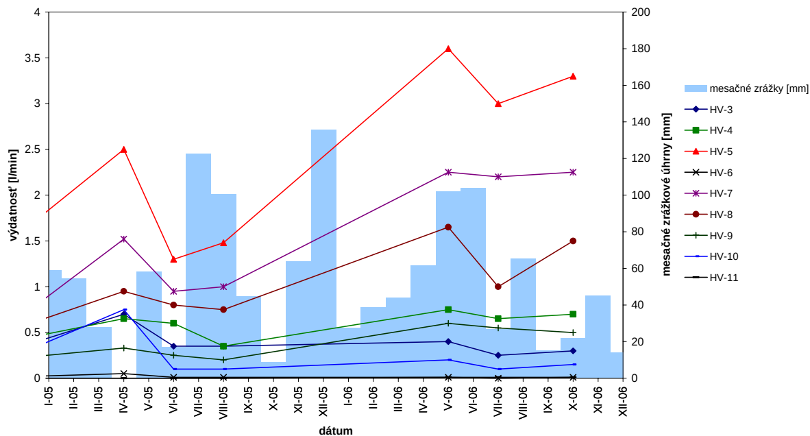
Obr. 2.1.34: Výsledky pozorování hĺbky hladiny podzemnej vody (A) a výdatnosti odvodňovacích zariadení (B) v rokoch 2005 a 2006 na lokalite Ľubietová znázornené spoločne s mesačnými úhrnmi zrážok zo stanice SHMÚ v Ľubietovej
