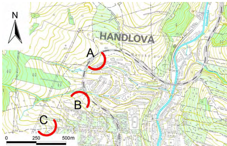
Obr. 2.1.12: Lokalizácia zosuvov nad Morovnianskym sídliskom v Handlovej. A – Morovnianske sídlisko, B – Malá Hôrka, C – Jánošíkova cesta. Značky zosuvov sú umiestnené v čele akumulačných oblastí
