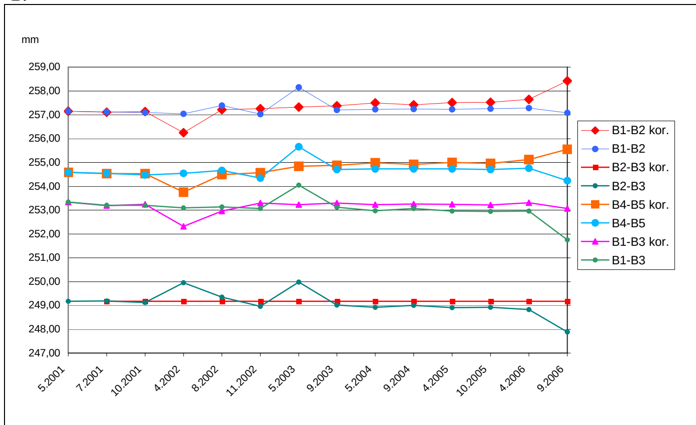
Obr. 2.1.93: Výsledky dlhodobého merania posunu blokov na lokalite Banská Štiavnica: A) meradlom posuvov, B) dilatometrom Somet. Grafy s korekciou nameraných hodnôt zohľadňujú zmeny podmienok a techniky merania (označené príponou kor. – údaje v nich sú upravované v závislosti od hodnoty nameranej vzdialenosti medzi bodmi B2-B3, situovanými na jednom samostatnom horninovom bloku)
