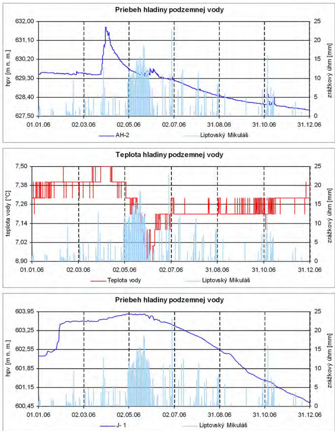
Obr. 2.1.46: Výsledky pozorovania zmien hĺbky hladiny podzemnej vody automatickými hladinomermi, umiestnenými vo vrtoch J-1 a AH-2 na lokalite Okoličné v roku 2006, znázornené spoločne s dennými úhrnmi zrážok zo stanice SHMÚ Liptovský Mikuláš
