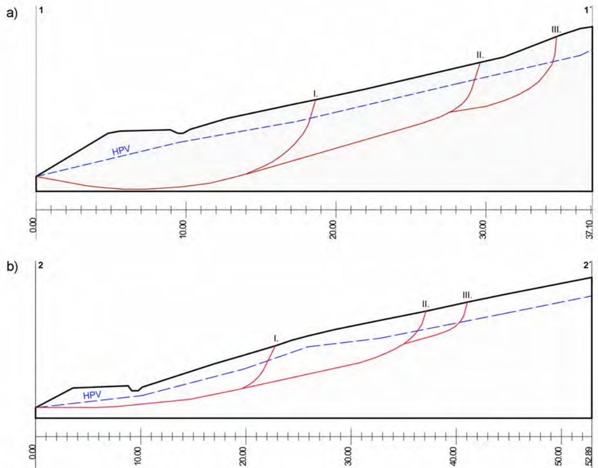
Obr. 2.1.66: Schematické profily pre stabilitné výpočty na lokalite Bojnice. a) profil 1-1', b) profil 2-2', HPV- hladina podzemnej vody, I. až III – výpočtové šmykové plochy
