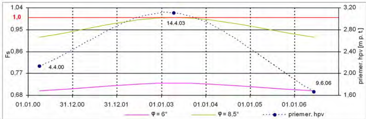
Obr. 2.1.25: Výsledky stabilitných výpočtov v profile 1-1' na lokalite Fintice
