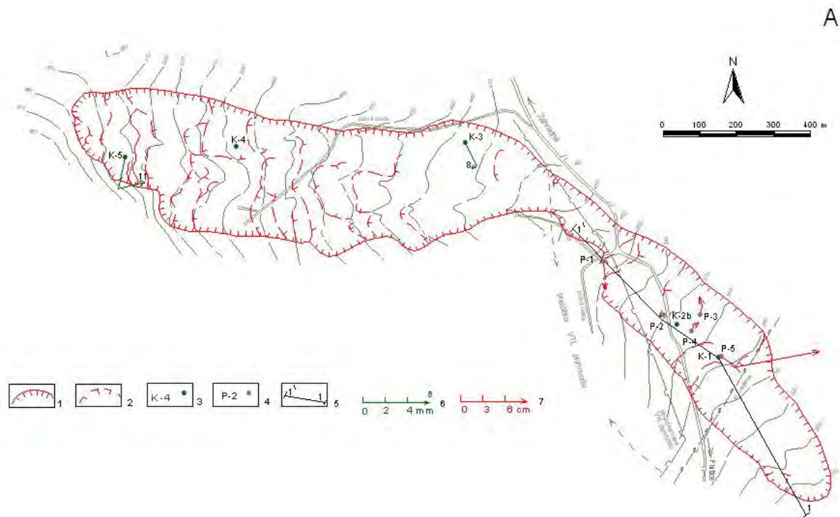
Obr. 2.1.21A: Lokalita Fintice – výsledky geodetických a inklinometrických meraní v rokoch 2005 a 2006. 1 – ohraničenie aktívneho zosuvu, 2 – dielčie zosuvy a zátrhy, 3 – inklinometrické vrty, 4 – geodetické pozorovacie body, 5 – línia profilu pre stabilné výpočty, 6 – mierka vektorov deformácie inklinometrickej pažnice za obdobie IV.04-V.05-VII.06 (číslo označuje hĺbku zaznamenananej deformácie od povrchu terénu v m), 7 – mierka vektorov premiestnení geodetických bodov za obdobie V.04-VII.05-VI.06
