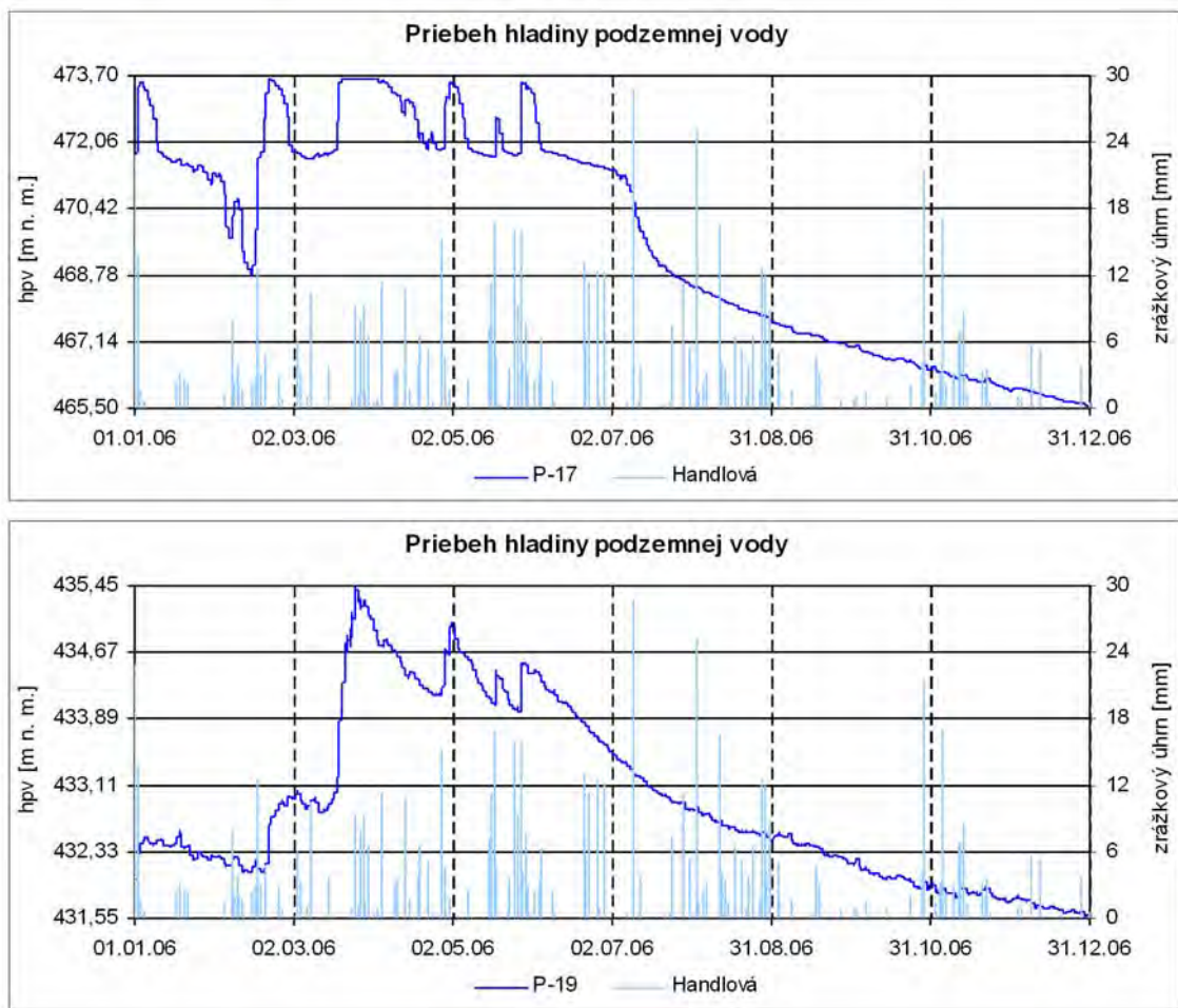
Obr. 2.1.14: Priebeh zmien úrovne hladiny podzemnej vody (hpl), zaznamenaný v roku 2006 automatickými hladinomerami, umiestnenými vo vrtoch P-17 a P-19 na lokalite Handlová – Morovnianske sídlisko spoločne so znázornením denných zrážkových úhrnov zo stanice SHMÚ v Handlovej
