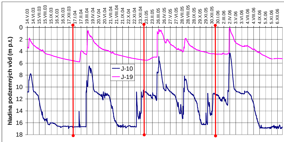
Obr. 2.1.61: Kolísanie hladín podzemných vôd v piezometroch s kontinuálnym meraním
