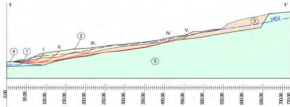
Obr. 2.1.48: Schematický profil 1-1' pre stabilitné výpočty na lokalite Okoličné. 1 – železničný násyp, 2 – zosuvné delúvium, 3 – zvetrané paleogénne ílovce, 4 – aluviálne sedimenty, 5 – podložné paleogénne ílovce a pieskovce, HPV- hladina podzemnej vody, I. až V – výpočtové šmykové plochy
