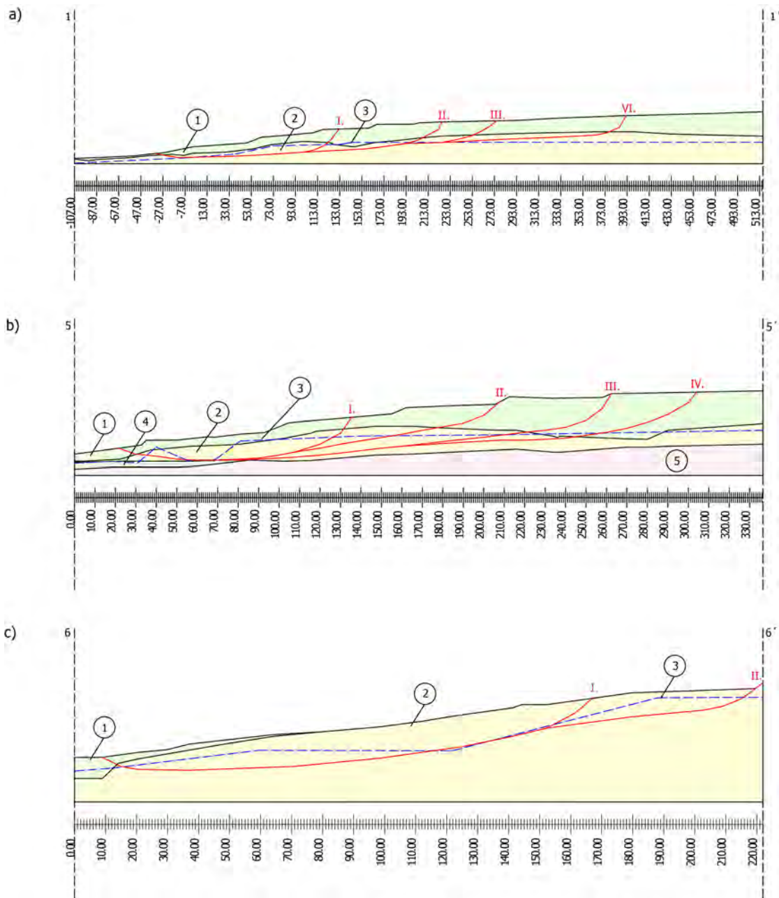
Obr. 2.1.126: Výpočtové modely svahu SN v profiloch: a) 1-1', b) 5-5' a c) 6-6'. I. až IV. označenie šmykových plôch; 1 – navážka, 2 – zosuvné delúvium, 3 – priebeh hladiny podzemnej vody (maximálna úroveň zaznamenaná počas hodnoteného obdobia), 4 – náplavy toku Handlovky, 5 – paleogénne podložie (ílvice, prachovce a slieňovce)
