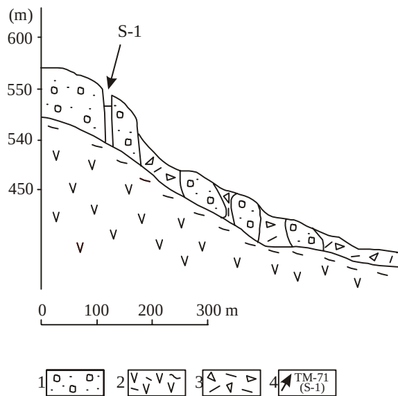
Obr. 2.1.85: Inžinierskogeologický rez svahovou deformáciou na lokalite Sokol s vyznačením osadenia dilatometra S-1. 1 – striedanie andezitov lávových prúdov a autochtónnych pyroklastík, 2 – andezit propylitizovaný a silno zbrekciovatý, 3 – balvanité a úlomkovito-ílovité svahové sedimenty (sute), 4 – lokalizácia dilatometra TM-71 (S-1)
