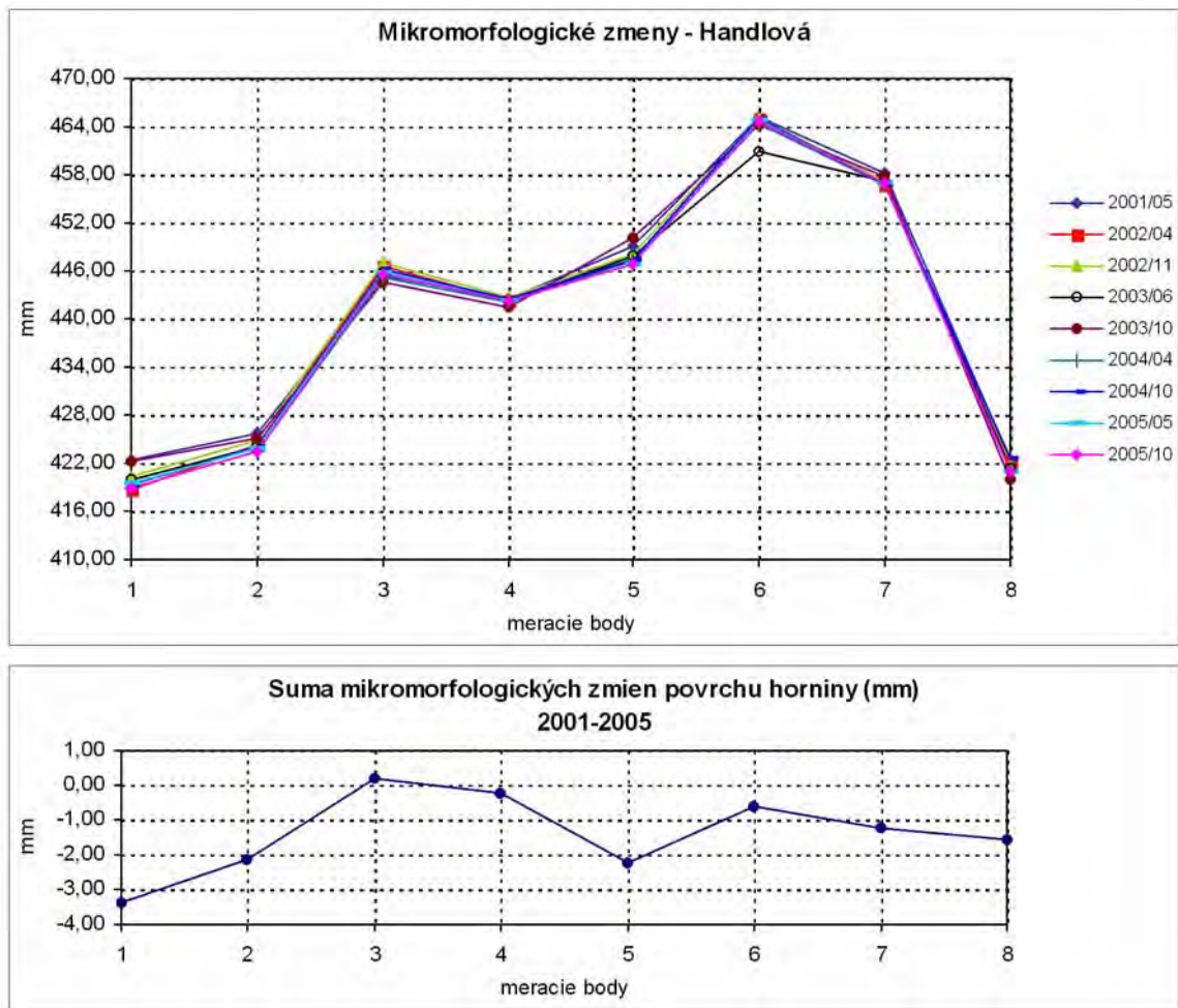
Obr. 2.1.42: Výsledky dlhodobého merania mikromorfologických zmien povrchu odkryvu na lokalite Handlová
