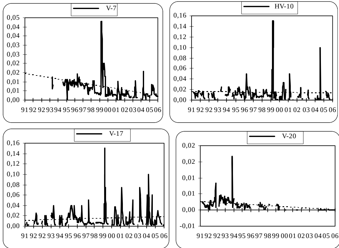
Obr. 2.1.60: Priebeh výdatnosti ( \text{l.s}^{-1} ) vo vybraných horizontálnych odvodňovacích vrtoch a jej trend v období rokov 1991 až 2005
