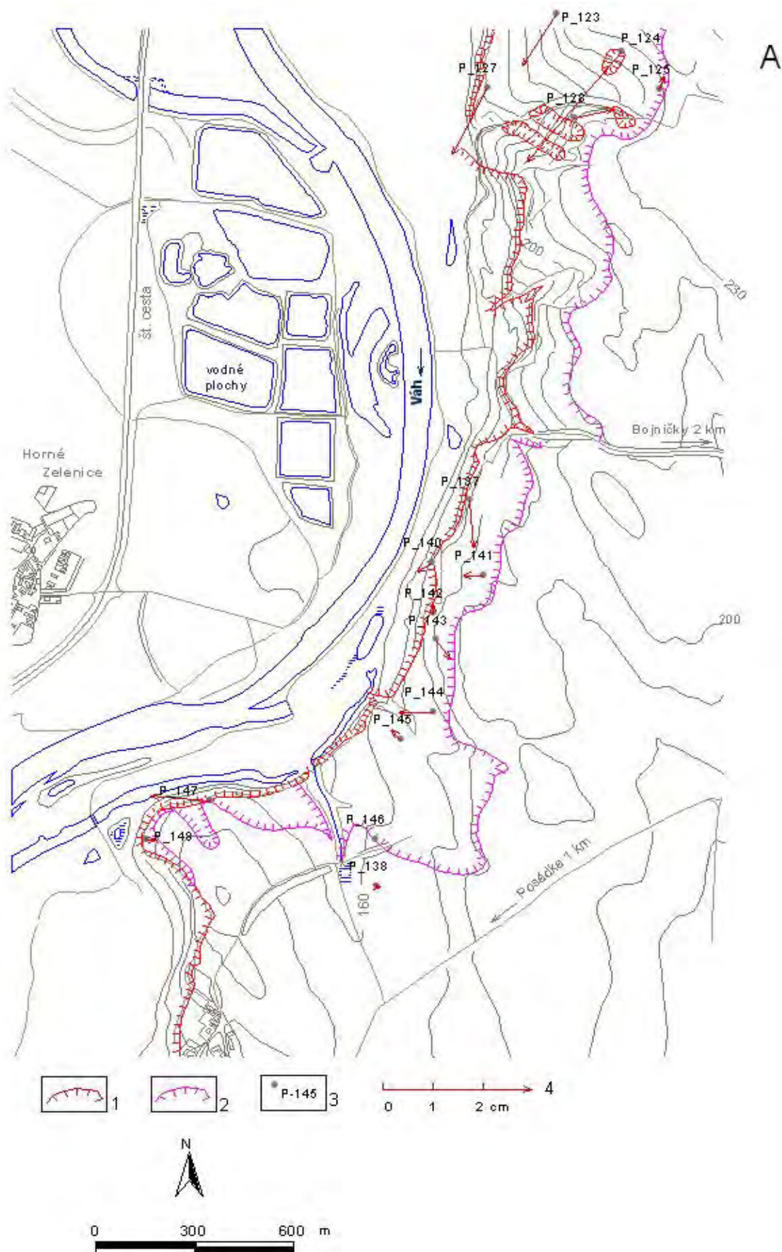
Obr. 2.1.73A: Lokalita Hlohovec-Posádka – výsledky geodetických meraní v rokoch 2004 a 2006. 1 – ohraničenie aktívnych zosuvov, 2 – hranice potenciálnych zosuvov, 3 – geodetické body, 4 – miera vektorov premiestnení geodetických bodov za obdobie VIII.04-IX.06
