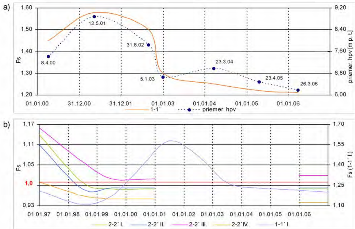
Obr. 2.1.10: Výsledky stabilitných výpočtov v profile 1-1' (a) a 2-2' (b) na lokalite Veľká Čausa
