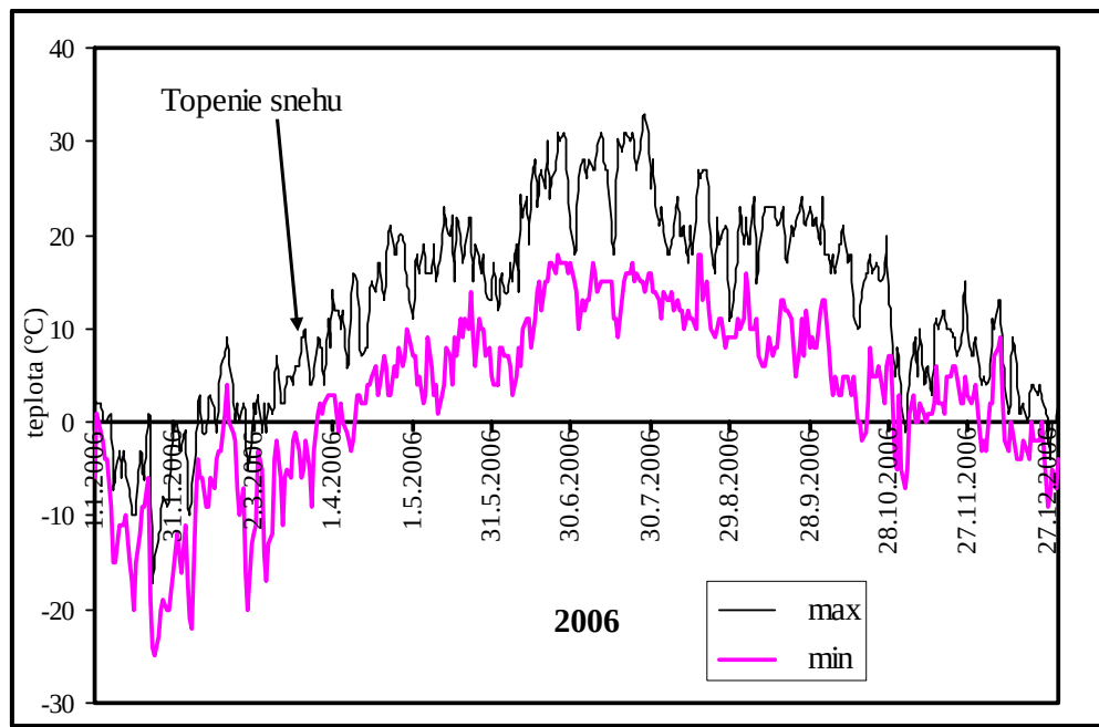
Obr. 2.1.55: Pribeh denných teplôt v roku 2006 (stanica Liptovská Mara)
