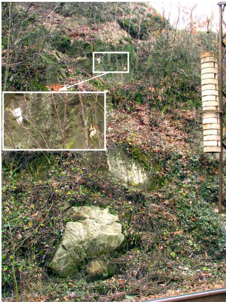
Obr. 2.1.114: Skalná stena železničného zárezu, na ktorej sa vykonáva meranie mikromorfologických zmien povrchu (s detailom umiestnenia meradla morfologických zmien)
