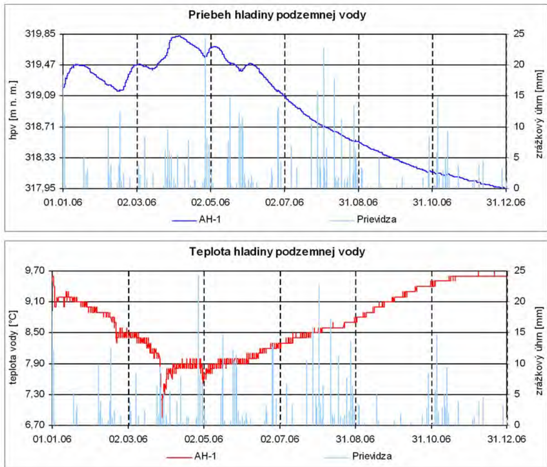
Obr. 2.1.7: Kontinuálny záznam údajov o zmenách hladiny podzemnej vody a teploty vody z dataloggera na lokalite Veľká Čausa
