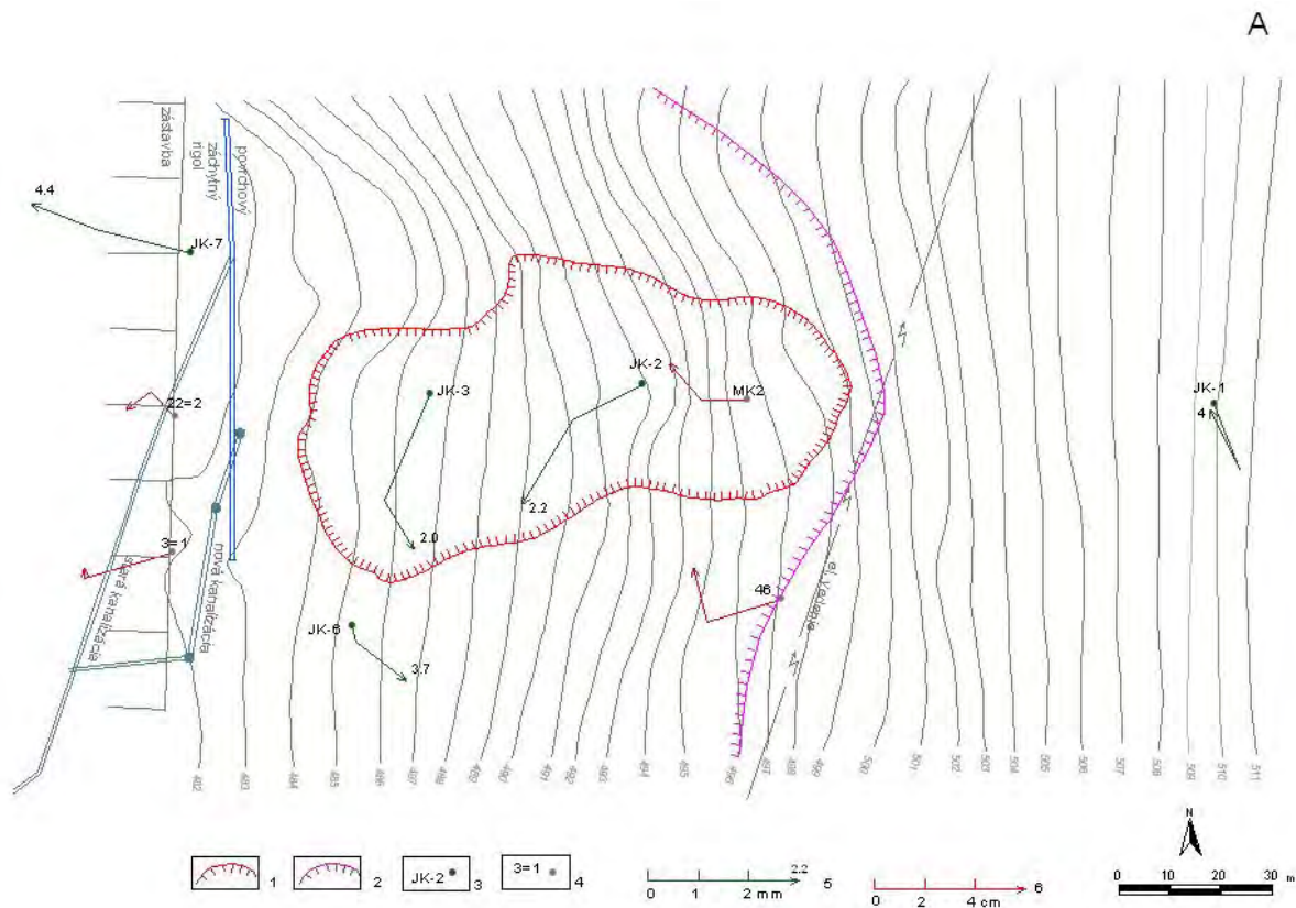
Obr. 2.1.17A: Lokalita Handlová – Kunešovská cesta. Výsledky geodetických a inklinometrických meraní v roku 2006. 1 – ohraničenie aktívneho zosuvu z jesene 1998, 2 – hranica starších svahových deformácií, 3 – inklinometrické (JK) a piezometrické (MK) vrty, 4 – geodetické body, 5 – mierka vektorov inklinometrických deformácií za obdobie V.04-V.05-VII.06 (číslo označuje hĺbku zaznamenatej deformácie od povrchu terénu v m), 6 – mierka vektorov premiestnení geodetických bodov za obdobie V. 05-XI.05-V.06
