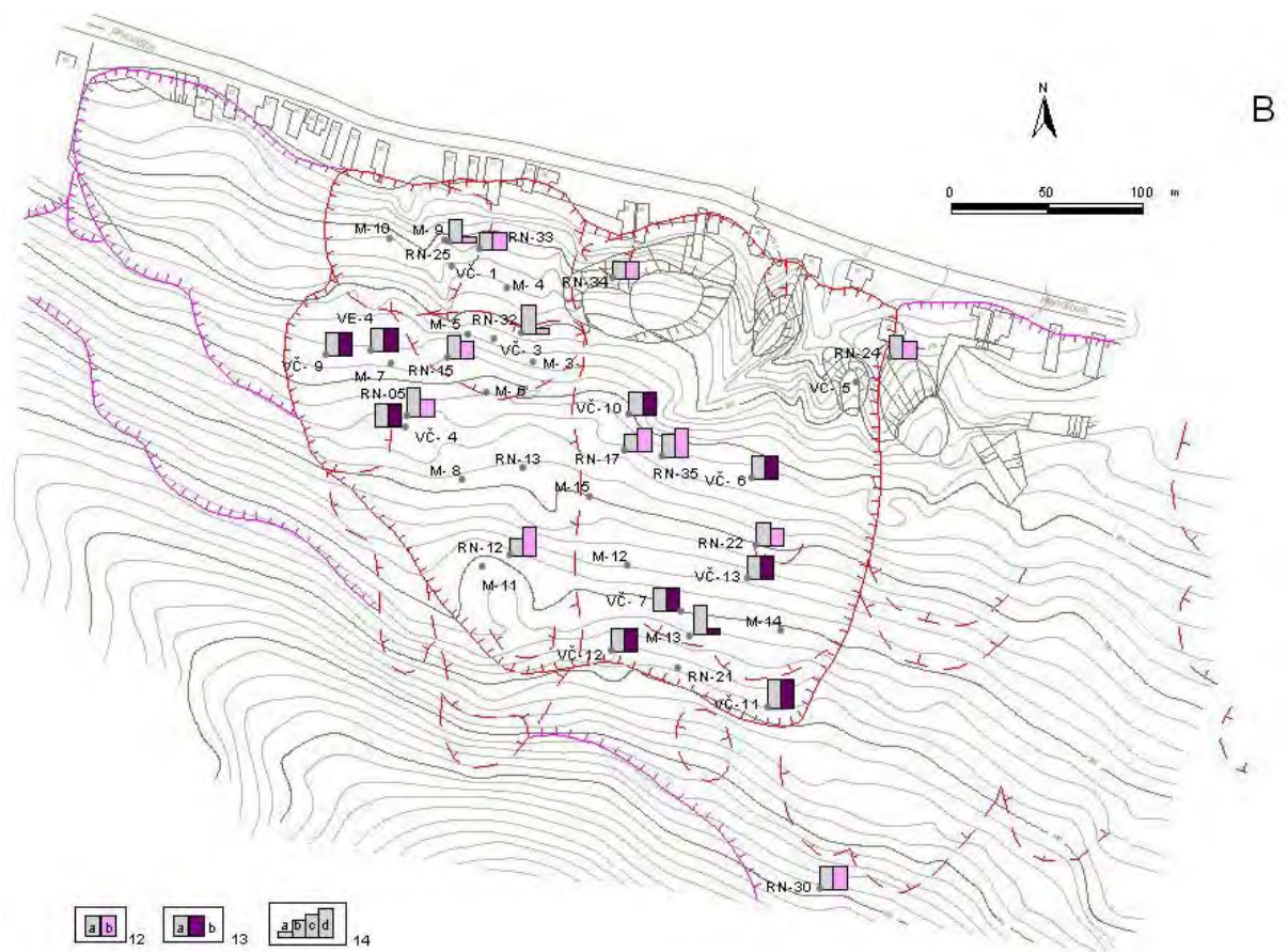
Obr. 2.1.4B: Lokalita Veľká Čausa – výsledky merania povrchového reziduálnych napätí a poľa PEE. 12 – povrchové reziduálne napätia v rokoch: a – 2005, b – 2006, 13 – aktivita poľa PEE v rokoch: a – 2005, b – 2006, 14 – hodnotenie napätostného poľa podľa kritérií, zhrnutých v tab. 2.1.4: a – nemerané, b – nízky stav povrchových reziduálnych napätí, resp. nízka aktivita poľa PEE (stupeň 1), c – stredný stav napätí, resp. stredná aktivita poľa PEE (stupeň 2), d – vysoký stav napätí, resp. vysoká aktivita poľa PEE (stupeň 3)
