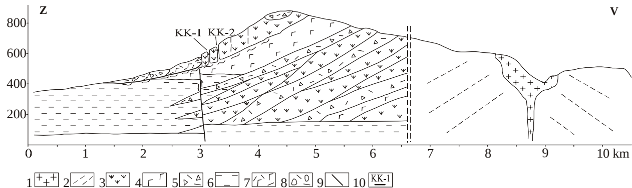
Obr. 2.1.88: Inžinierskogeologický rez stratovulkánom Strechový vrch so svahovou deformáciou a vyznačením osadenia dilatometrov KK-1 a KK-2 (lokalita Košický Klečenov). 1 – itrúzia dioritového porfyritu, 2 – striedanie lávových prúdov a pyroklastík, 3 – andezitový lávový prúd, 4 – pyroklastiká (nečlenené), 5 – redeponované andezitové pyroklastiká, 6 – neogénne íly, 7 –redeponované andezitové tufy, 8 – ílovito-úlomkovitá suť, 9 – aktívny zlom, 10 –lokalizácia dilatometrov KK-1 a KK-2
