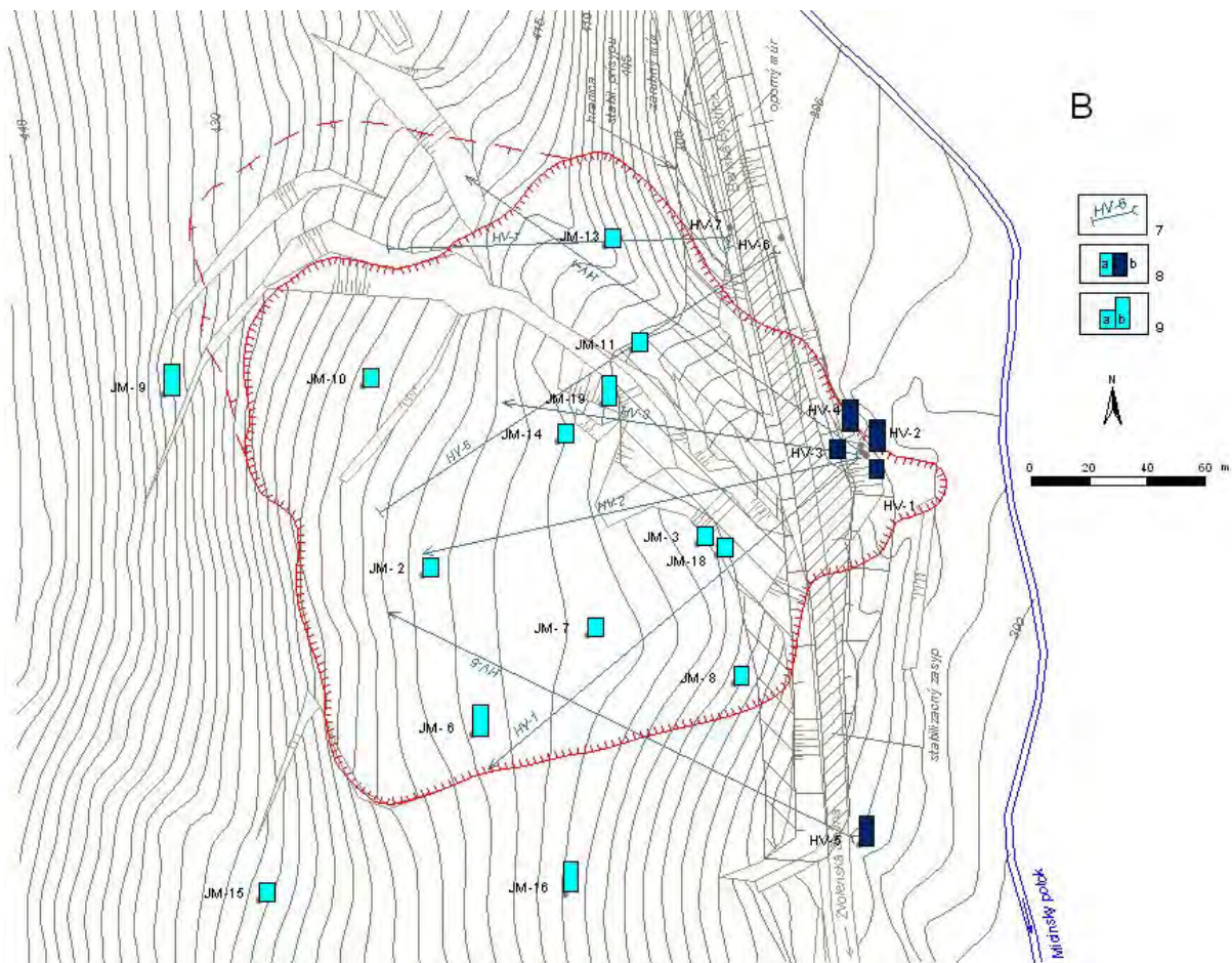
Obr. 2.1.27B: Lokalita Dolná Mičiná – výsledky režimových pozorovaní. 7 – horizontálne odvodňovacie vrty, 8 – režimové pozorovania v roku 2006: a – zmeny hĺbky hladiny podzemnej vody, b – výdatnosť odvodňovacích zariadení, 9 – hodnotenie režimových pozorovaní podľa kritérií, zhrnutých v tab. 2.1.5: a – stav priaznivý (stupeň 1) vo vertikálnych vrtoch, resp. priem. výdatnosť do 1 \text{ l.min}^{-1} v horizontálnych vrtoch, b – stav nepriaznivý (stupeň 3), resp. výdatnosť nad 3 \text{ l.min}^{-1}
