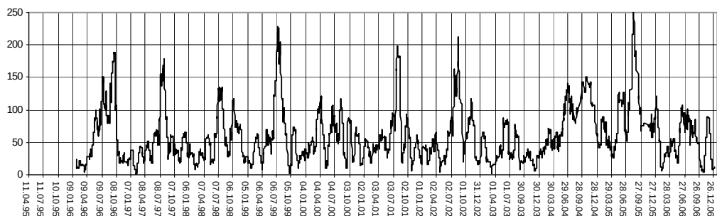
Obr. 2.1.47: Výsledky režimových pozorovaní na lokalite Okoličné
