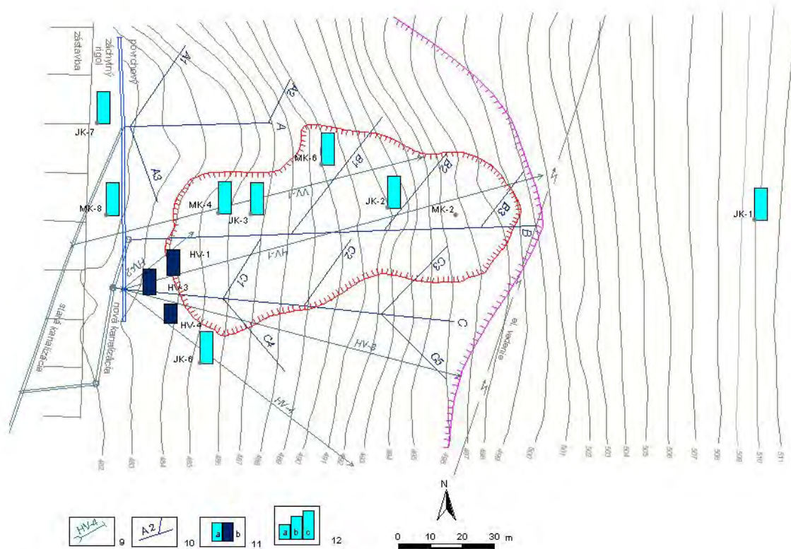
Obr. 2.1.17C – Lokalita Handlová – Kunešovská cesta. Výsledky režimových pozorovaní. 9 – horizontálne odvodňovacie vrty, 10 – stabilizačno - odvodňovacie rebrá (A, B, C) a bočné drenážne rebrá (A1, A2 atď.), 11 – režimové pozorovania v roku 2006: a – zmeny hĺbky hladiny podzemnej vody, b – výdatnosť odvodňovacích zariadení, 12 – hodnotenie režimových pozorovaní za rok 2006 podľa kritérií, zhrnutých v tab. 2.1.5: a – stav priaznivý (stupeň 1) vo vertikálnych vrtoch, resp. priemerná výdatnosť do 1 l.min -1 v horizontálnych vrtoch, b – náznaky nepriaznivého stavu (stupeň 2), resp. priemerná výdatnosť 1 až 3 l.min -1 , c - stav nepriaznivý (stupeň 3), resp. priemerná výdatnosť nad 3 l.min -1
