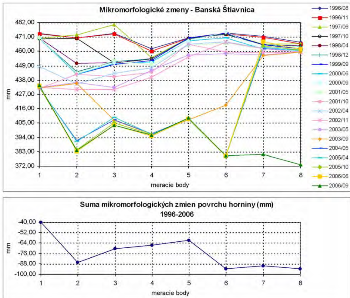
Obr. 2.1.94: Výsledky dlhodobého merania mikromorfologických zmien povrchu skalného svahu na lokalite Banská Štiavnica
