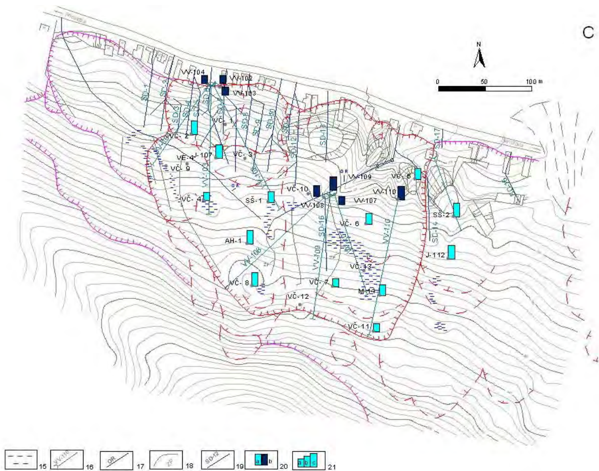
Obr. 2.1.4C: Lokalita Veľká Čausa – výsledky režimových pozorovaní. 15 – zamokrené územia, 16 – horizontálne odvodňovacie vrty, 17 – dláždené odvodňovacie rigoly, 18 – zemné odvodňovacie priekopy, 19 – sanačné drenážne a stabilizačné rebrá, 20 – režimové pozorovania v roku 2006: a – zmeny hĺbky hladiny podzemnej vody, b – výdatnosť odvodňovacích zariadení, 21 – hodnotenie režimových pozorovaní za rok 2006 podľa kritérií, zhrnutých v tab. 2.1.5: a – stav priaznivý (stupeň 1) vo vertikálnych vrtoch, resp. priem. výdatnosť do 1 \text{ l.min}^{-1} v horizontálnych vrtoch, b – náznaky nepriaznivého stavu (stupeň 2), resp. priemerná výdatnosť 1 až 3 \text{ l.min}^{-1} , c – stav nepriaznivý (stupeň 3), resp. priemerná výdatnosť nad 3 \text{ l.min}^{-1}
