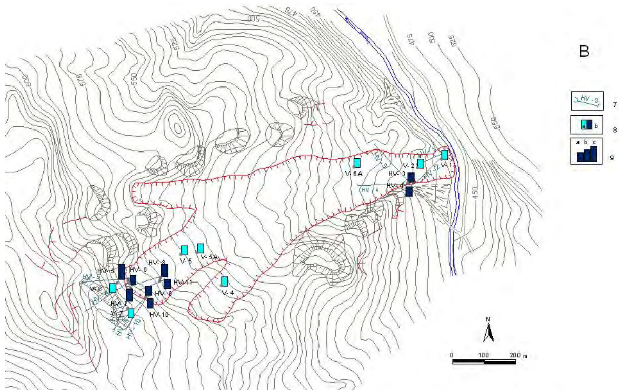
Obr. 2.1.32B: Lokalita Ľubietová – výsledky režimových pozorovaní. 7 – odvodňovacie horizontálne vrty, 8 – režimové pozorovania v roku 2006: a – zmeny hĺbky hladiny podzemnej vody, b – výdatnosť odvodňovacích zariadení, 9 – hodnotenie režimových pozorovaní podľa kritérií, zhrnutých v tab. 2.1.5: a – stav priaznivý (stupeň 1) vo vertikálnych vrtoch, resp. priem. výdatnosť do 1 \text{ l.min}^{-1} v horizontálnych vrtoch, b – výdatnosť 1 až 3 \text{ l.min}^{-1} , c – výdatnosť nad 3 \text{ l.min}^{-1}
