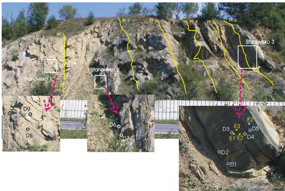
Obr. 2.1.96: Rozmiestnenie pozorovaných profilov a bodov na monitorovanom úseku zárezu cesty severne od obce Demjata. PF1 až PF6 – profily pre stereofotogrametrické merania, E1 až E3, E2' – pozorovacie body pre merania dilatometrom Somet, D1 až D9 – pozorovacie body pre merania meradlom posuvov. Stanovisko s bodmi E4 a E5 sa nachádza na protiľahlom svahu zárezu
