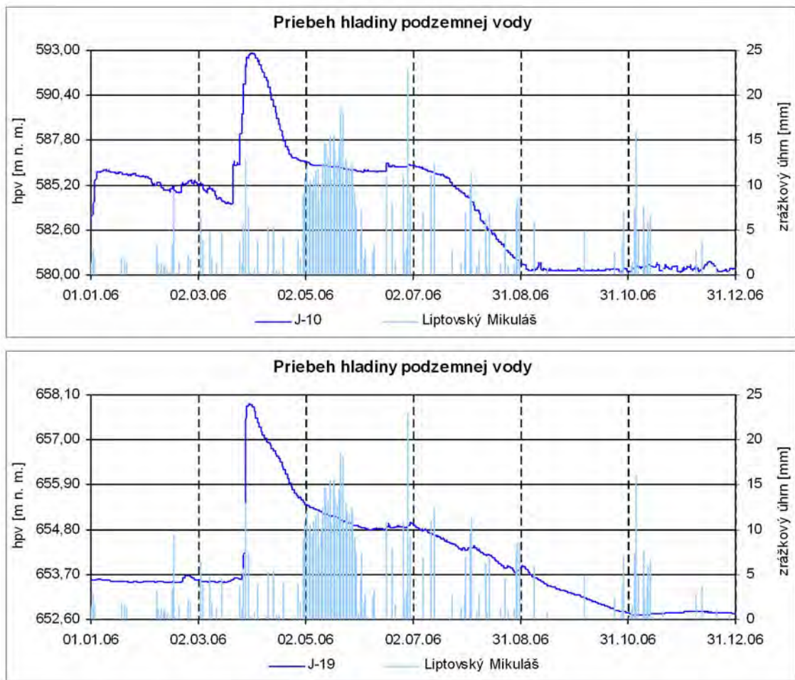
Obr. 2.1.56: Priebehy zmien hladiny podzemnej vody v automatických hladinomeroch umiestnených vo vrtoch J-10 a J-19 na lokalite Liptovská Mara v roku 2006, znázornené spoločne s dennými úhrnmi zrážok zo stanice SHMÚ Liptovský Mikuláš
