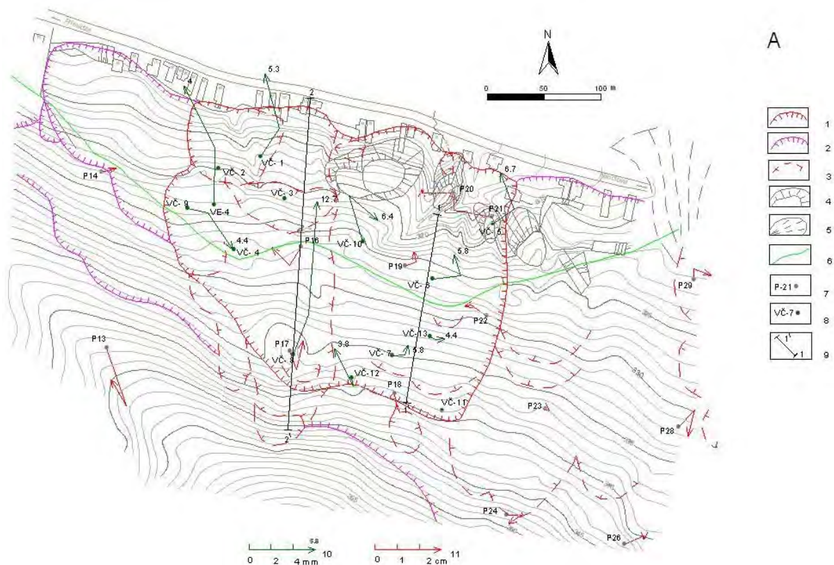
Obr. 2.1.4A: Lokalita Veľká Čausa – výsledky geodetických a inklinometrických meraní v rokoch 2005 a 2006. 1 – ohraňenie aktívnych zosuvov, 2 – ohraňenie potenciálnych zosuvov, 3 – lokálne zosuvy a zátrhy, 4 – premiestnené bloky vulkanických hornín, 5 – prolúviálny kužeľ, 6 – interpretovaný okraj štrkovej terasovej akumulácie, 7 – geodetické body, 8 – inklinometrické vrty, 9 – línie profilov pre stabilné výpočty, 10 – mierka vektorov inklinometrických deformácií za obdobie IV.04-V.05-IX.06 (číslo označuje hĺbku zaznamenananej deformácie od povrchu terénu v m) 11 – mierka vektorov premiestnení geodetických bodov za obdobie V.04-V.05-VI.06
