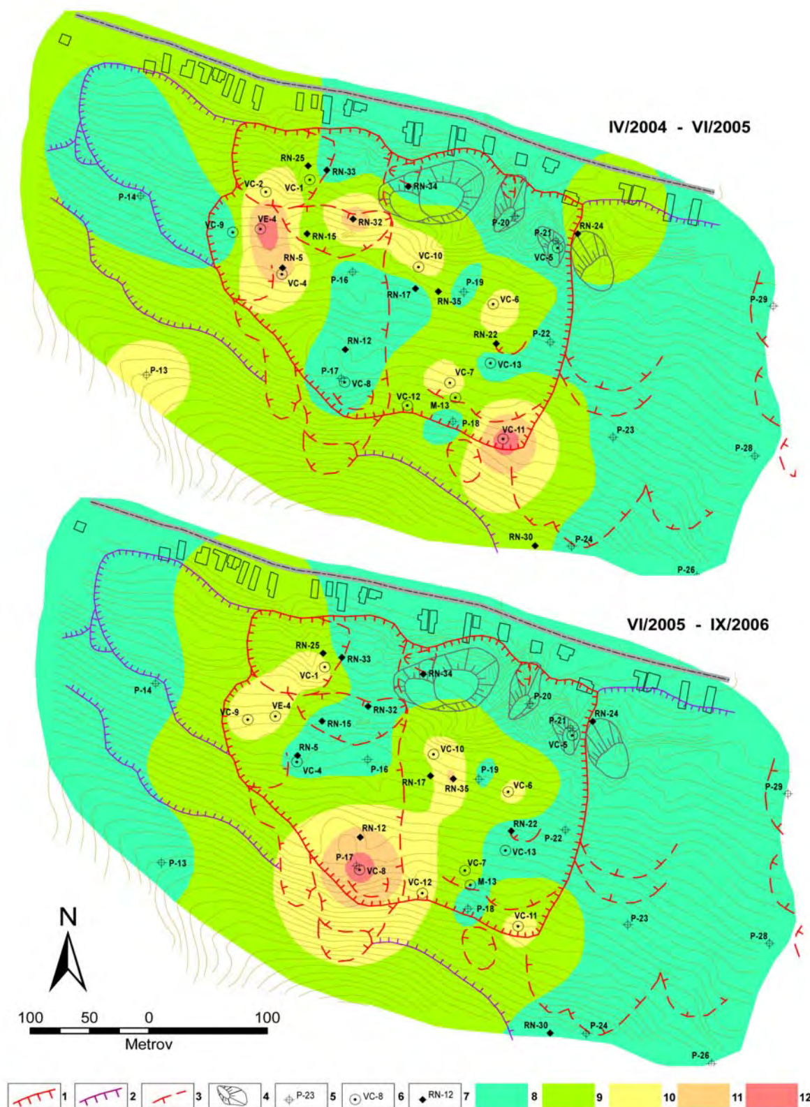
Obr. 2.1.11: Komplexné spracovanie výsledkov monitorovacích meraní (zhodnotených podľa kritérií tab. 2.1.4) na lokalite Veľká Čausa za roky 2004 až 2006. 1 – ohraničenie aktívnych foriem zosuvov, 2 – ohraničenie potenciálnych a stabilizovaných zosuvov, 3 – lokálne zosuvy a zátrhy, 4 – premiestnené bloky vulkanických hornín, 5 – body geodetickej siete, 6 – inklinometrické vrty, 7 – miesta merania povrchových reziduálnych napätí, 8 – stabilný stav častí územia, 9 – náznaky pohybovej aktivity zosuvu, 10 – mierne aktívny stav, 11 – aktívny stav, 12 – vysoko aktívny stav
