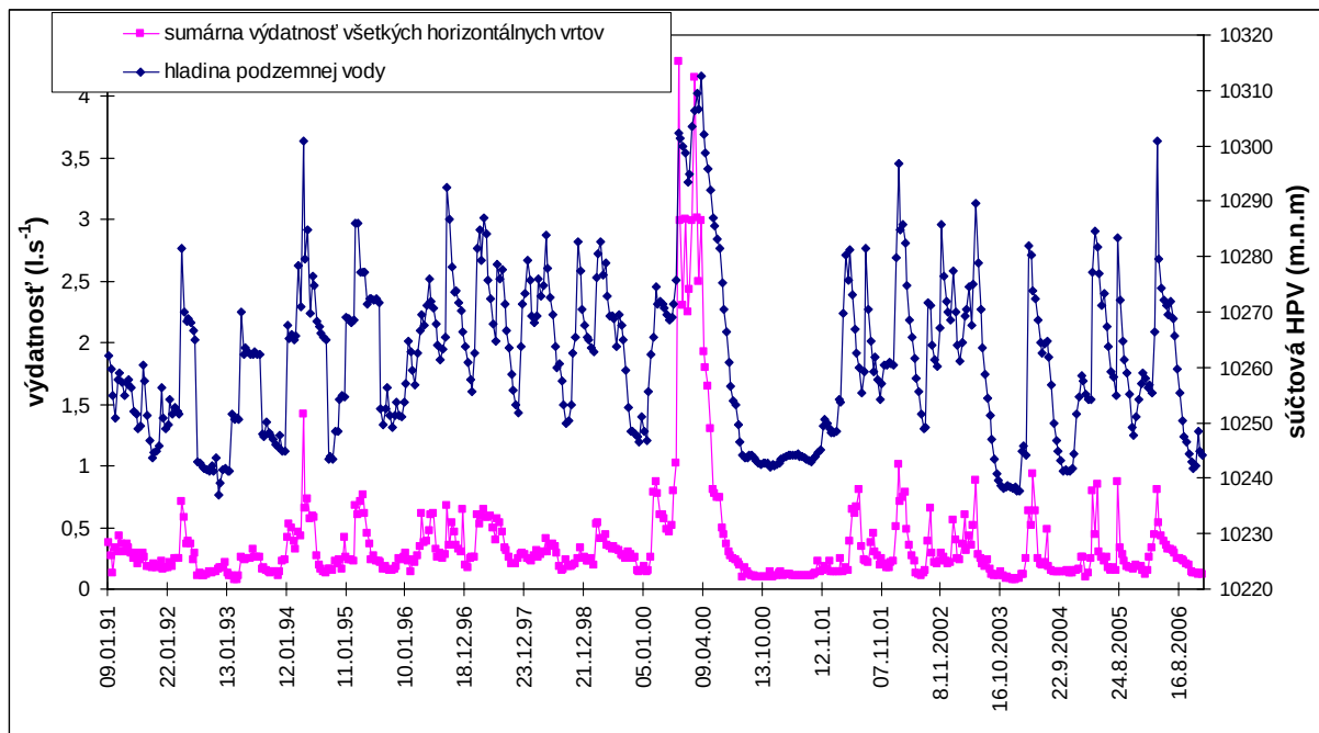
Obr. 2.1.59: Závislosť medzi stavom hladín podzemných vôd na Veľkomarskom zosuve (súčet hladín) a sumárnou výdatnosťou horizontálnych odvodňovacích vrtov
