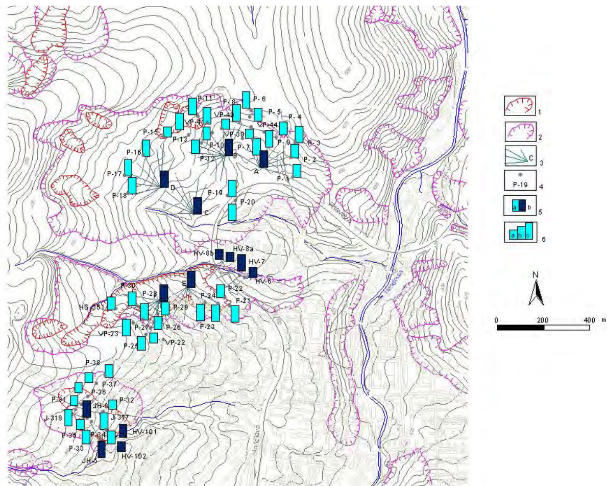
Obr. 2.1.13: Lokalita Handlová – Morovnianske sídlisko – situácia monitorovacích objektov a semikvantitatívne hodnotenie výsledkov režimových pozorovaní v roku 2006. 1 – ohraničenie aktívnych zosuvov, 2 – potenciálne zosuvy, 3 – odvodňovacie jamy s vejármi horizontálnych vrto, 4 – pozorovacie vrty, 5 – režimové pozorovania v roku 2006: a – zmeny úrovne hladiny podzemnej vody, b – výdatnosť odvodňovacích zariadení, 6 – hodnotenie režimových pozorovaní za rok 2006 podľa kritérií, zhrnutých v tab. 2.1.5: a – stav priaznivý (stupeň 1) vo vertikálnych vrtoch, resp. priemerná výdatnosť do 1 \text{ l.min}^{-1} v horizontálnych vrtoch, b – náznaky nepriaznivého stavu (stupeň 2), resp. priem. výdatnosť 1 až 3 \text{ l.min}^{-1} , c – stav nepriaznivý (stupeň 3), resp. priem. výdatnosť nad 3 \text{ l.min}^{-1}
