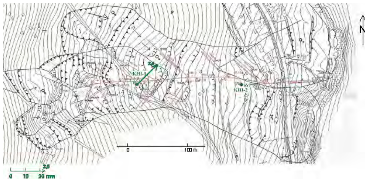
Obr. 2.1.70: Monitorovaný zosuv s vyznačením odvodňovacieho systému, pozostávajúceho z hlavného a 10 bočných drénov (zobrazené červenou farbou) a monitorovaného vrtu KHI-1 s vektorom deformácie inklinometrickej pažnice za obdobie 12. 2004 až 04. 2006 (znázornené zelenou farbou)
