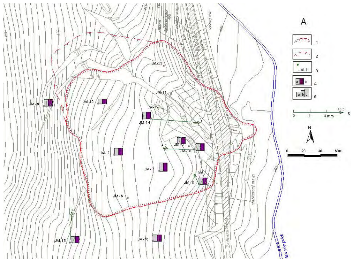
Obr. 2.1.27A: Lokalita Dolná Mičiná – výsledky inklinometrických meraní a merania poľa PEE. 1 – ohraničenie aktívneho zosuvu z roku 1994, 2 – dielčí zosuv, 3 – inklinometrické vrty, 4 – aktivita poľa PEE v rokoch: a – 2005, b – 2006, 5 – hodnotenie poľa PEE podľa kritérií, zhrnutých v tab. 2.1.4: a – nízka aktivita poľa PEE (stupeň 1), b – stredná aktivita poľa PEE (stupeň 2), c – vysoká aktivita poľa PEE (stupeň 3), 6 – mierka vektorov deformácie inklinometrickej pažnice za obdobie IV.04-X.06 (číslo označuje hĺbku zaznamenanaj deformácie od povrchu terénu v m)
