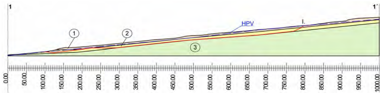
Obr. 2.1.24: Schematický profil 1-1' pre stabilitné výpočty na lokalite Fintice. 1 – deluviálna suť, 2 – zosuvné prevažne hlinité delúvium, 3 – paleogénne ílovce, HPV- hladina podzemnej vody, I. – výpočtová šmyková plocha
