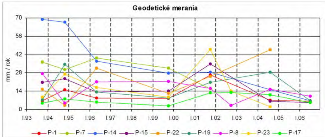
Obr. 2.1.33: Dlhodobé zmeny hodnôt geodetických meraní na lokalite Ľubietová
