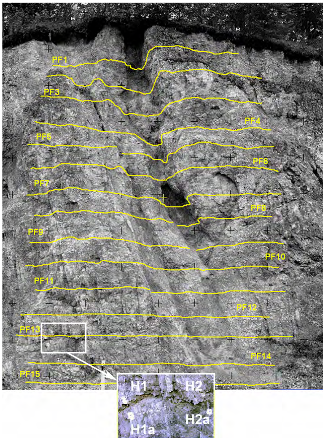
Obr. 2.1.107: Rozmiestnenie pozorovaných profilov a bodov na monitorovanom úseku zárezu cesty medzi Dolným Harmancom a Čremošným. PF1 až PF15 – profily pre stereofotogrametrické merania, H1, H1'. H2, H2' – pozorovacie body pre merania dilatometrom Somet
