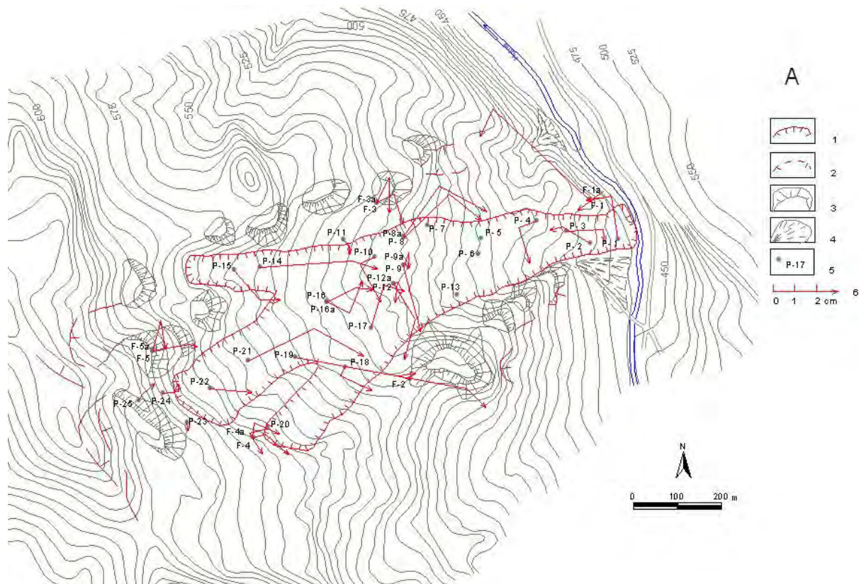
Obr. 2.1.32A: Lokalita Ľubietová – výsledky geodetických meraní v rokoch 2004 a 2006. 1 – ohraničenie aktívneho zosuvu, 2 – dielčie zosuvy a zátrhy, 3 – bloky a blokové polia vulkanických hornín, 4 – náplavové kužele, 5 – geodetické body, 6 – mierka vektorov premiestnení geodetických bodov za obdobie X.01-VIII.04-VIII.06
