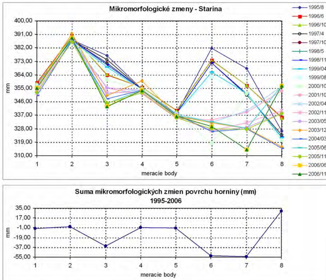
Obr. 2.1.101: Výsledky dlhodobého merania mikromorfologických zmien povrchu odkryvu na lokalite Starina
