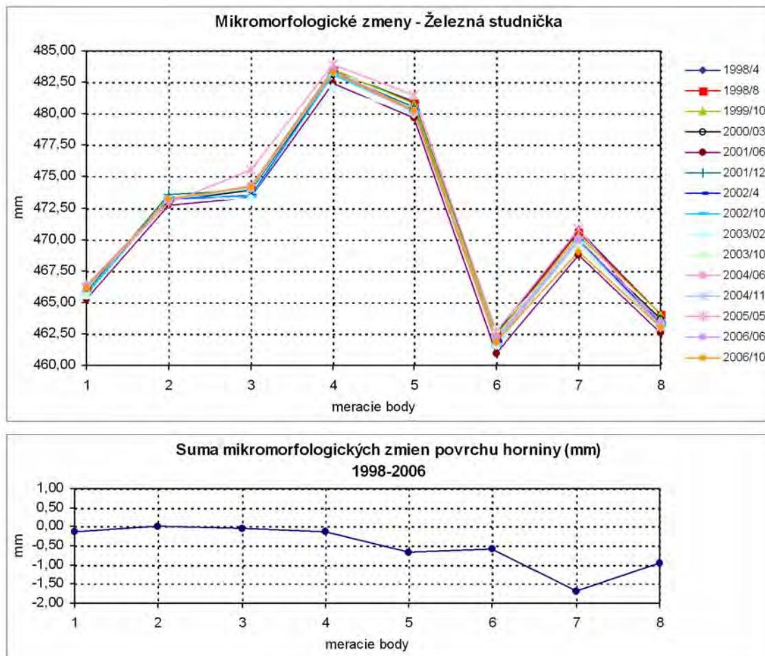
Obr. 2.1.115: Výsledky dlhodobého merania mikromorfologických zmien povrchu odkryvu na lokalite Bratislava-Železná studnička
