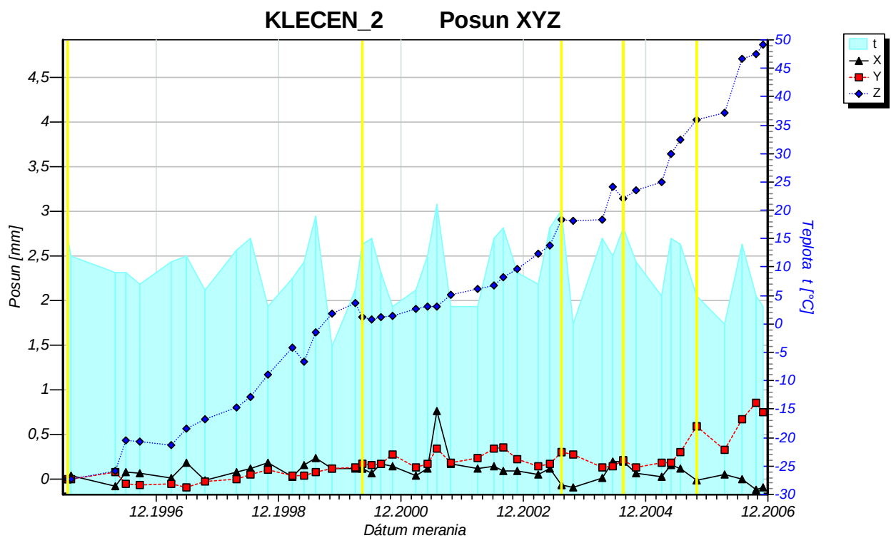
Obr. 2.1.89: Výsledky dlhodobého merania posunov horninových blokov dilatometrami TM-71 na lokalite Košícký Klečenov
