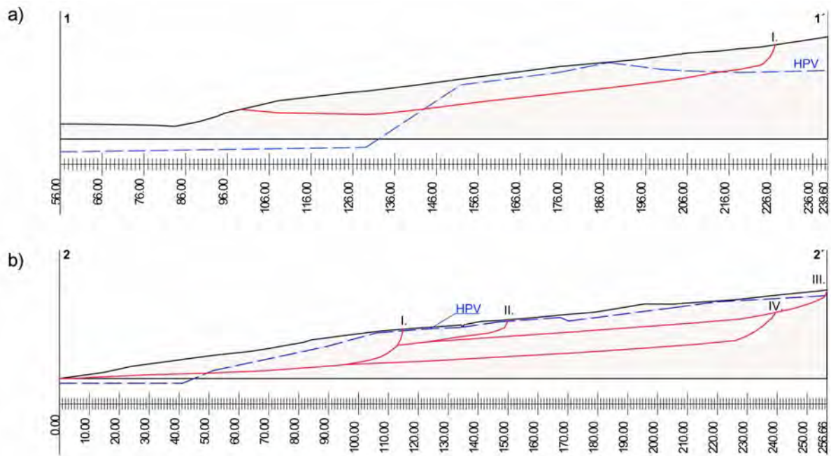
Obr. 2.1.9: Schematické profily pre stabilitné výpočty na lokalite Veľká Čausa. a – profil 1-1', b – profil 2-2' (obr. 2.1.4A), HPV – uvažovaná hladina podzemnej vody, I.. až IV. – predpokladané šmykové plochy
