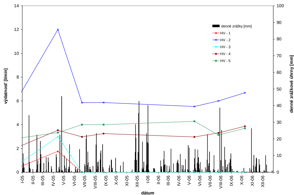
Obr. 2.1.29: Výsledky pozorování hĺbky hladiny podzemnej vody (A) a výdatnosti odvodňovacích zariadení (B) v rokoch 2005 a 2006 znázornené spoločne s dennými úhrnmi zrážok zo stanice SHMÚ v Banskej Bystrici
