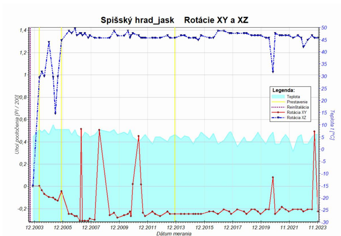
Obr. 17b Graf rotácií travertínových blokov v horizontálnej (XY) a vertikálnej (XZ) rovine zostavený na základe údajov z dilatometra TM-71-jaskyňa za monitorovacie obdobie 2003 – 2023.
