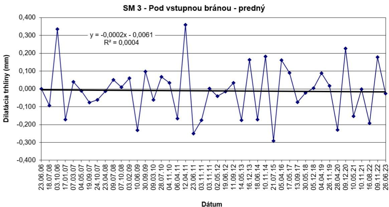
Obr. 26 Výsledky meraní pohybu blokov dilatometrom SM 3 na Trenčianskom hrade v rokoch 2006 – 2023.
