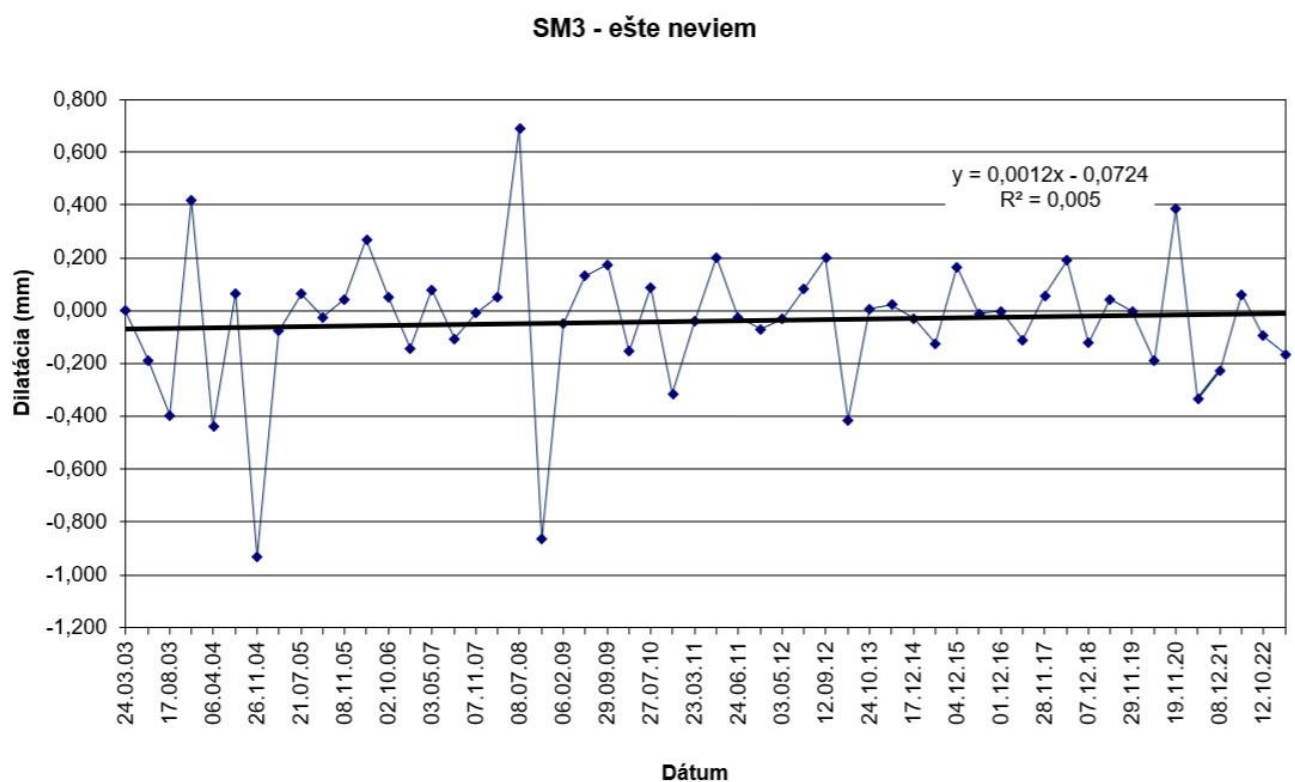
Obr. 34 Výsledky meraní pohybu blokov dilatometrom SM 3 na Pajštúnskom hrade v rokoch 2003 – 2023.
