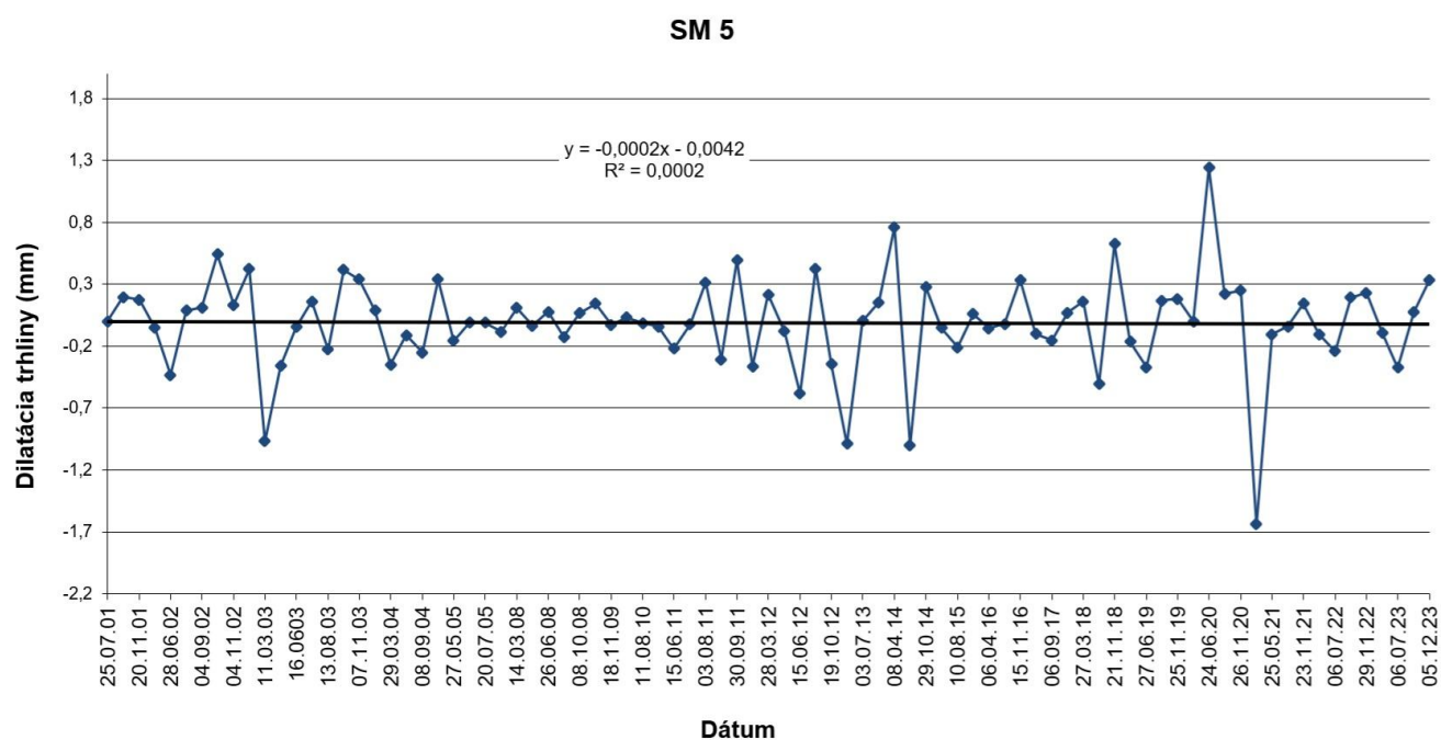
Obr.19 Výsledky meraní pohybu blokov dilatometrom SM 5 na lokalite Spišský hrad za monitorovacie obdobie 2001 – 2023
