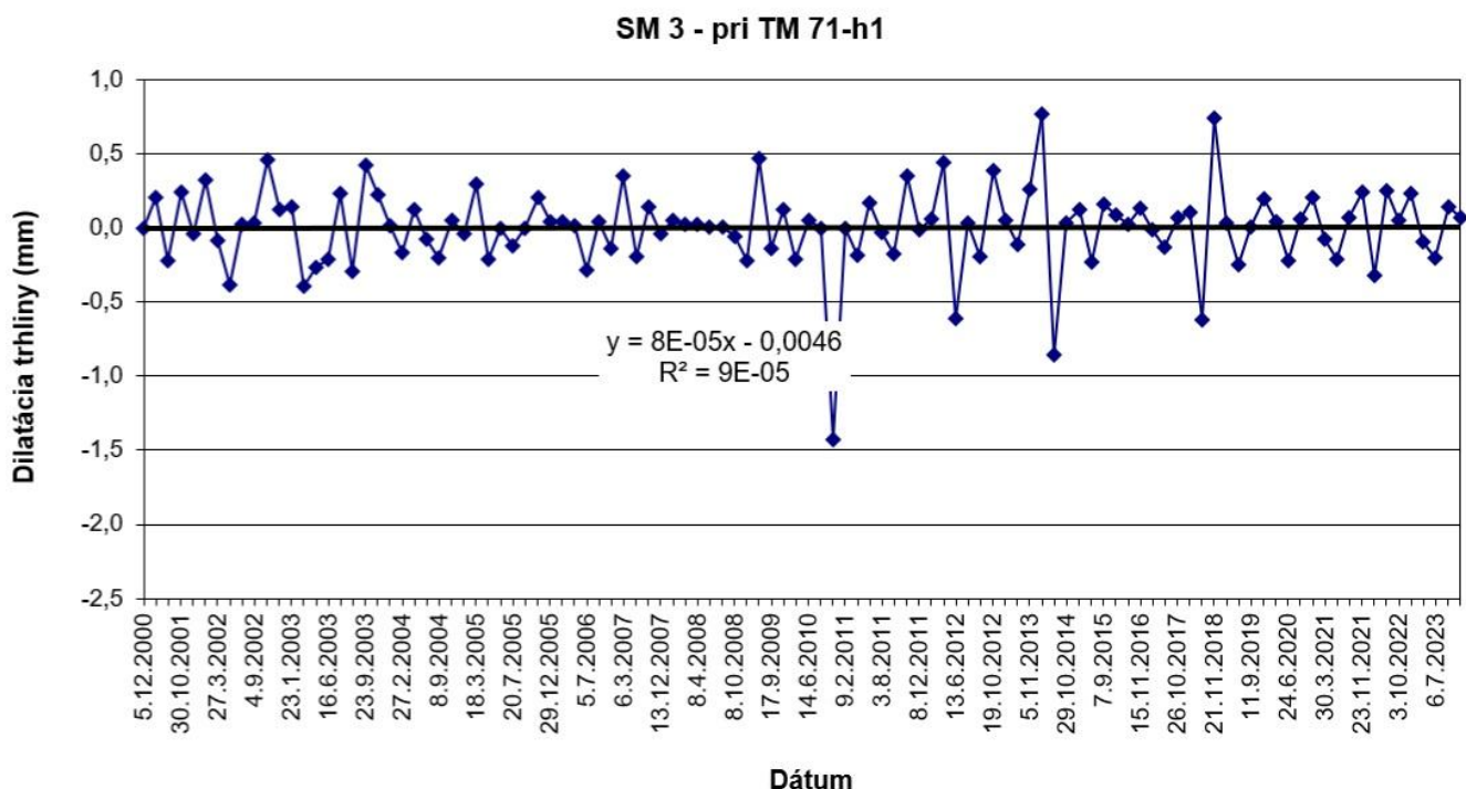
Obr. 7 Výsledky meraní pohybu blokov dilatometrom SM 3 na Spišskom hrade v období rokov 2000 – 2023
