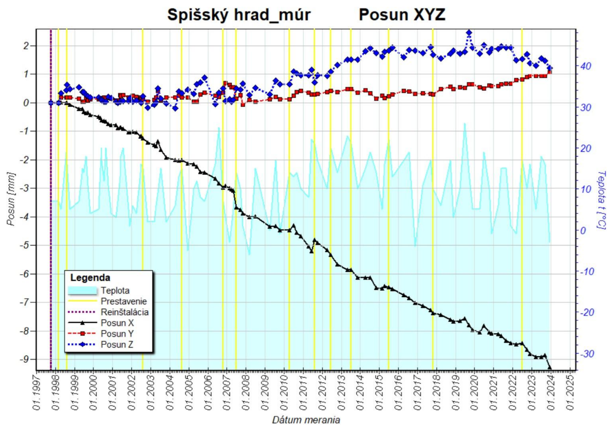
Obr. 14a Graf posunu travertínových blokov pozdĺž osí x, y, z zostavený na základe údajov z dilatometra TM-71-h2 (múr) za monitorovacie obdobie 1997 – 2023.
