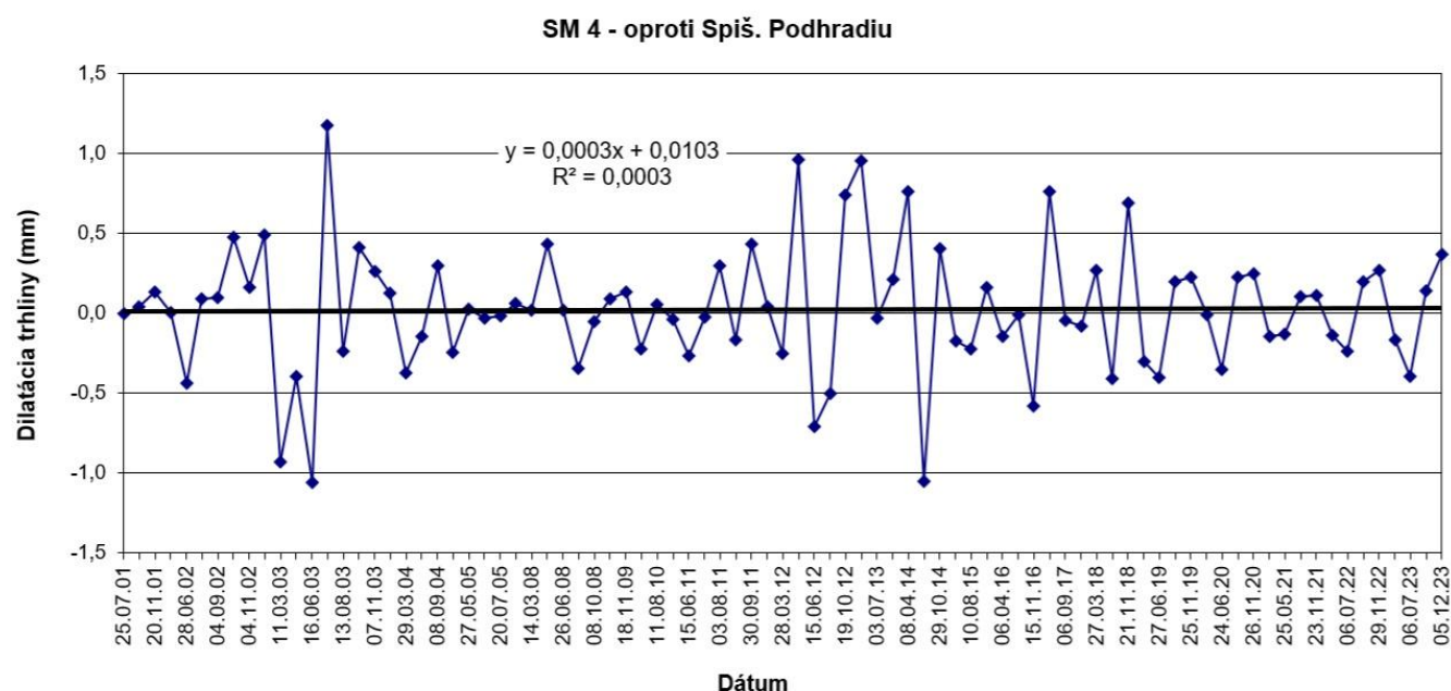
Obr. 18: Výsledky meraní pohybu blokov dilatometrom SM 4 na lokalite Spišský hrad za monitorovacie obdobie 2001 – 2023
