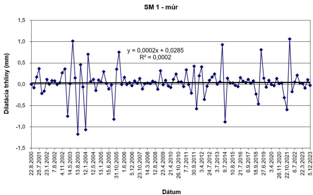
Obr.15 Výsledky meraní pohybu blokov dilatometrom SM 1 na lokalite Spišský hrad v rokoch 2000 – 2023
