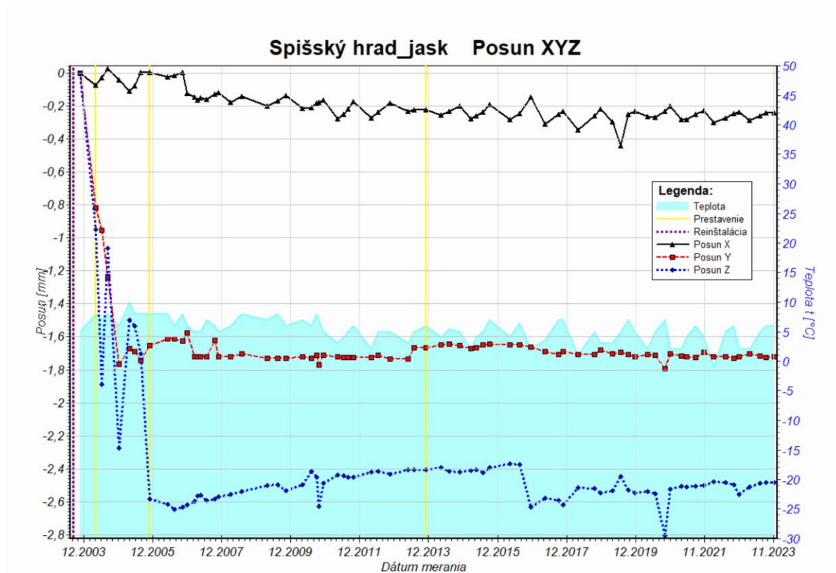
Obr. 17a Graf posunu travertínových blokov pozdĺž osí x, y a z zostavený na základe údajov z dilatometra TM- 71-jaskyňa za monitorovacie obdobie 2003 – 2023.
