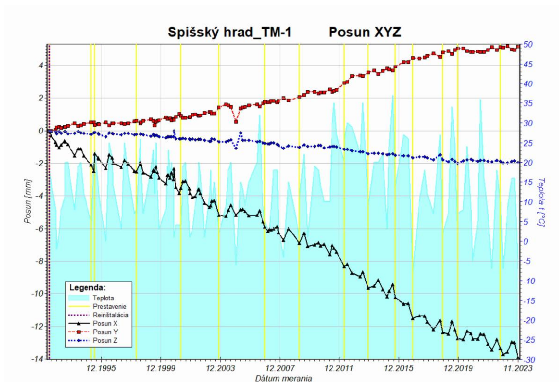
Obr. 8a Graf posunu travertínových blokov pozdĺž osí x, y a z zostavený na základe údajov z dilatometra TM-71-1 za monitorovacie obdobie 1992 – 2023.
