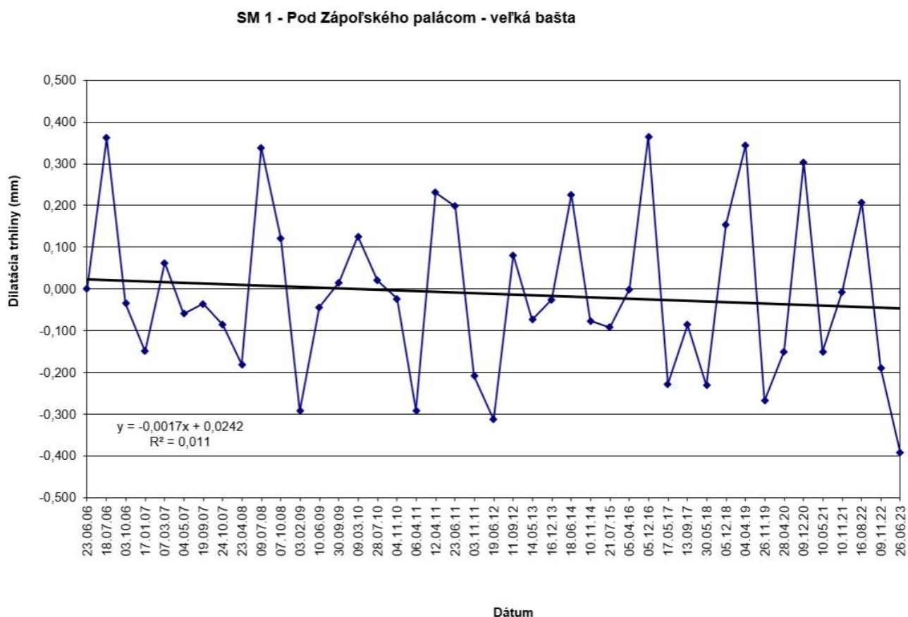
Obr. 25 Výsledky meraní pohybu blokov dilatometrom SM 1 na Trenčianskom hrade v rokoch 2006 – 2023.
