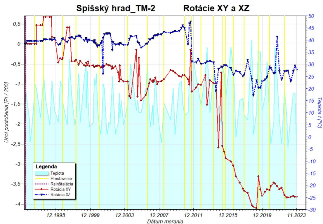
Obr. 11b Graf rotácií travertínových blokov v horizontálnej (XY) a vertikálnej (XZ) rovine zostavený na základe údajov z dilatometra TM-71-2 za monitorovacie obdobie 1992 – 2023.
