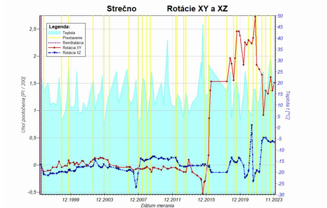
Obr. 23b Graf rotácií bloku (previsu) v horizontálnej (XY) a vertikálnej (XZ) rovine zostavený na základe údajov z dilatometra TM-71 inštalovaného v trhlíne pod kaplnkou hradu Strečno za monitorovacie obdobie 1996 – 2023.
