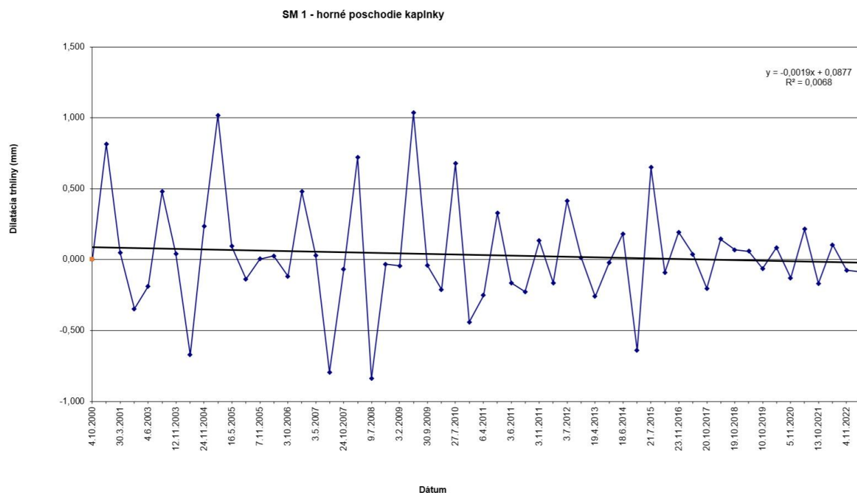
Obr. 29 Výsledky meraní pohybu blokov dilatometrom SM 1 na Uhrovskom hrade v rokoch 2000 – 2023.
