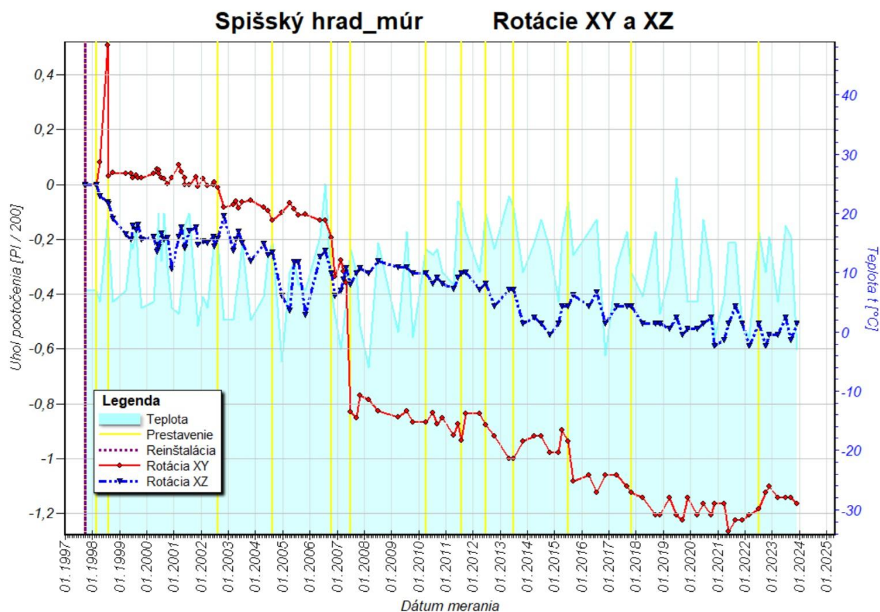
Obr. 14b Graf rotácií travertínových blokov v horizontálnej (XY) a vertikálnej (XZ) rovine zostavený na základe údajov z dilatometra TM-71-h2 (múr) za monitorovacie obdobie 1997 – 2023.
