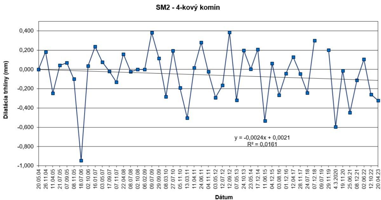
Obr. 33 Výsledky meraní pohybu blokov dilatometrom SM 2 na Pajštúnskom hrade v rokoch 2004 – 2023.
