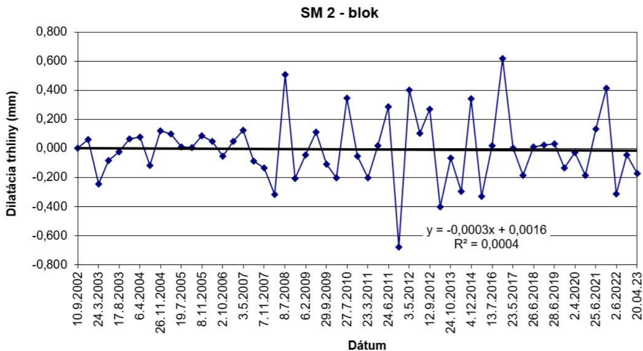
Obr. 39 Výsledky meraní pohybu blokov dilatometrom SM2 na Plaveckom hrade v rokoch 2002 – 2023
