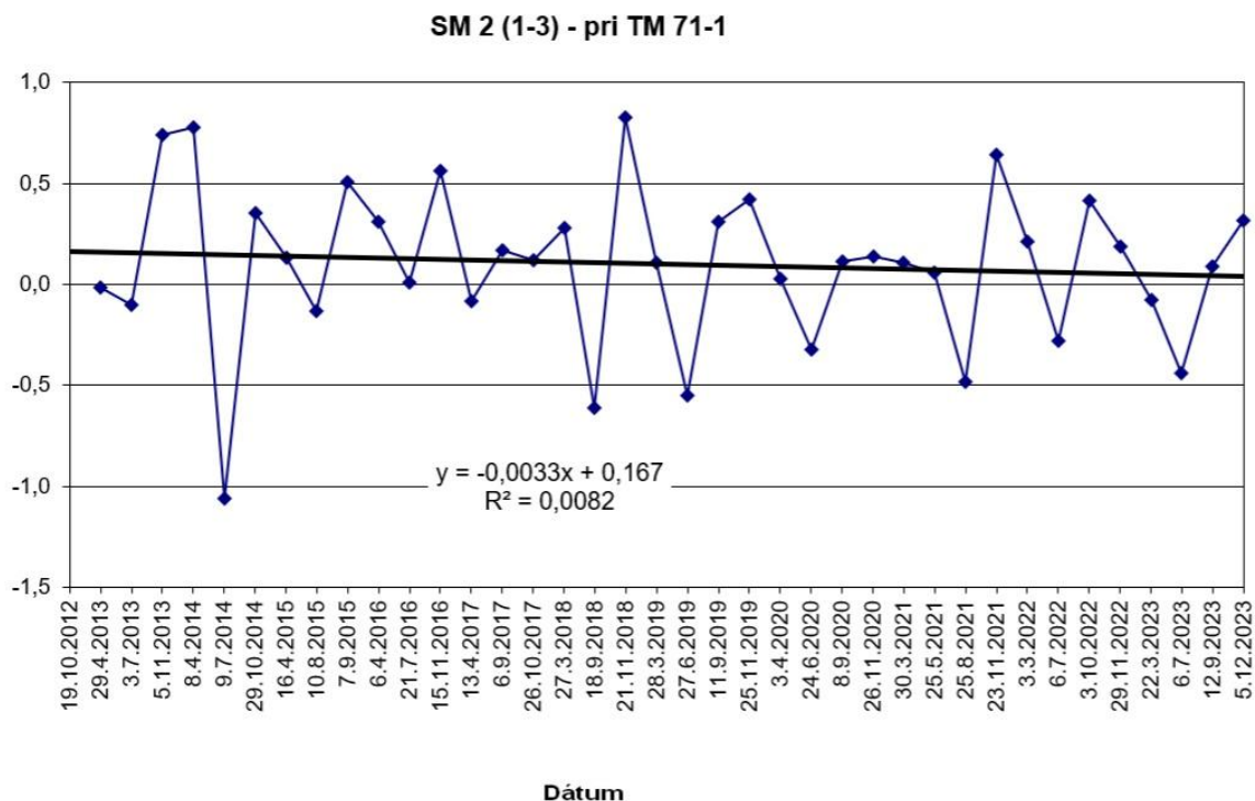
Obr. 9 Výsledky meraní pohybu blokov dilatometrom SM 2 (medzi monitorovacími bodmi 1 – 3) na lokalite Spišský hrad v rokoch 2012 – 2023
