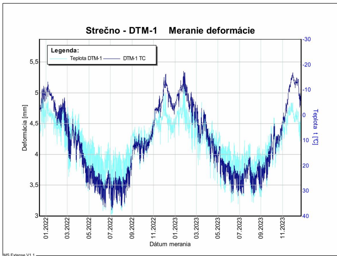
Obr. 23c Graf merania deformácií DTM-1 (prístroj GEOKON-1).
