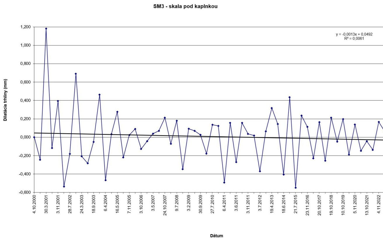
Obr. 31 Výsledky meraní pohybu blokov dilatometrom SM 3 na Uhrovskom hrade v rokoch 2000 – 2023
