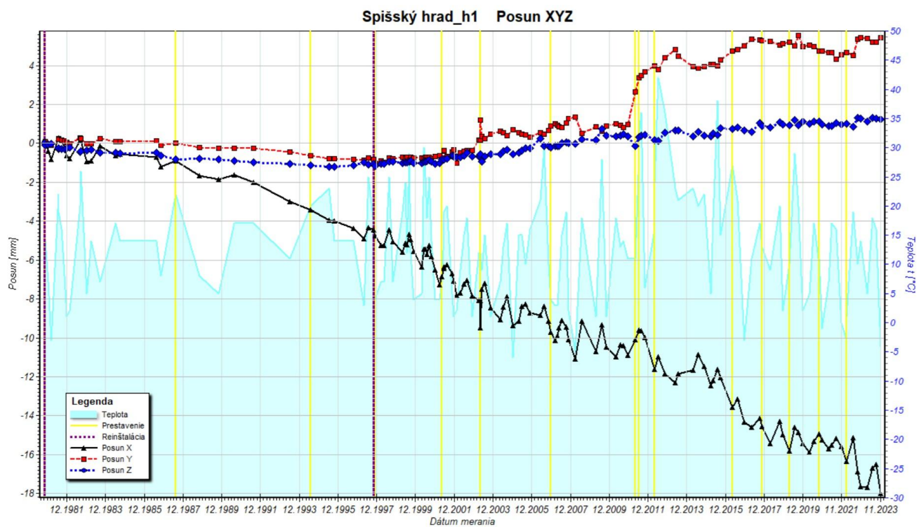
Obr. 6a Graf posunu travertínových blokov pozdĺž osí X,Y a Z zostavený na základe údajov z dilatometra TM-71- h1 za monitorovacie obdobie 1980 – 2023.
