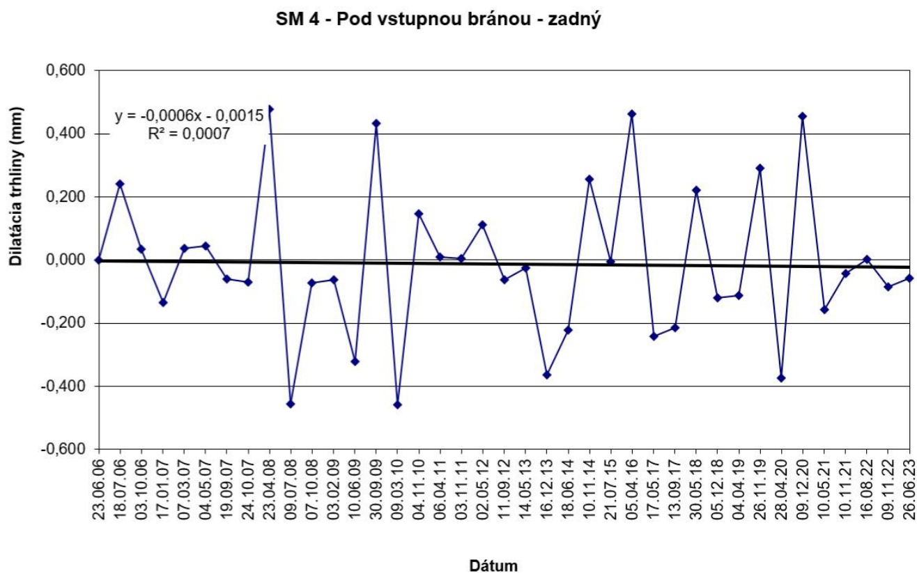
Obr. 27 Výsledky meraní pohybu blokov dilatometrom SM 4 na Trenčianskom hrade v rokoch 2006 – 2023.
