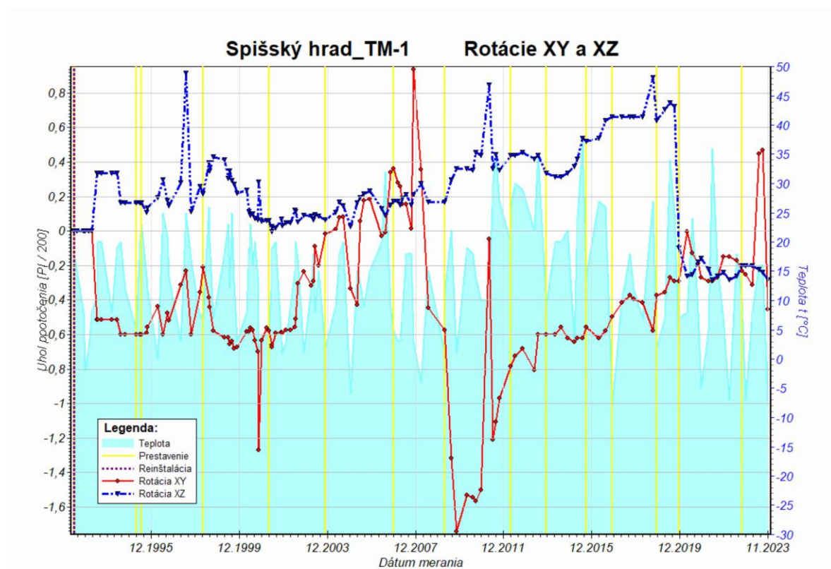
Obr. 8b Graf rotácii travertínových blokov v horizontálnej (XY) a vertikálnej (XZ) rovine zostavený na základe údajov z dilatometra TM-71-1 za monitorovacie obdobie 1992 – 2023.
