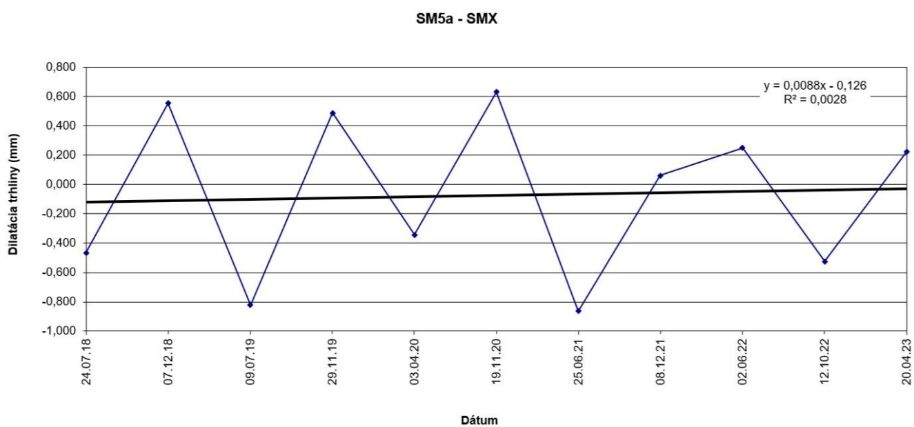
Obr. 36 Výsledky meraní pohybu blokov dilatometrom SM 5a na Pajštúnskom hrade v rokoch 2018 – 2023.
