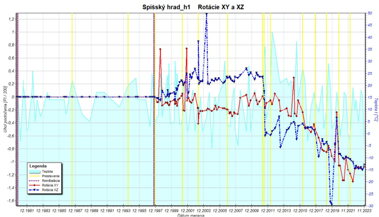
Obr. 6b Graf rotácií travertínových blokov v horizontálnej (XY) a vertikálnej (XZ) rovine zostavený na základe údajov z dilatometra TM-71-h1 za monitorovacie obdobie 1980 – 2023.
