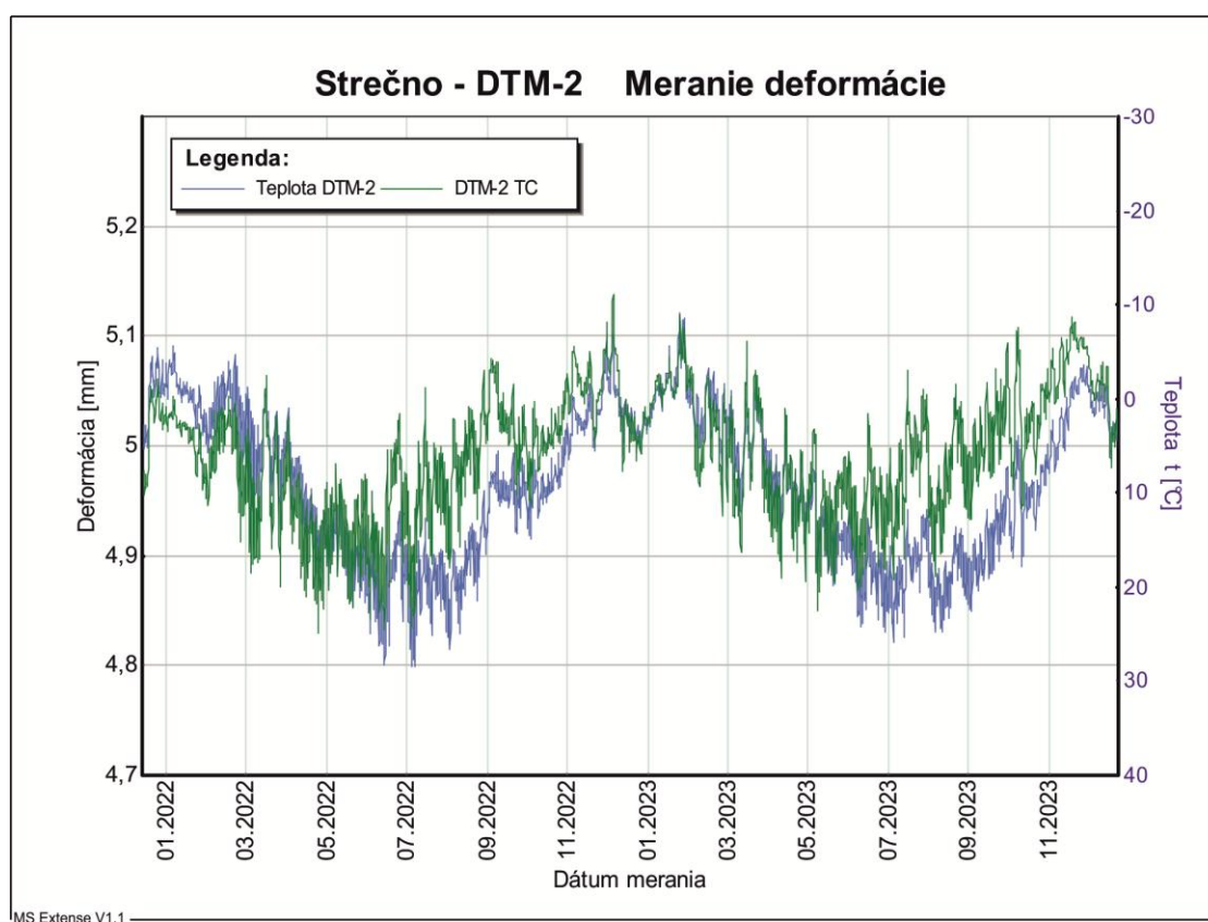
Obr. 23d Graf merania deformácií DTM-2 (prístroj GEOKON-2).
