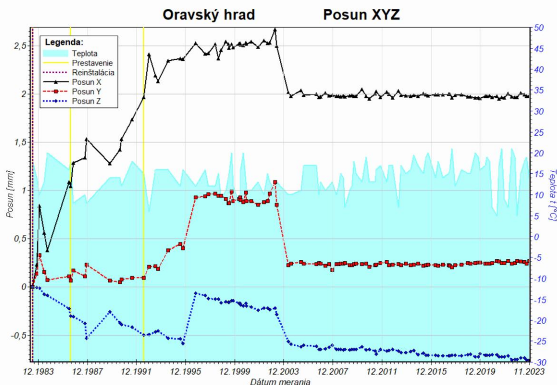
Obr. 21 Graf posunu blokov pozdĺž osí x, y a z zostavený na základe údajov z dilatometra TM-71 (starý typ) na Oravskom hrade za monitorovacie obdobie 1983 – 2023.
