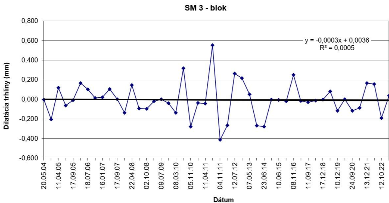
Obr. 40 Výsledky meraní pohybu blokov dilatometrom SM3 na Plaveckom hrade v rokoch 2004 – 2023
