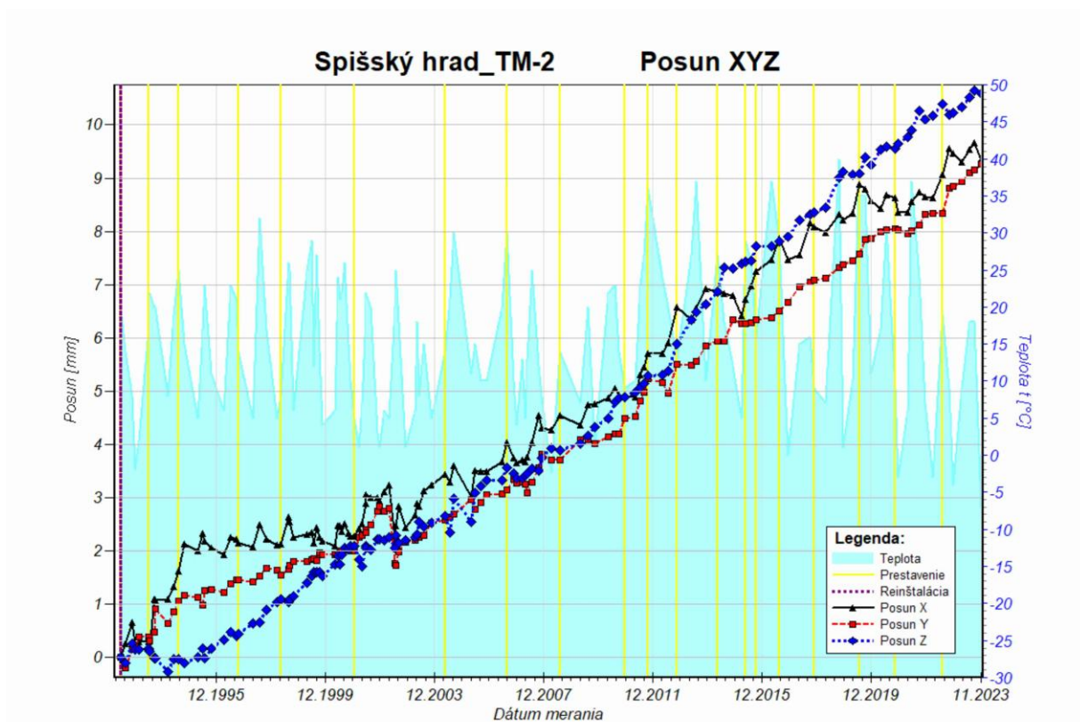
Obr. 11a Graf posunu travertínových blokov pozdĺž osí x, y a z zostavený na základe údajov z dilatometra TM-71-2 za monitorovacie obdobie 1992 – 2023.
