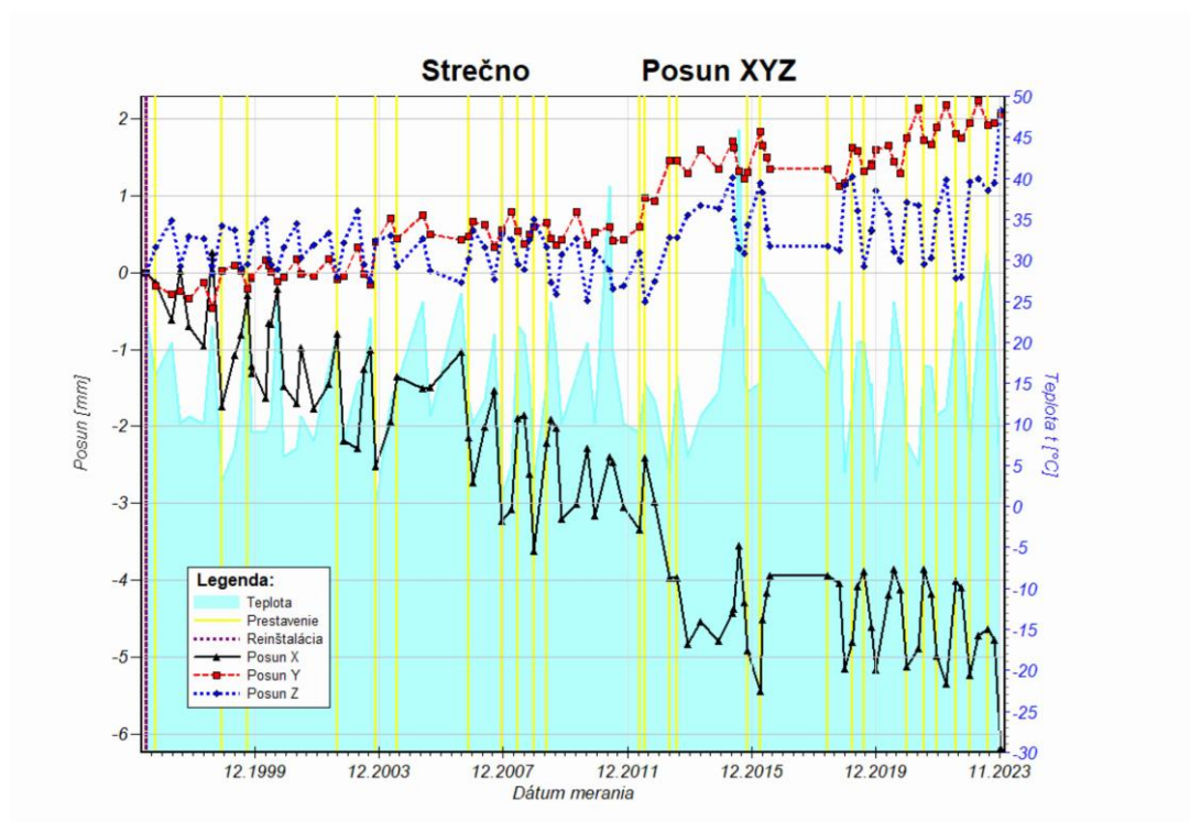
Obr. 23a Graf posunu blokov pozdĺž osí x, y a z zostavený na základe údajov z dilatometra TM-71 inštalovaného v trhlíne pod kaplnkou hradu Strečno za monitorovacie obdobie 1996 – 2023.
