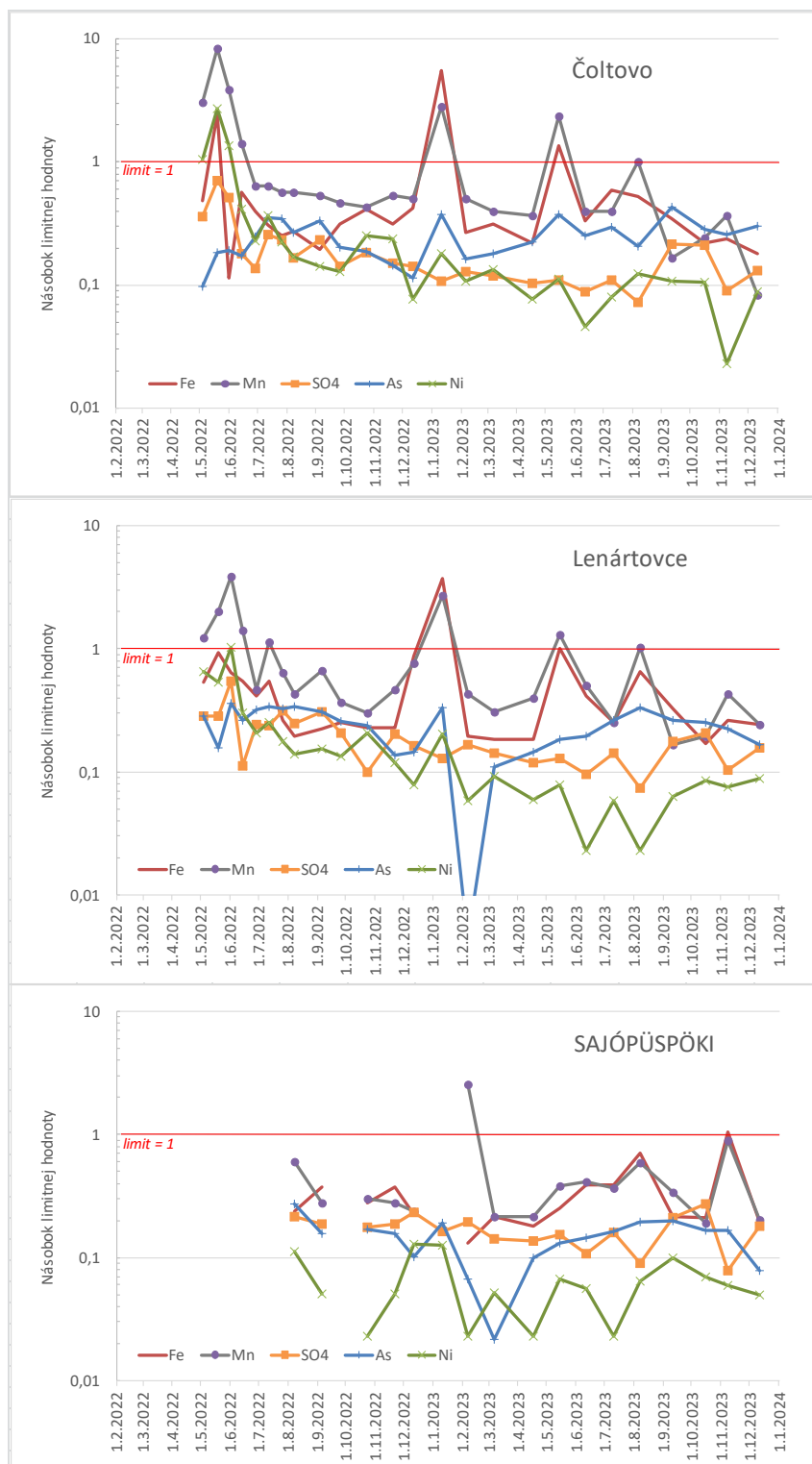
Obr. 4.7.4: Miera prekročenia limitných hodnôt pre povrchové vody vo vzorkách vody z rieky Slaná (podľa údajov SVP)
