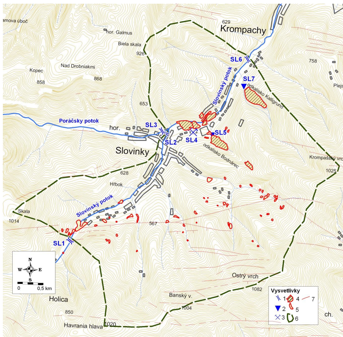
Obr. 4.8.2 Lokalizácia monitorovacích objektov na lokalite Slovinky. Vysvetlivky: 1 – monitorovaný profil povrchového toku, 2 – monitorovaná drenáž odkaliska, 3 – monitorované ústie štôľne, 4 – odkalisko, 5 – halda, 6 – rozvodnica, 7 – rudná žila.
