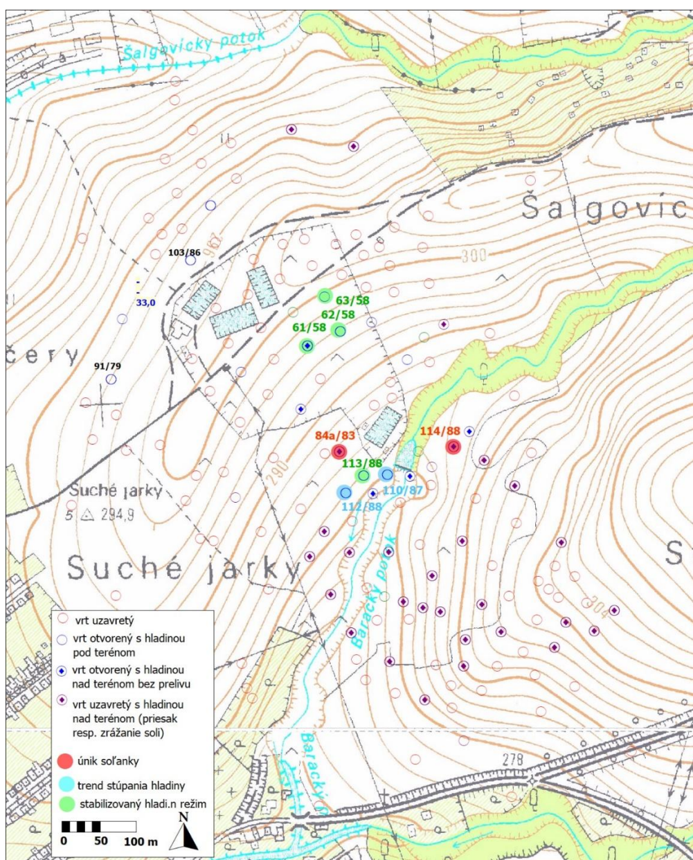
Obr. 4.13.3 Výšková úroveň a úniky soľanky v ťažobných vrtoch v lúhovacom poli soľného ložiska Prešov – Solivary v roku 2023.
