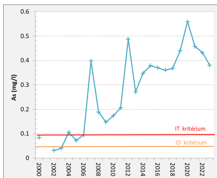
Obr. 4.8.1: Ročné mediány obsahu arzénu vo vode štôlne Alžbeta pre obdobie rokov 2000 – 2023.
