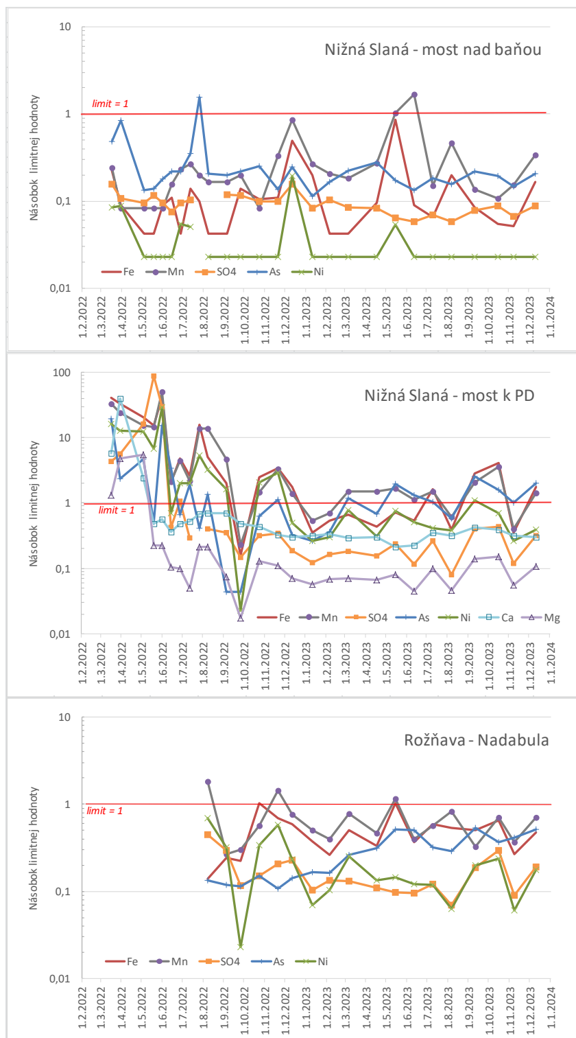
Obr. 4.7.3: Miera prekročenia limitných hodnôt pre povrchové vody vo vzorkách vody z rieky Slaná (podľa údajov SVP)
