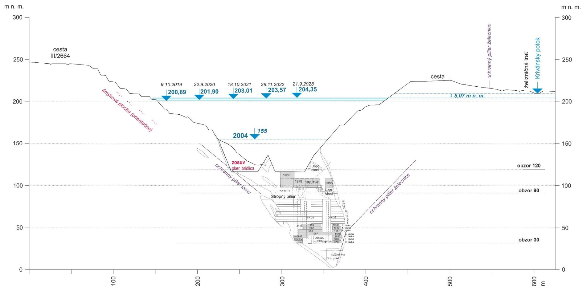
Obr. 4.12.2 Rez ložiskom – šošovky II. s použitím podkladov Dianiška (1990) s vyznačením zisťovanej úrovne hladiny vody v ťažobnom lome
