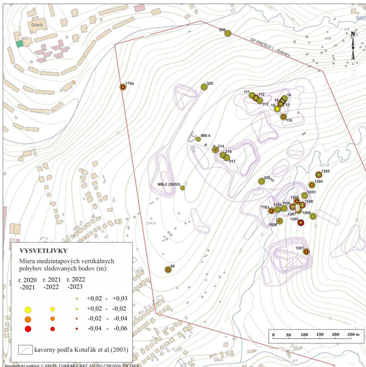
Obr. 4.13.5: Mapa medzietapových vertikálnych pohybov sledovaných bodov v období r. 2020 – 2023
