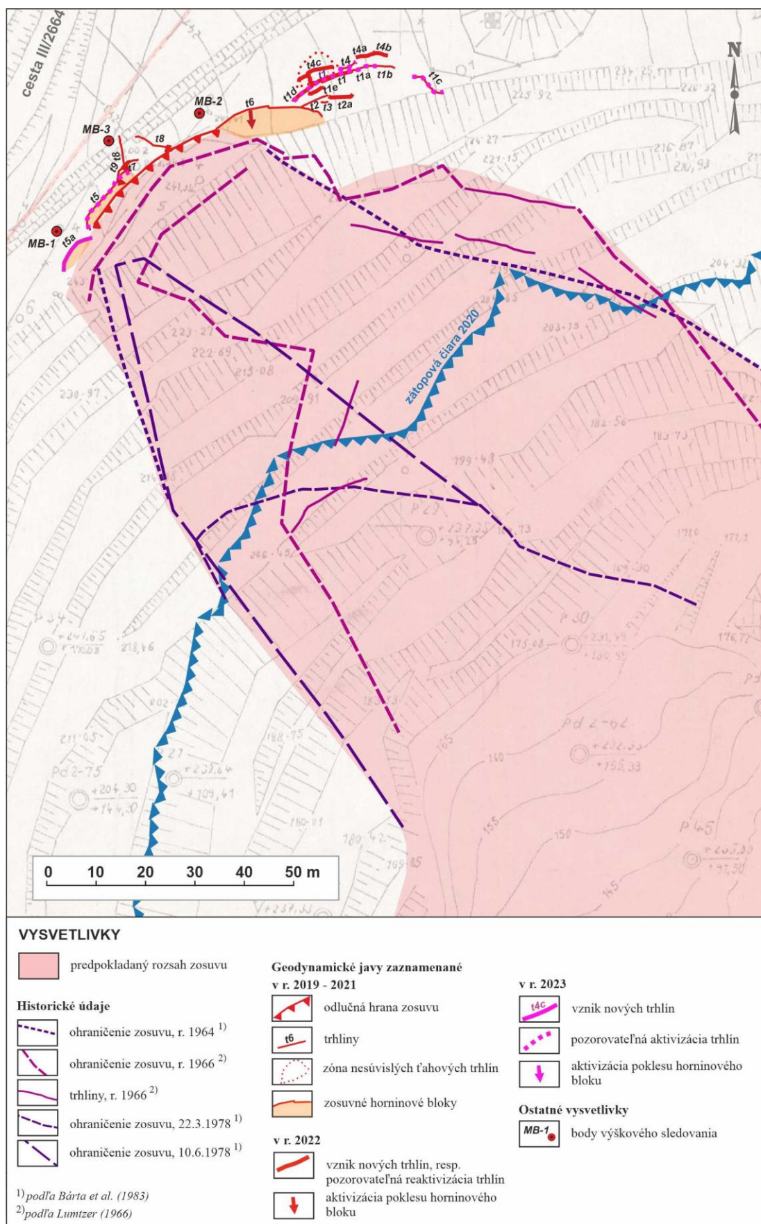
Obr. 4.12.3: Situácia zosuvu s približným označením zátopovej čiary podľa snímky Lidar-u z r. 2020 (zdroj: https://zbgis.skgeodesy.sk/mkzbgis/sk/teren ), (topograf. podklad: Dianiška, 1990)
