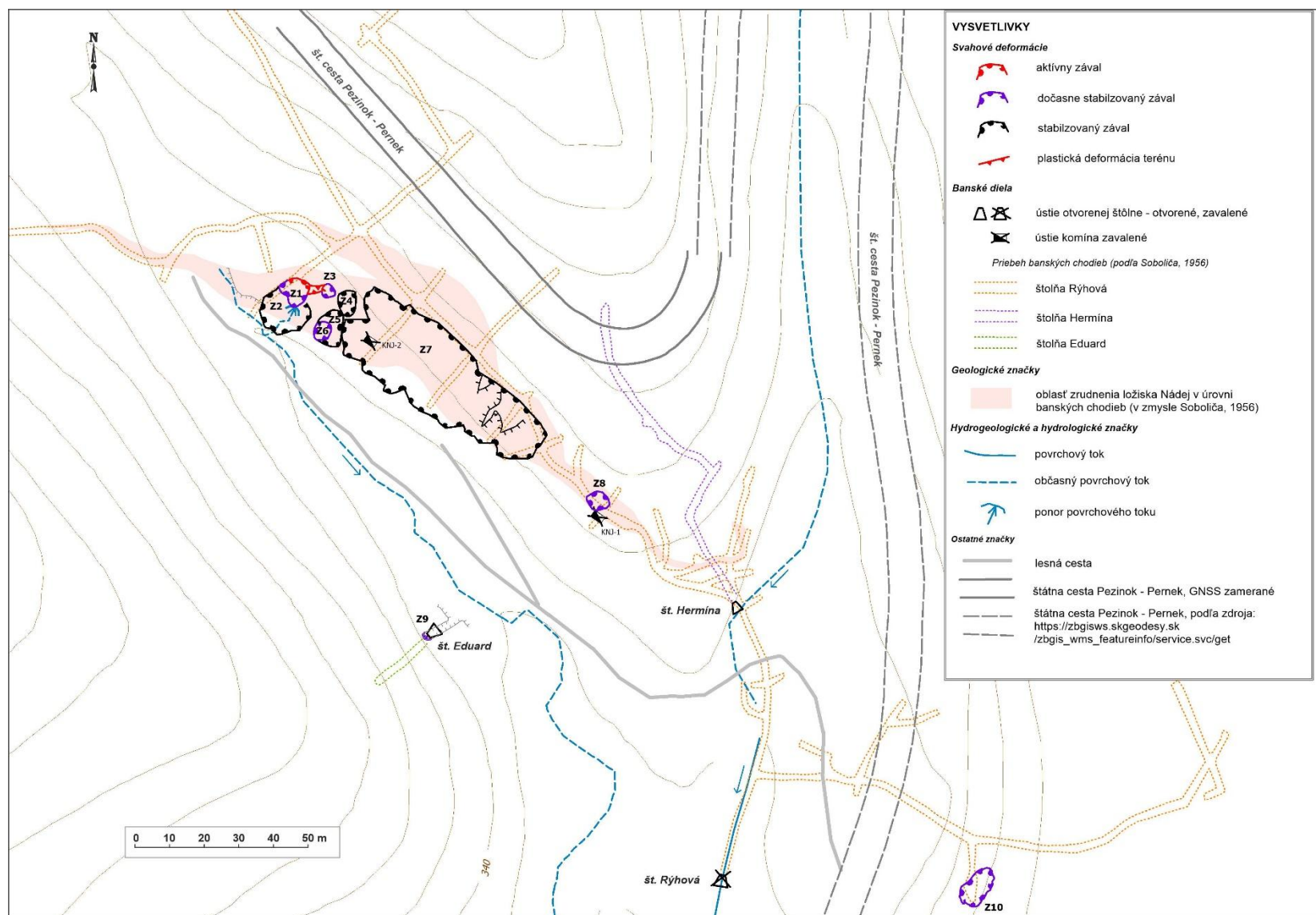
Obr. 4.4.2: Situácia závalov v oblasti ložiska Nádej (s použitím podkladov Sobolíč, 1956 a Mašlár et al., 2001).
