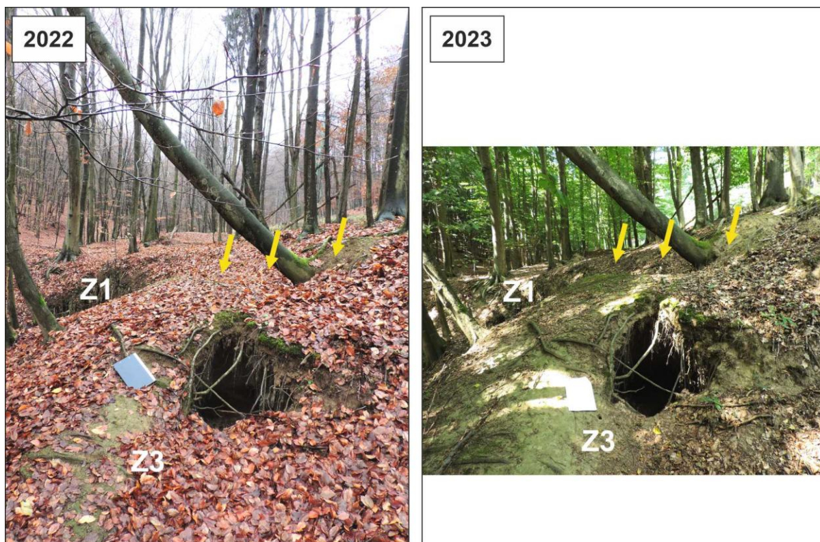
Obr. 4.4.8 Pokles povrchu terénu medzi závalmi Z1 a Z3 s pozorovaným nakláňaním kmeňov stromov, stav z r. 2022 a 2023
