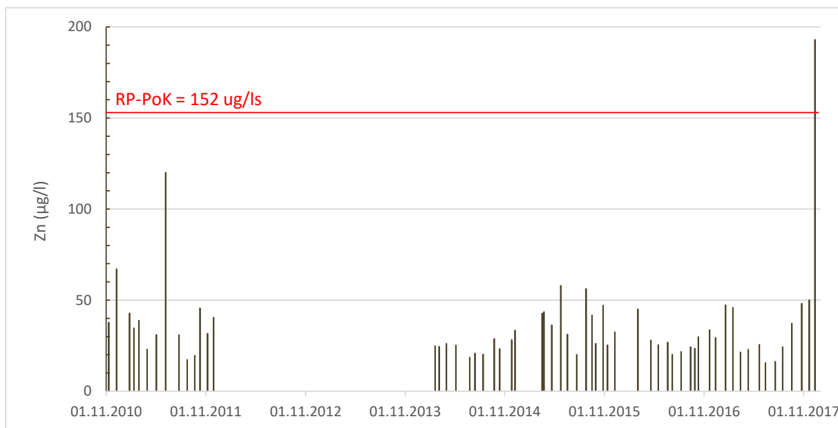
Obr. 4.1.1 Obsah zinku vo vode Hodruškého potoka na monitorovacom mieste SHMÚ R228000D „pod Dolnými Hámrami“ v období rokov 2010 – 2017 (podľa údajov SHMÚ)
