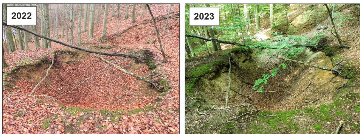
Obr. 4.4.11: Zával na ložisku Kristína nad chodbou štôlne Rýhová, stav z r. 2022 a r. 2023
