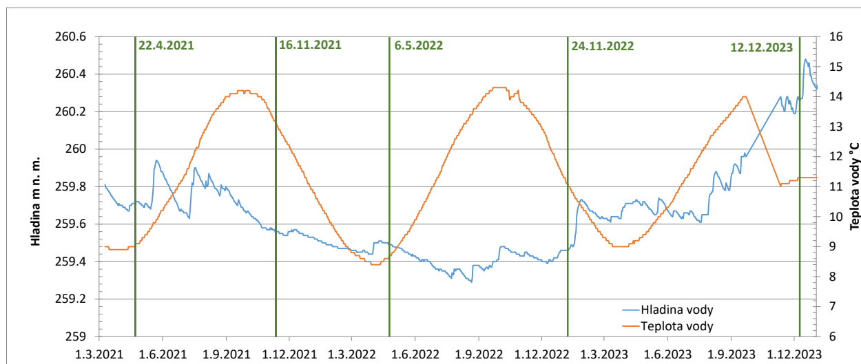
Obr. 4.13.1: Zmeny úrovne hladiny a teploty vody v sonde SHMÚ č. 1111 vo Veľkom Šariši v rokoch 2021 – 2023 s vyznačením doby merania hladiny vo vrtoch lúhovacieho poľa v Solivaroch
