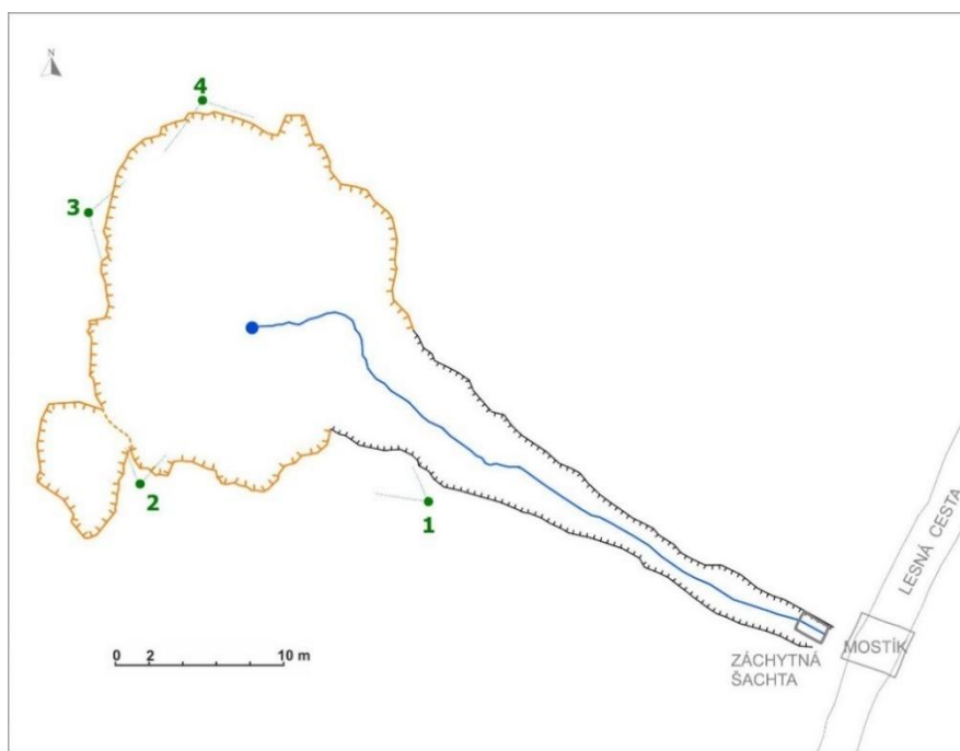
Obr. 4.11.2: Situácia závalov v oblasti Novej štôľne
