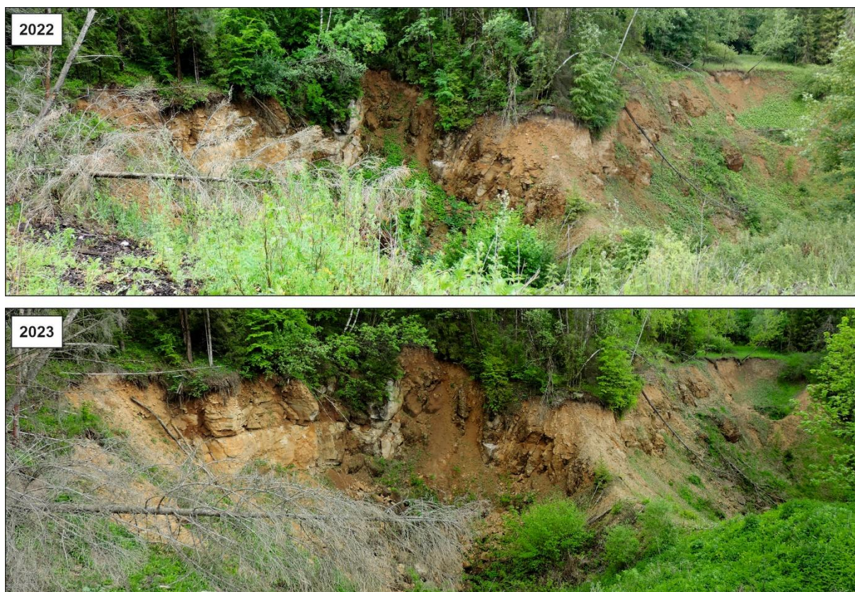
Obr. 4.11.5 Porovnávacie fotografické snímky juhovýchodného okraja závalu Z3 z r. 2022 a 2023
