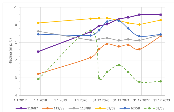
Obr. 4.13.2: Časový vývoj úrovne hladiny vody v niektorých ťažobných vrtoch lúhovacieho poľa Prešov – Solivary v období rokov 2017 – 2023
