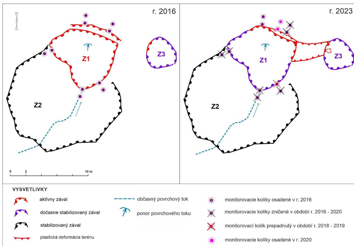
Obr. 4.4.3: Orientačný situačný náčrt závalov Z1 a Z2 s lokalizáciou monitorovacích vytyčovacích kolíkov so stavom k r. 2016 a 2023
