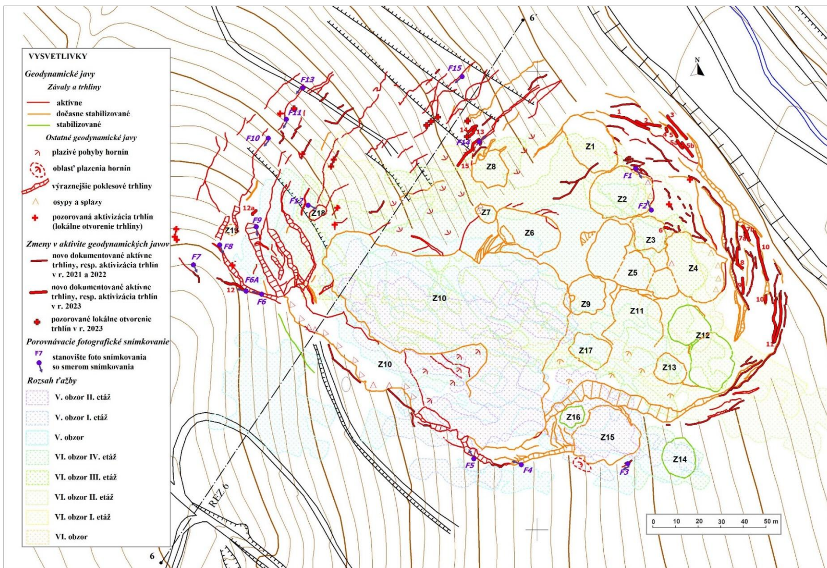
Obr. 4.7.7 Mapa závalov na ložisku Kobeliarovo so zobrazením dokumentovaných zmien v r. 2023 a so znázornením rozsahu ťažby získanom spracovaním mapových podkladov zo Slovenského banského archívu v Banskej Štiavnici (topografický podklad: Ščuka et al., 1982)
