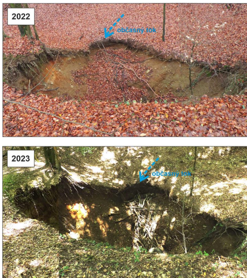
Obr. 4.4.6: Zával Z1 nad banskou chodbou štôlne Rýhová dokumentovaný v r. 2022 a 2023 (pohľad zo severu)
