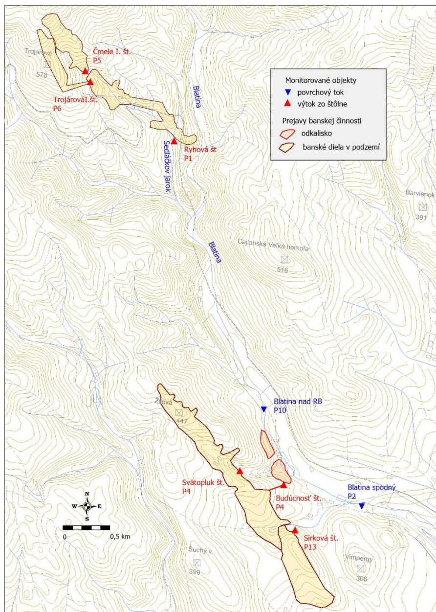
Obr. 4.4.1: Situácia monitorovaných objektov na lokalite Pezinok.
