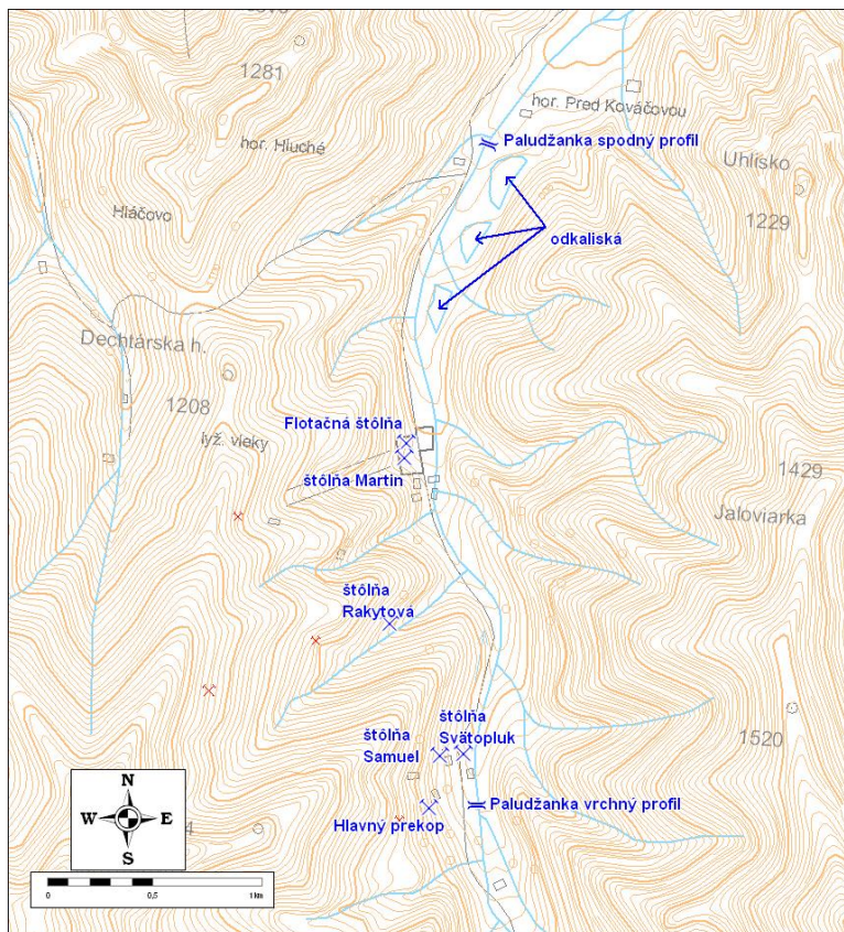
Obr. 4.3.1: Situácia monitorovaných objektov na lokalite Dúbrava
