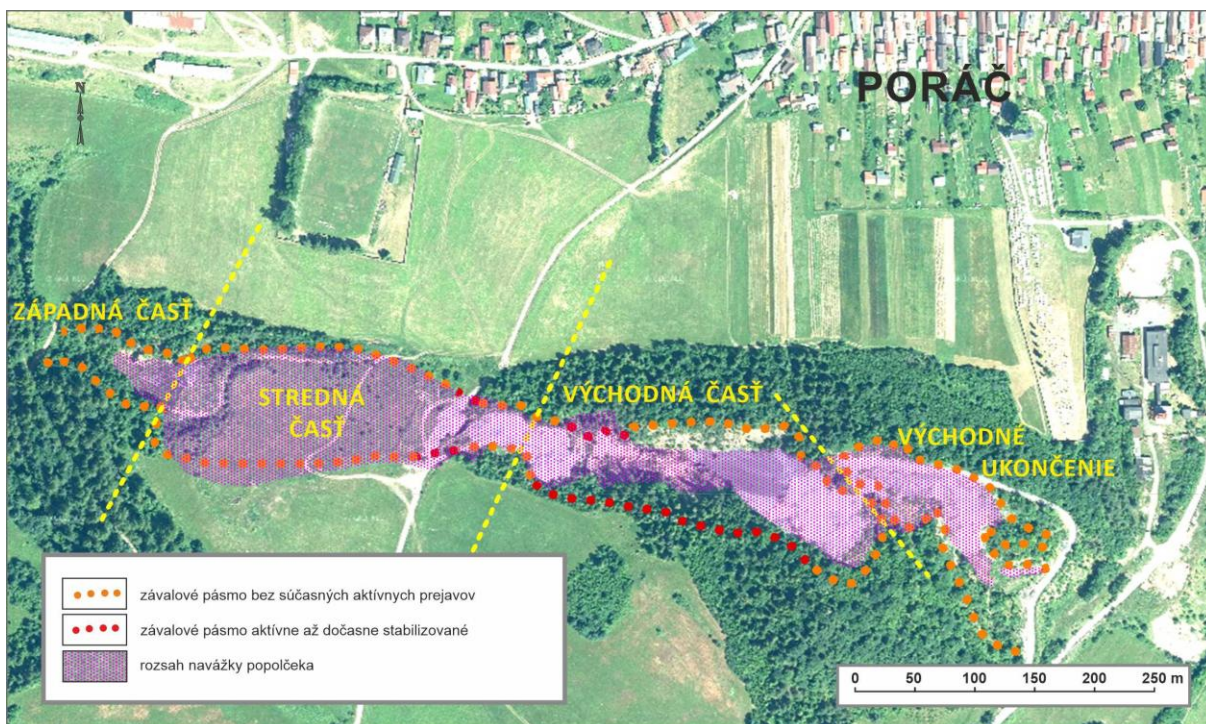
Obr. 4.6.2: Rozsah zavážania závalového pásma Baniská popolčekom s vymedzením úsekov podľa aktuálnej aktivity deformácií povrchu územia vplyvom ťažby so stavom k r. 2023 (topograf. podklad – zdroj: https://zbgisws.sk/geodesy.sk/zbgis_ortofoto_wms/service.svc/get )
