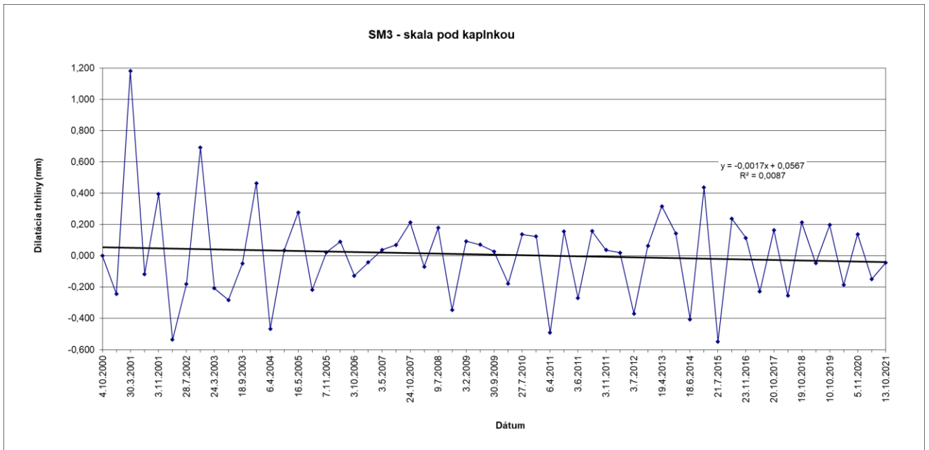
Obr. 32 Výsledky meraní pohybu blokov dilatometrom SM 3 na Uhrovskom hrade v rokoch 2000 – 2021
