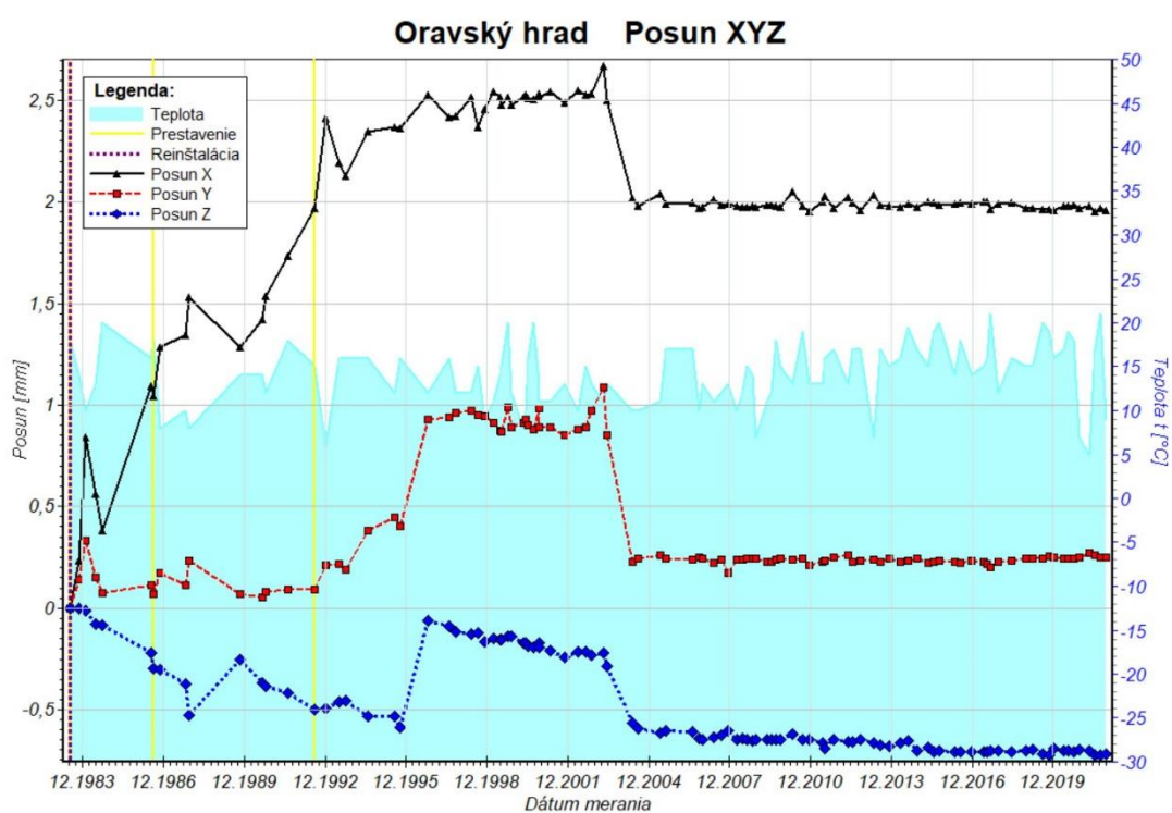
Obr. 21 Graf posunu blokov pozdĺž osí x, y a z zostavený na základe údajov z dilatometra TM-71 (starý typ) na Oravskom hrade za monitorovacie obdobie 1983 – 2021.
