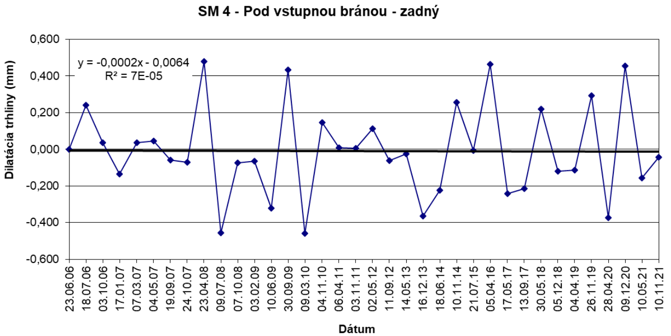
Obr. 28 Výsledky meraní pohybu blokov dilatometrom SM 4 na Trenčianskom hrade v rokoch 2006 – 2021.
