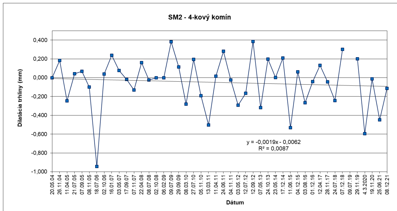
Obr. 34 Výsledky meraní pohybu blokov dilatometrom SM 2 na Pajštúnskom hrade v rokoch 2004 – 2021.
