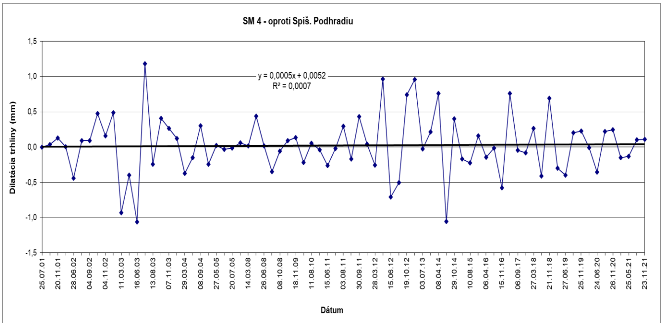
Obr. 18: Výsledky meraní pohybu blokov dilatometrom SM 4 na lokalite Spišský hrad za monitorovacie obdobie 2001 – 2021
