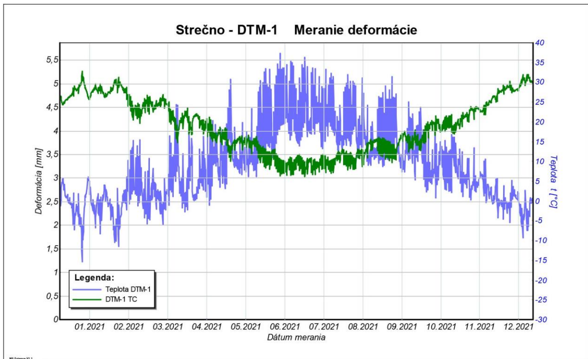
Obr. 23c Graf merania deformácií DTM-1 (prístroj GEOKON-1).
