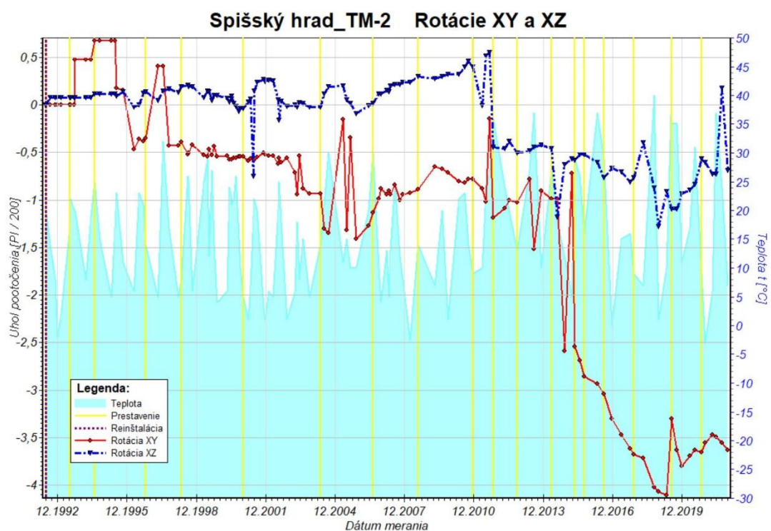
Obr. 11b Graf rotácií travertínových blokov v horizontálnej (XY) a vertikálnej (XZ) rovine zostavený na základe údajov z dilatometra TM-71-2 za monitorovacie obdobie 1992 – 2021.
