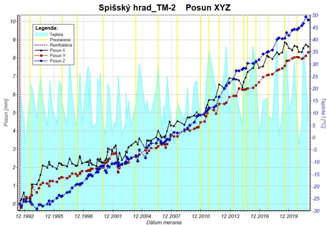
Obr. 11a Graf posunu travertínových blokov pozdĺž osí x, y a z zostavený na základe údajov z dilatometra TM-71-2 za monitorovacie obdobie 1992 – 2021.
