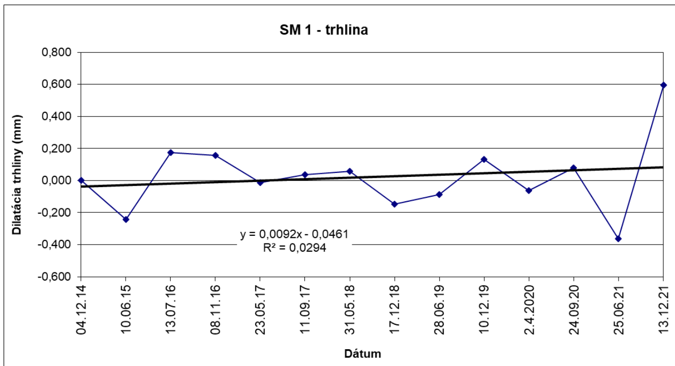
Obr. 38 Výsledky meraní pohybu blokov dilatometrom novým profilom SM 1 na Plaveckom hrade dilatometrom v rokoch 2014 – 2021
