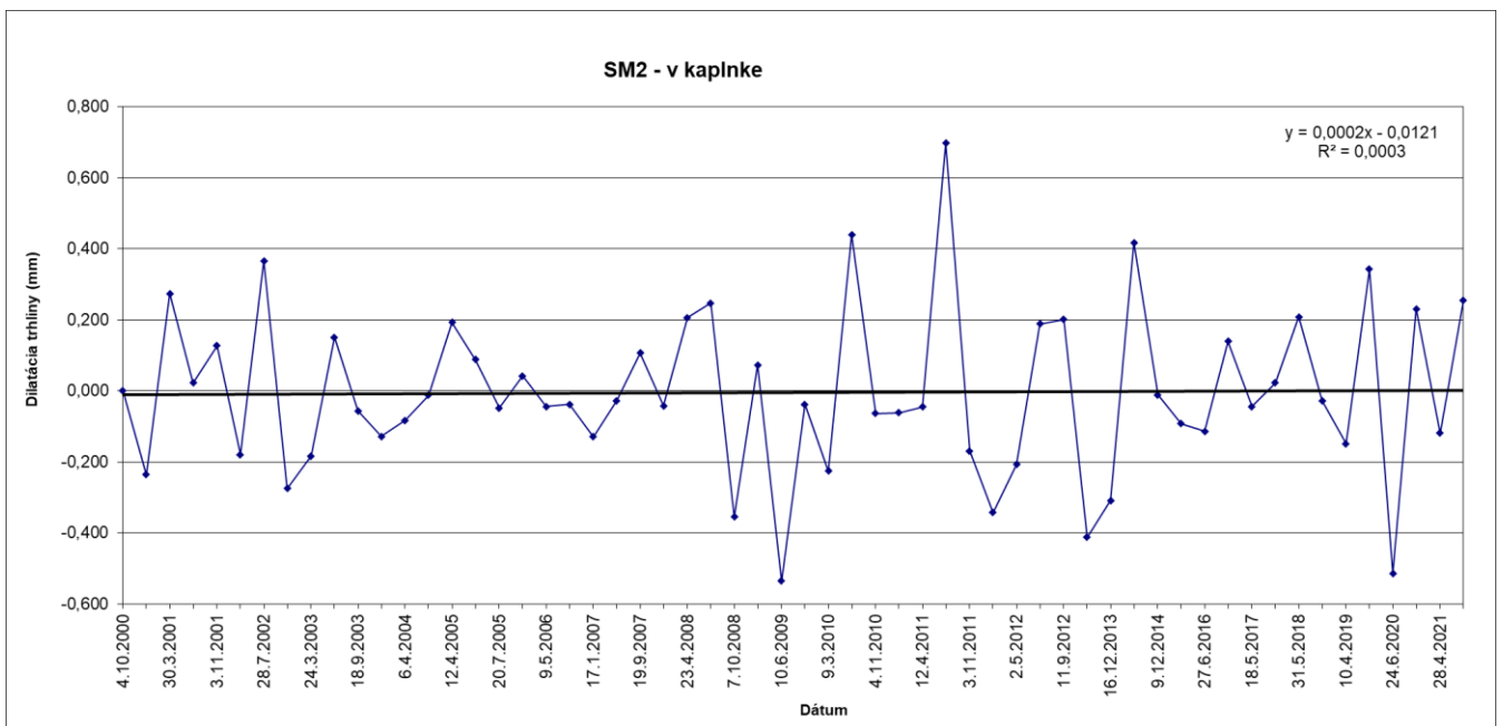
Obr. 31 Výsledky meraní pohybu blokov dilatometrom SM 2 na Uhrovskom hrade v rokoch 2000 – 2021
