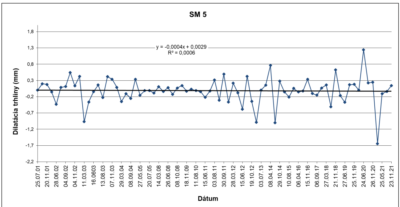
Obr. 19 Výsledky meraní pohybu blokov dilatometrom SM 5 na lokalite Spišský hrad za monitorovacie obdobie 2001 – 2021
