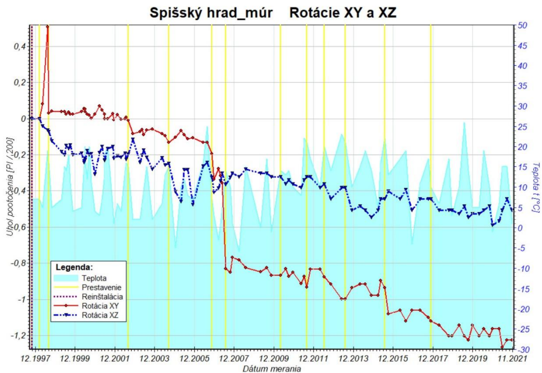
Obr. 14b Graf rotácií travertínových blokov v horizontálnej (XY) a vertikálnej (XZ) rovine zostavený na základe údajov z dilatometra TM-71-h2 (múr) za monitorovacie obdobie 1997 – 2021.
