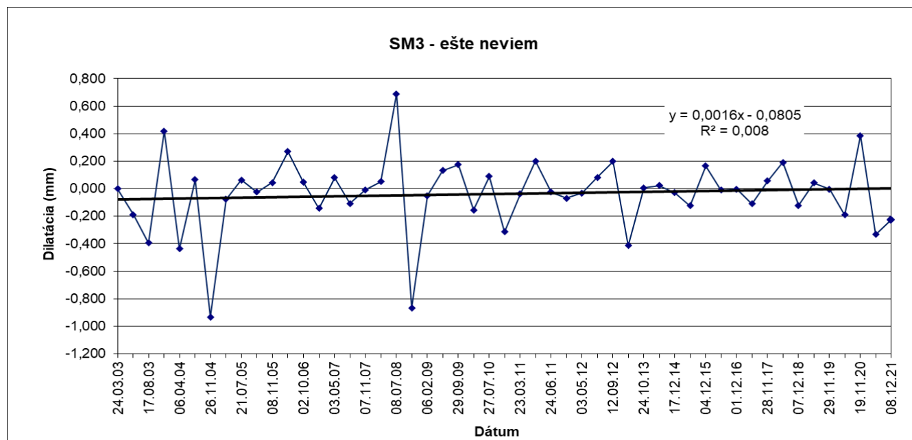
Obr. 35 Výsledky meraní pohybu blokov dilatometrom SM 3 na Pajštúnskom hrade v rokoch 2003 – 2021.
