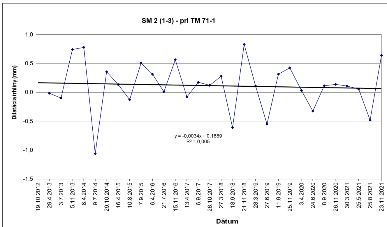
Obr. 9 Výsledky meraní pohybu blokov dilatometrom SM 2 (medzi monitorovacími bodmi 1 – 3) na lokalite Spišský hrad v rokoch 2012 – 2021
