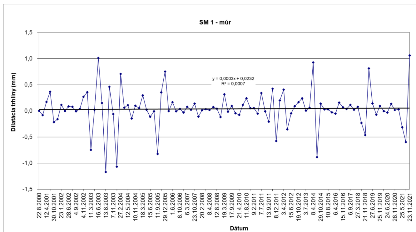
Obr.15 Výsledky meraní pohybu blokov dilatometrom SM 1 na lokalite Spišský hrad v rokoch 2000 – 2021
