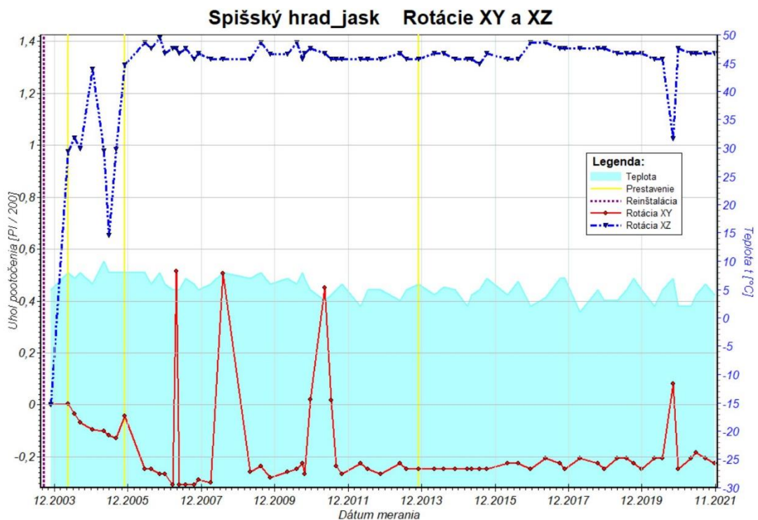
Obr. 17b Graf rotácií travertínových blokov v horizontálnej (XY) a vertikálnej (XZ) rovine zostavený na základe údajov z dilatometra TM-71-jaskyňa za monitorovacie obdobie 2003 – 2021.
