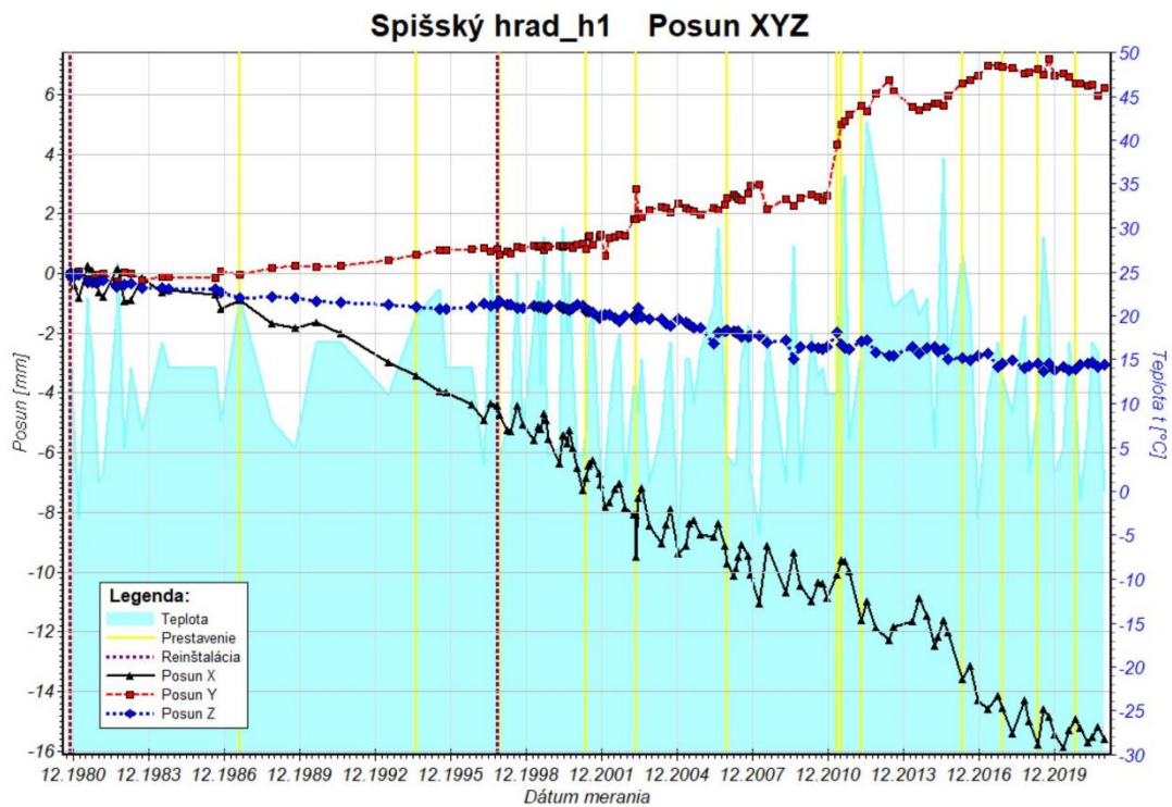
Obr. 6a Graf posunu travertínových blokov pozdĺž osí X,Y a Z zostavený na základe údajov z dilatometra TM-71- h1 za monitorovacie obdobie 1980 – 2021.
