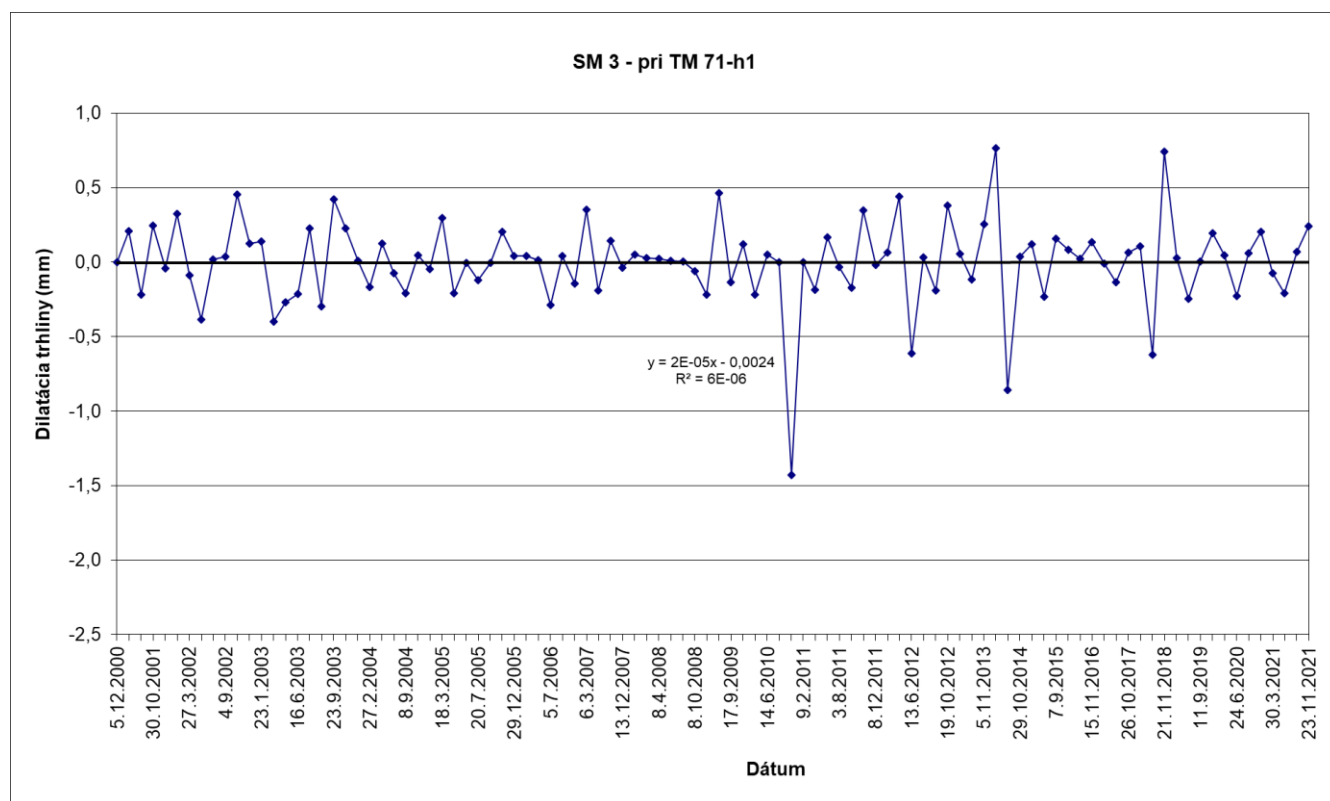
Obr. 7 Výsledky meraní pohybu blokov dilatometrom SM 3 na Spišskom hrade v období rokov 2000 – 2021
