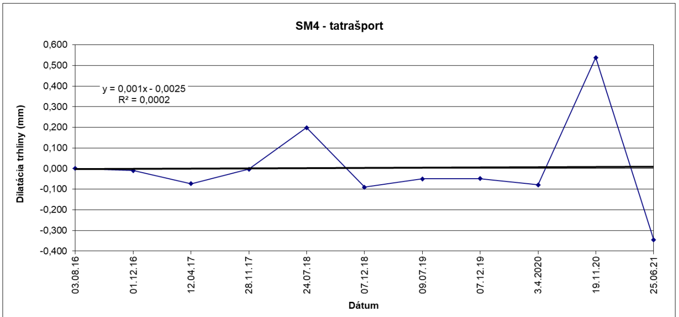
Obr. 36 Výsledky meraní pohybu blokov dilatometrom SM 4 na Pajštúnskom hrade v rokoch 2016 – 2021.
