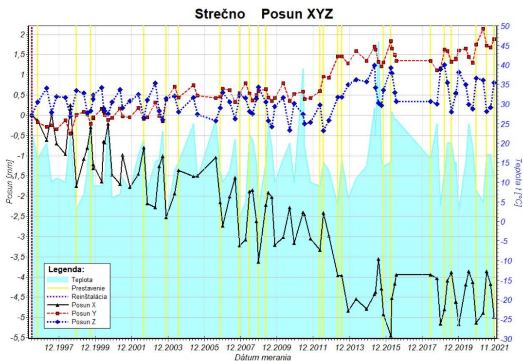
Obr. 23a Graf posunu blokov pozdĺž osí x , y a z zostavený na základe údajov z dilatometra TM-71 inštalovaného v trhline pod kaplnkou hradu Strečno za monitorovacie obdobie 1996 – 2021.
