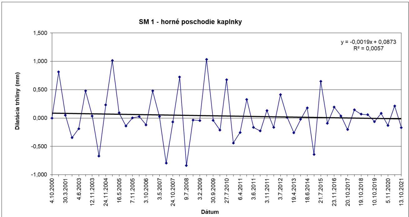
Obr. 30 Výsledky meraní pohybu blokov dilatometrom SM 1 na Uhrovskom hrade v rokoch 2000 – 2021.
