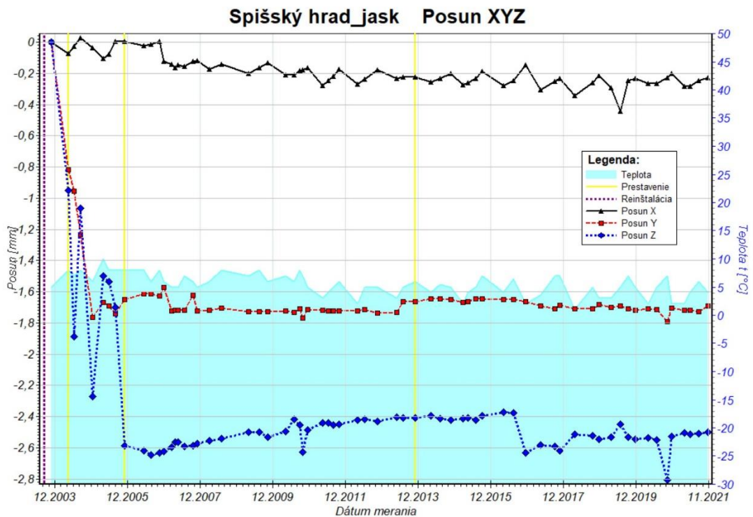
Obr. 17a Graf posunu travertínových blokov pozdĺž osí x, y a z zostavený na základe údajov z dilatometra TM- 71-jaskyňa za monitorovacie obdobie 2003 – 2021.
