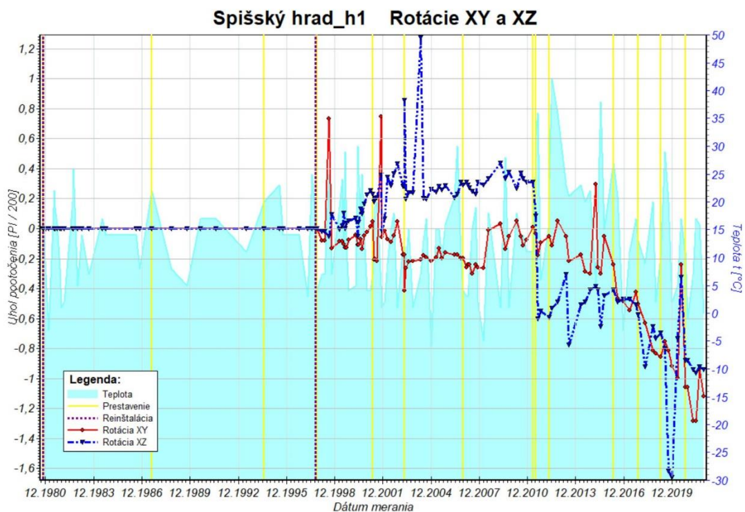
Obr. 6b Graf rotácií travertínových blokov v horizontálnej (XY) a vertikálnej (XZ) rovine zostavený na základe údajov z dilatometra TM-71-h1 za monitorovacie obdobie 1980 – 2021.
