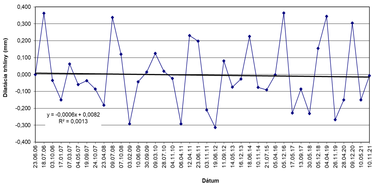
Obr. 25 Výsledky meraní pohybu blokov dilatometrom SM 1 na Trenčianskom hrade v rokoch 2006 – 2021.
