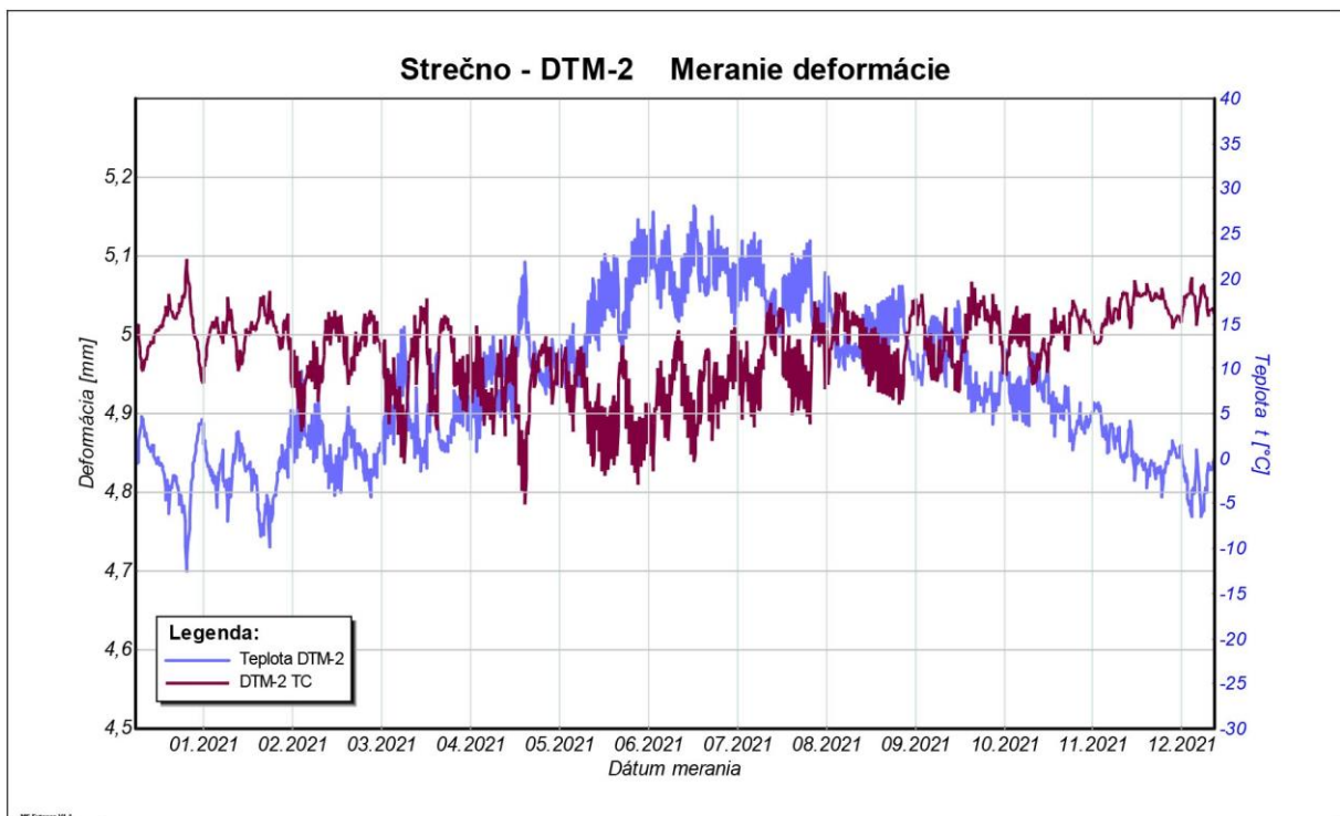
Obr. 23d Graf merania deformácií DTM-2 (prístroj GEOKON-2).
