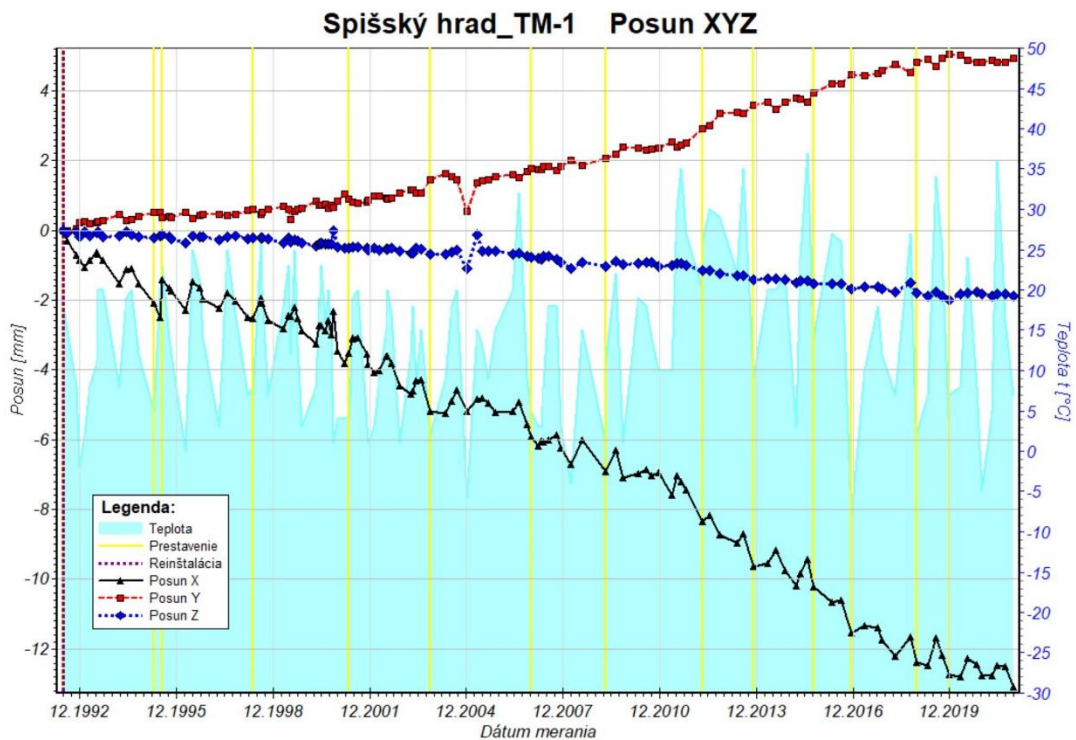
Obr. 8a Graf posunu travertínových blokov pozdĺž osí x, y a z zostavený na základe údajov z dilatometra TM - 71
