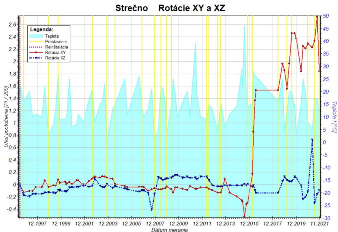
Obr. 23b Graf rotácií bloku (previsu) v horizontálnej (XY) a vertikálnej (XZ) rovine zostavený na základe údajov z dilatometra TM-71 inštalovaného v trhline pod kaplnkou hradu Strečno za monitorovacie obdobie 1996 – 2021.
