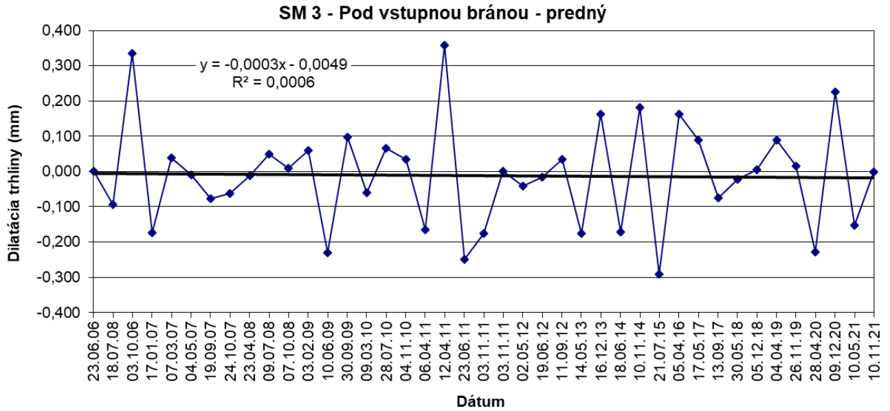
Obr. 27 Výsledky meraní pohybu blokov dilatometrom SM 3 na Trenčianskom hrade v rokoch 2006 – 2021.
