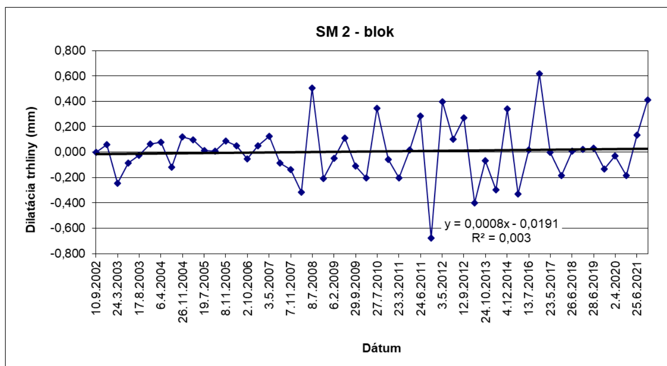
Obr. 39 Výsledky meraní pohybu blokov dilatometrom SM2 na Plaveckom hrade v rokoch 2002 – 2021
