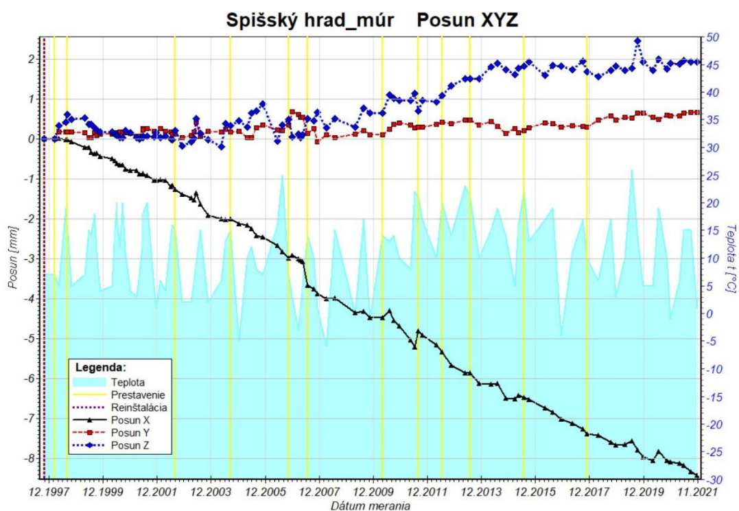
Obr. 14a Graf posunu travertínových blokov pozdĺž osí x, y, z zostavený na základe údajov z dilatometra TM-71-h2 (múr) za monitorovacie obdobie 1997 – 2021.
