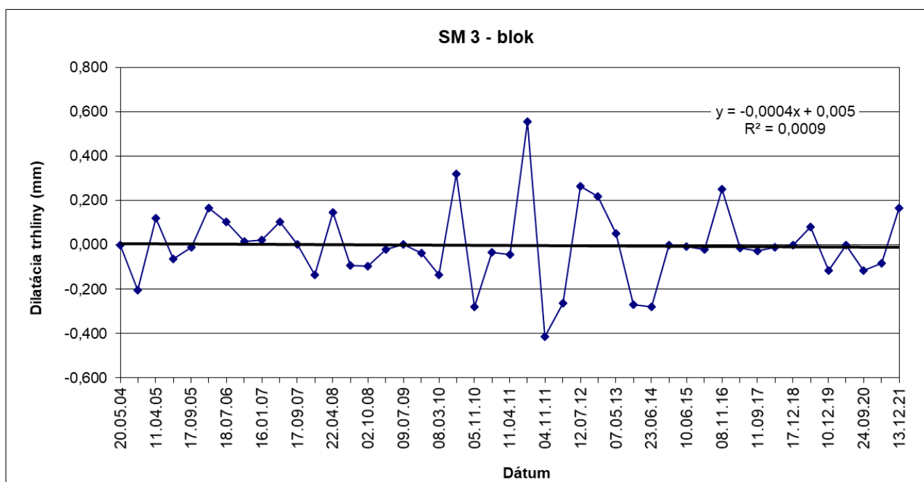
Obr. 40 Výsledky meraní pohybu blokov dilatometrom SM3 na Plaveckom hrade v rokoch 2004 – 2021.
