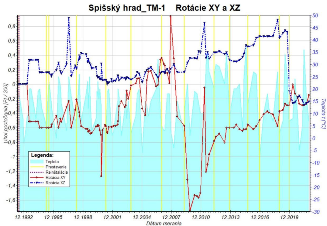
Obr. 8b Graf rotácií travertínových blokov v horizontálnej (XY) a vertikálnej (XZ) rovine zostavený na základe údajov z dilatometra TM-71-1 za monitorovacie obdobie 1992 – 2021.
