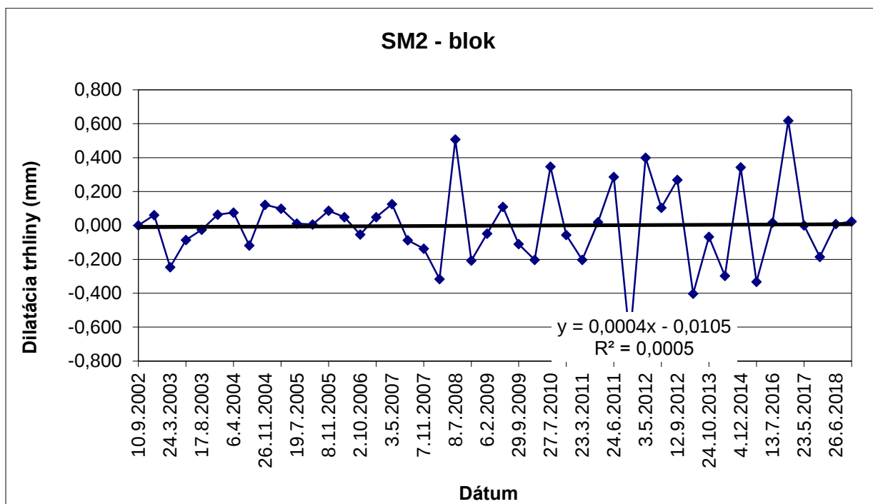
Obr. 40 Výsledky meraní pohybu blokov dilatometrom SM2 na Plaveckom hrade v rokoch 2002 – 2018
