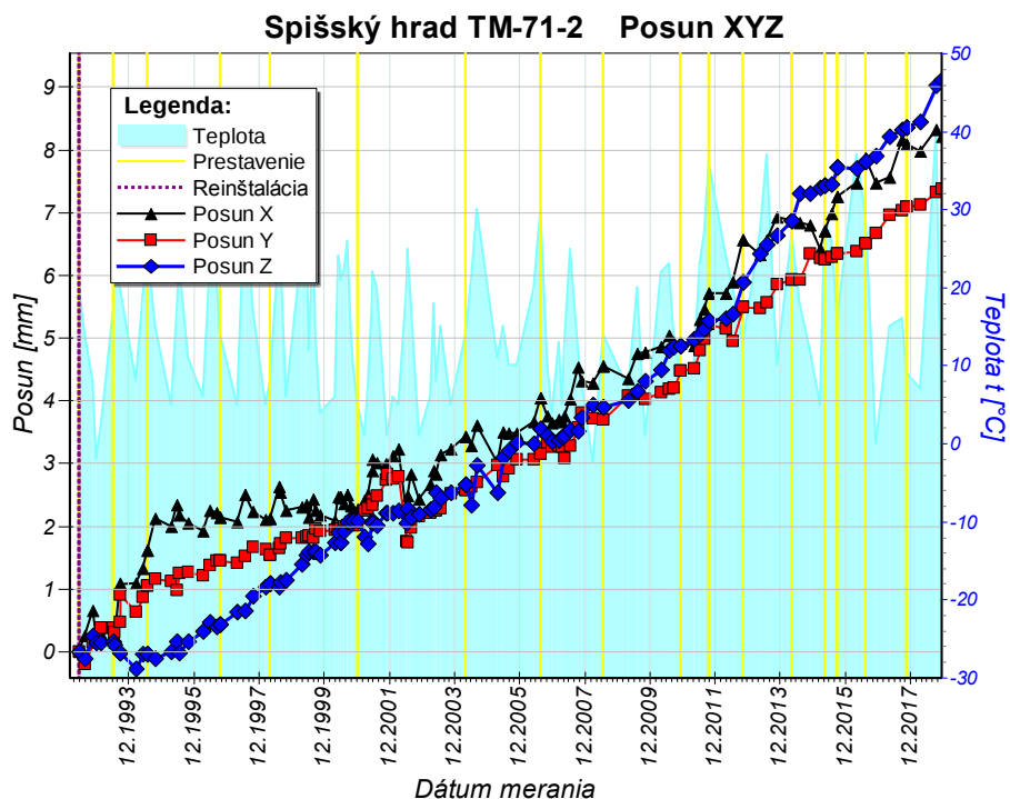
Obr. 11a Graf posunu travertínových blokov pozdĺž osí x, y a z zostavený na základe údajov z dilatometra TM-71-2 za monitorovacie obdobie 1992 – 2018.
