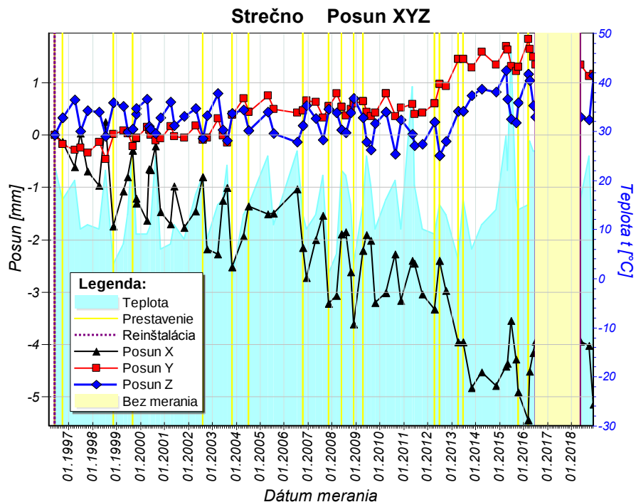
Obr. 23a Graf posunu blokov pozdĺž osí x, y a z zostavený na základe údajov z dilatometra TM-71 inštalovaného v trhline pod kaplnkou hradu Strečno za monitorovacie obdobie 1996 – 2018.
