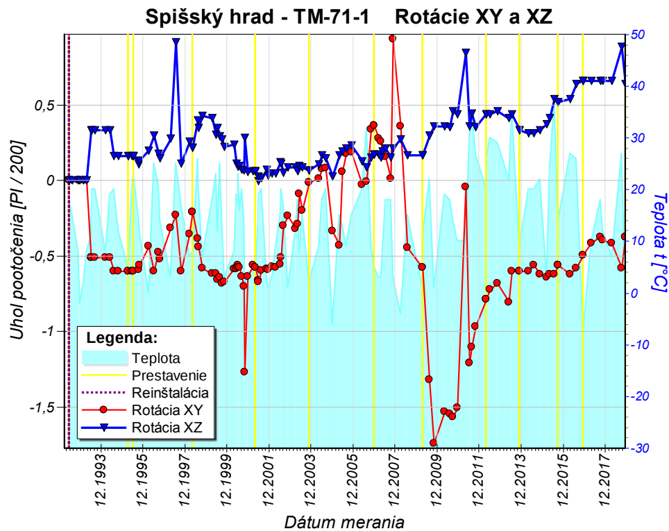
Obr. 8b Graf rotácií travertínových blokov v horizontálnej (XY) a vertikálnej (XZ) rovine zostavený na základe údajov z dilatometra TM-71-1 za monitorovacie obdobie 1992 – 2018.
