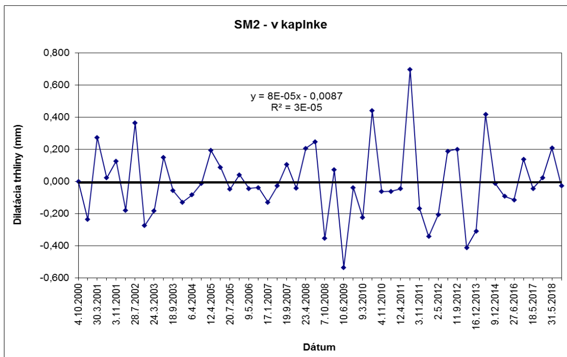
Obr. 31 Výsledky meraní pohybu blokov dilatometrom SM 2 na Uhrovskom hrade v rokoch 2000 – 2018
