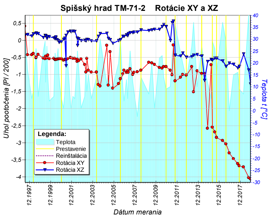
Obr. 11b Graf rotácií travertínových blokov v horizontálnej (XY) a vertikálnej (XZ) rovine zostavený na základe údajov z dilatometra TM-71-2 za monitorovacie obdobie 1992 – 2018.
