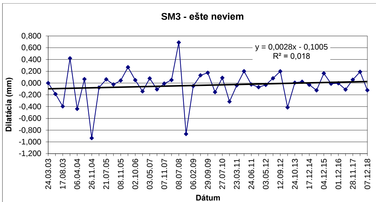
Obr. 36 Výsledky meraní pohybu blokov dilatometrom SM 3 na Pajštúnskom hrade v rokoch 2003 – 2018.
