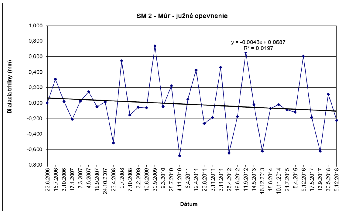
Obr. 26 Výsledky meraní pohybu blokov dilatometrom SM 2 na Trenčianskom hrade v rokoch 2006 – 2018.
