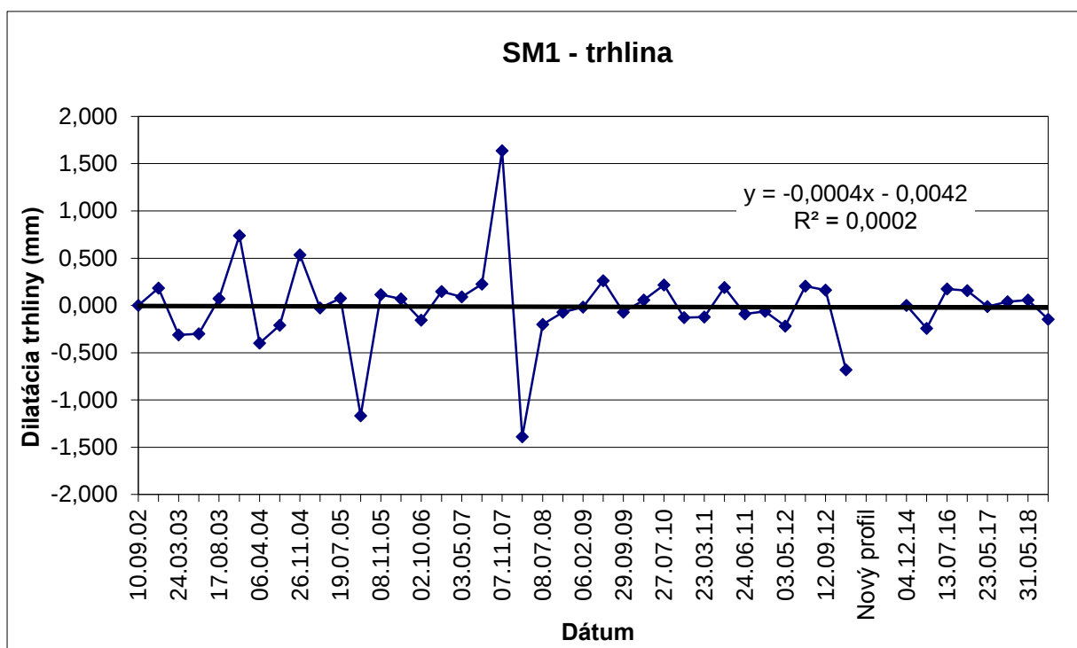
Obr. 39 Výsledky meraní pohybu blokov dilatometrom SM 1 na Plaveckom hrade v rokoch 2002 – 2013 a 2014 – 2018
