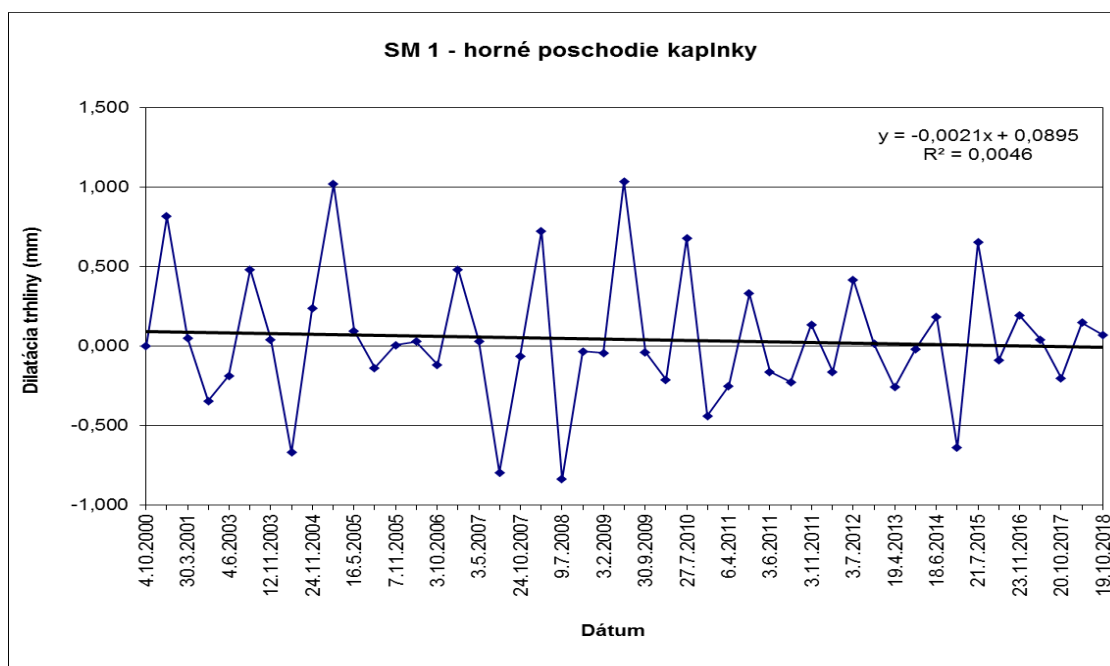
Obr. 30 Výsledky meraní pohybu blokov dilatometrom SM 1 na Uhrovskom hrade v rokoch 2000 – 2018.
