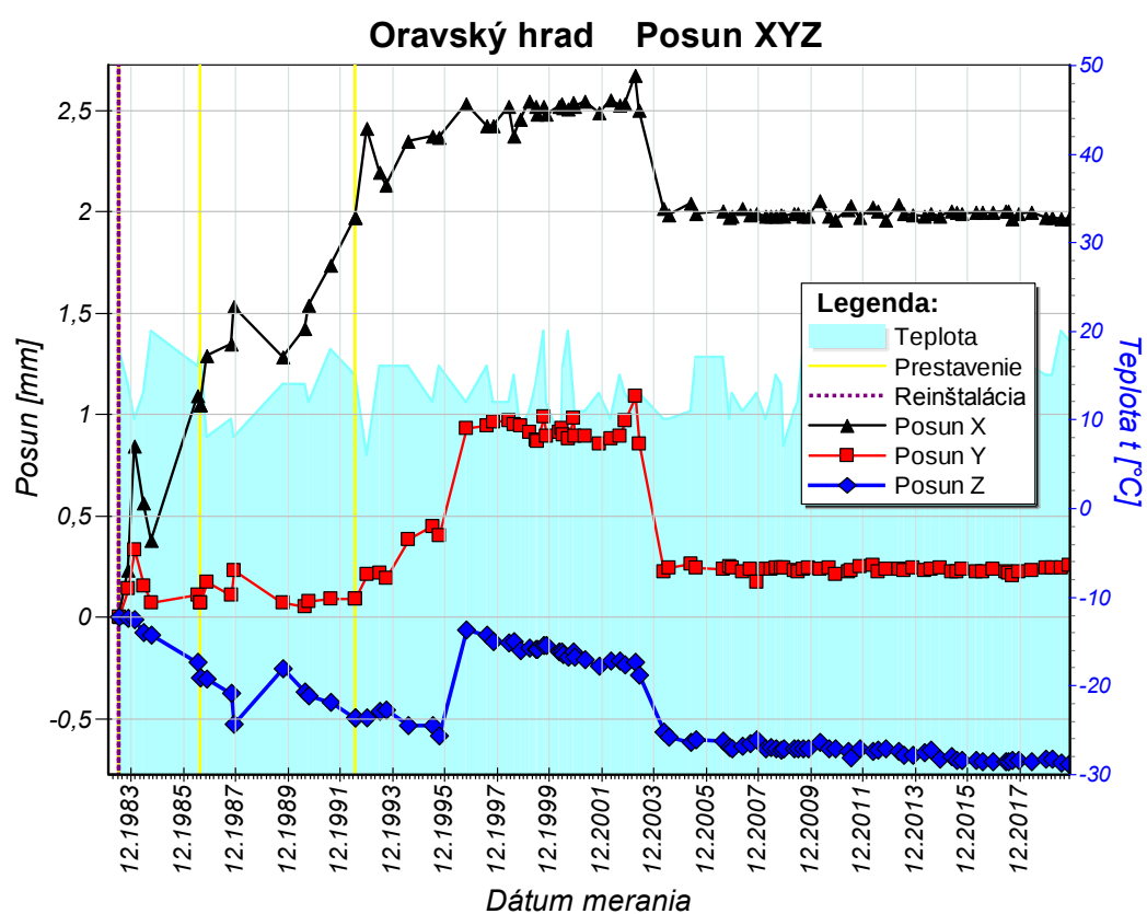
Obr. 21 Graf posunu blokov pozdĺž osí x, y a z zostavený na základe údajov z dilatometra TM-71 (starý typ) na Oravskom hrade za monitorovacie obdobie 1983 – 2018.
