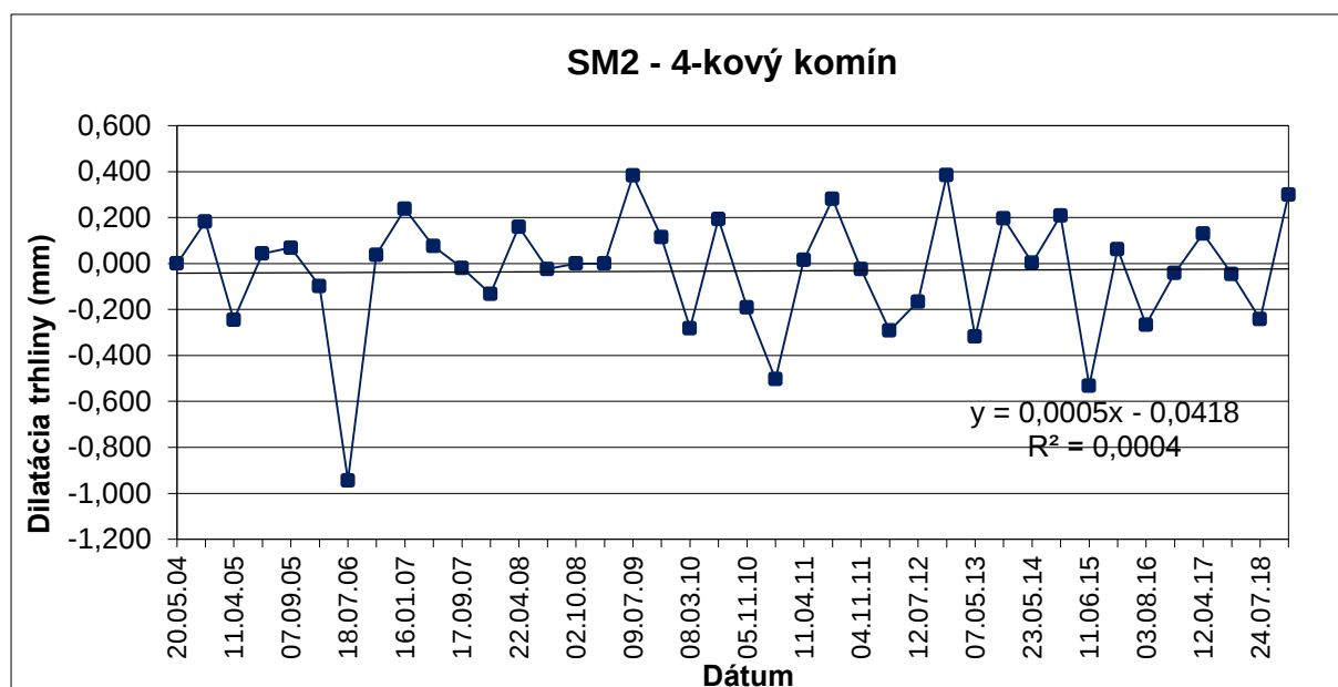
Obr. 35 Výsledky meraní pohybu blokov dilatometrom SM 2 na Pajštúnskom hrade v rokoch 2004 – 2018.
