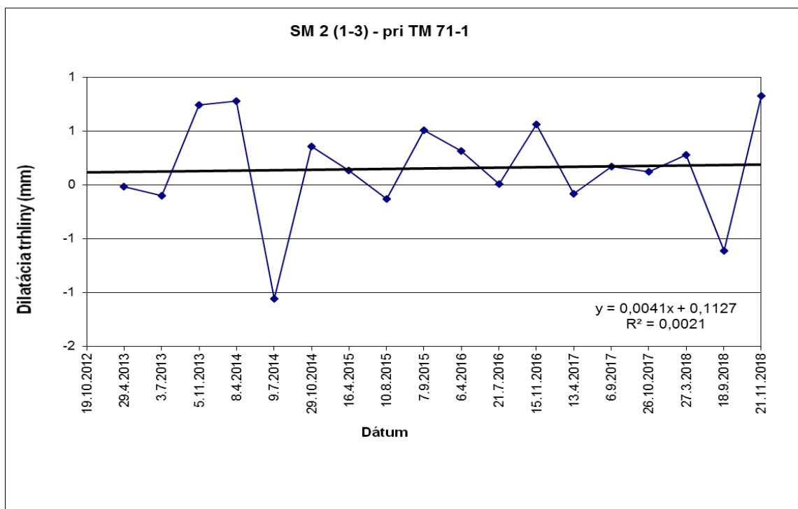
Obr. 9 Výsledky meraní pohybu blokov dilatometrom SM 2 (medzi monitorovacími bodmi 1 – 3) na lokalite Spišský hrad v rokoch 2012 – 2018
