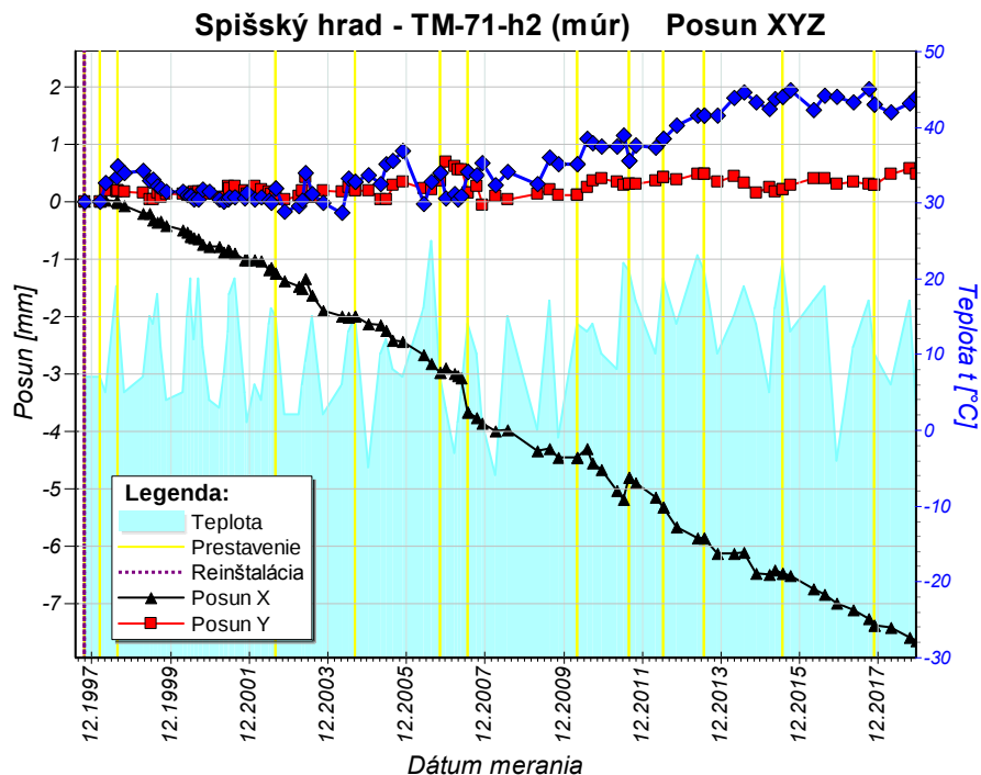
Obr. 14a Graf posunu travertínových blokov pozdĺž osí x, y, z zostavený na základe údajov z dilatometra TM-71-h2 (múr) za monitorovacie obdobie 1997 – 2018.
