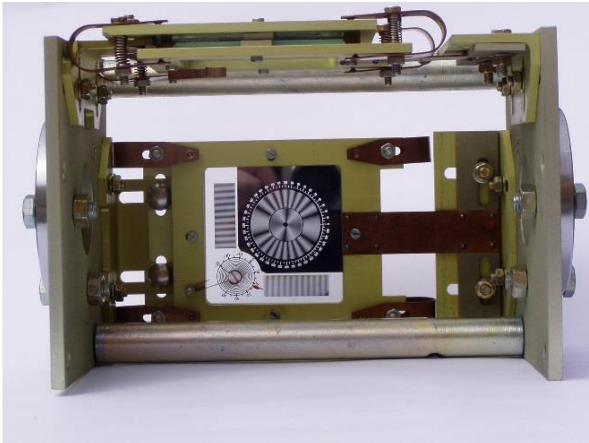
Obr. 2 Mechanicko-optický dilatometer typu TM-71.
