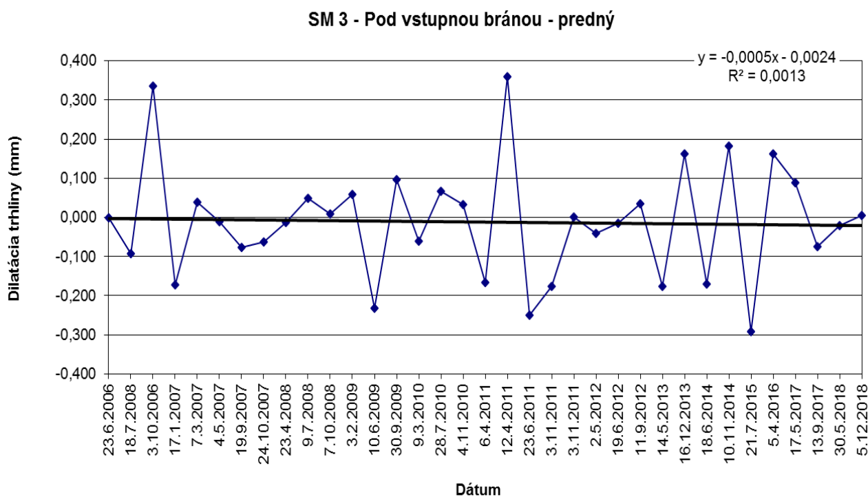
Obr. 27 Výsledky meraní pohybu blokov dilatometrom SM 3 na Trenčianskom hrade v rokoch 2006 – 2018.
