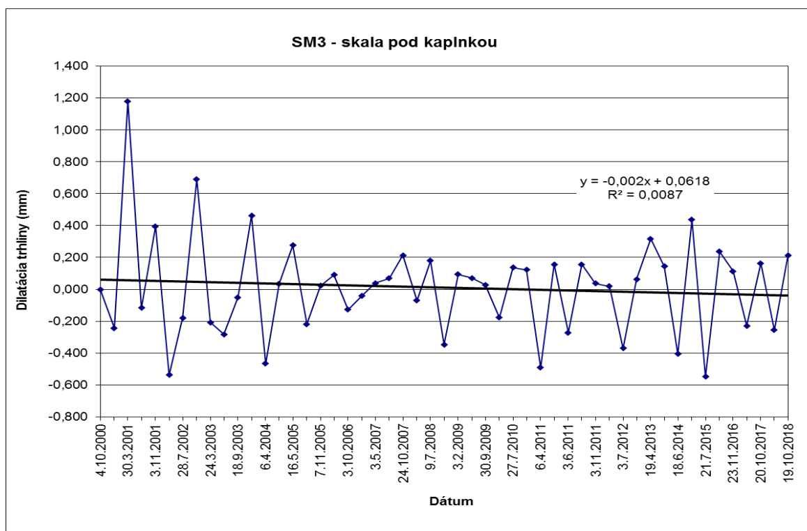
Obr. 32 Výsledky meraní pohybu blokov dilatometrom SM 3 na Uhrovskom hrade v rokoch 2000 – 2018
