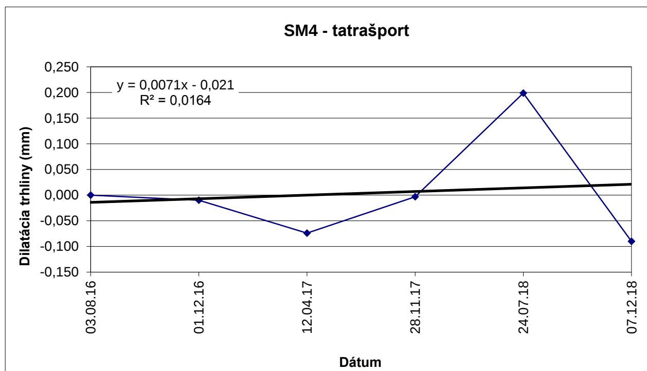
Obr. 37 Výsledky meraní pohybu blokov dilatometrom SM 4 na Pajštúnskom hrade v rokoch 2016 – 2018.
