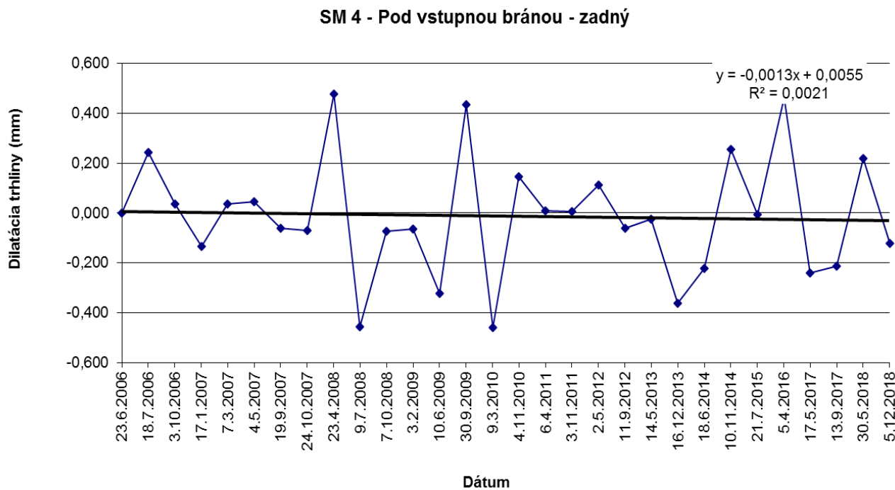
Obr. 28 Výsledky meraní pohybu blokov dilatometrom SM 4 na Trenčianskom hrade v rokoch 2006 – 2018.
