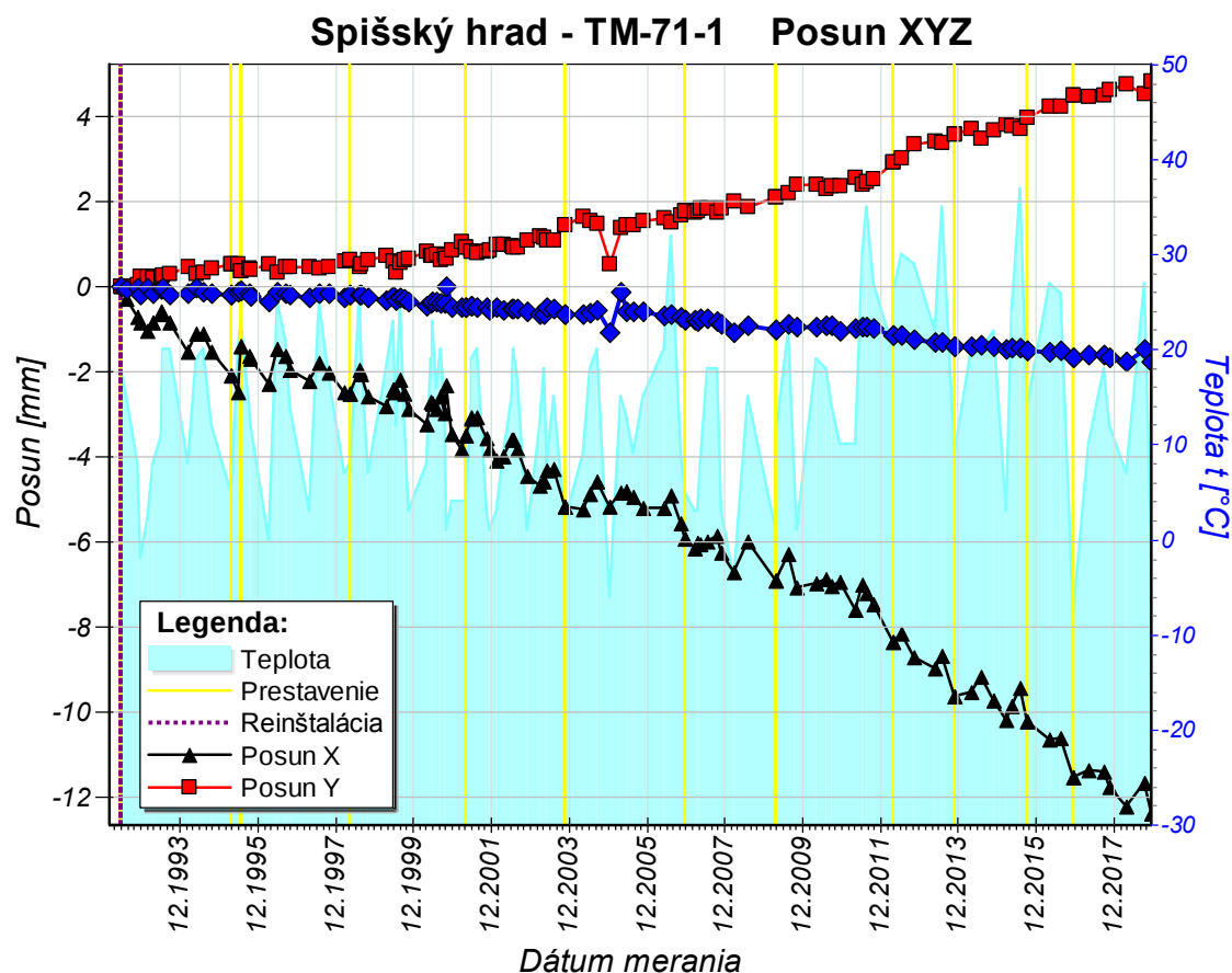
Obr. 8a Graf posunu travertínových blokov pozdĺž osí x, y a z zostavený na základe údajov z dilatometra TM- 71-1 za monitorovacie obdobie 1992 – 2018.
