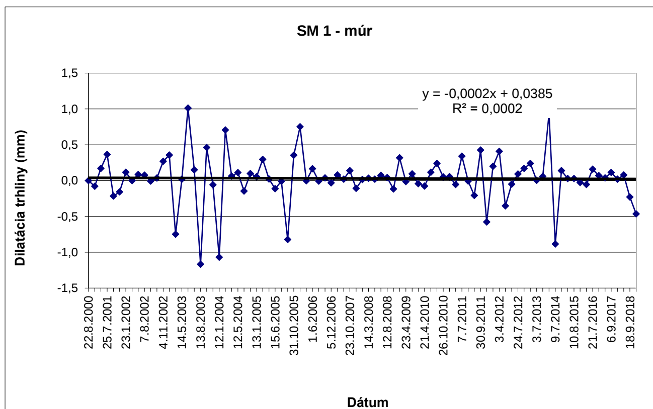
Obr.15 Výsledky meraní pohybu blokov dilatometrom SM 1 na lokalite Spišský hrad v rokoch 2000 – 2018
