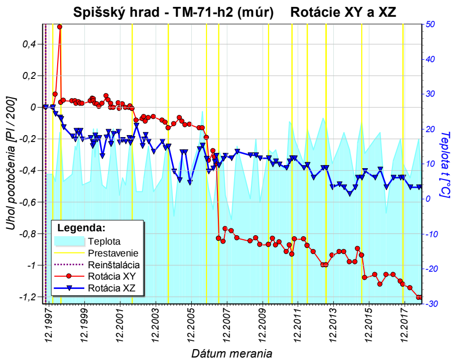
Obr. 14b Graf rotácií travertínových blokov v horizontálnej (XY) a vertikálnej (XZ) rovine zostavený na základe údajov z dilatometra TM-71-h2 (múr) za monitorovacie obdobie 1997 – 2018.
