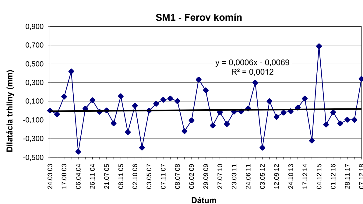
Obr. 34 Výsledky meraní pohybu blokov dilatometrom SM 1 na Pajštúnskom hrade v rokoch 2003 – 2018.
