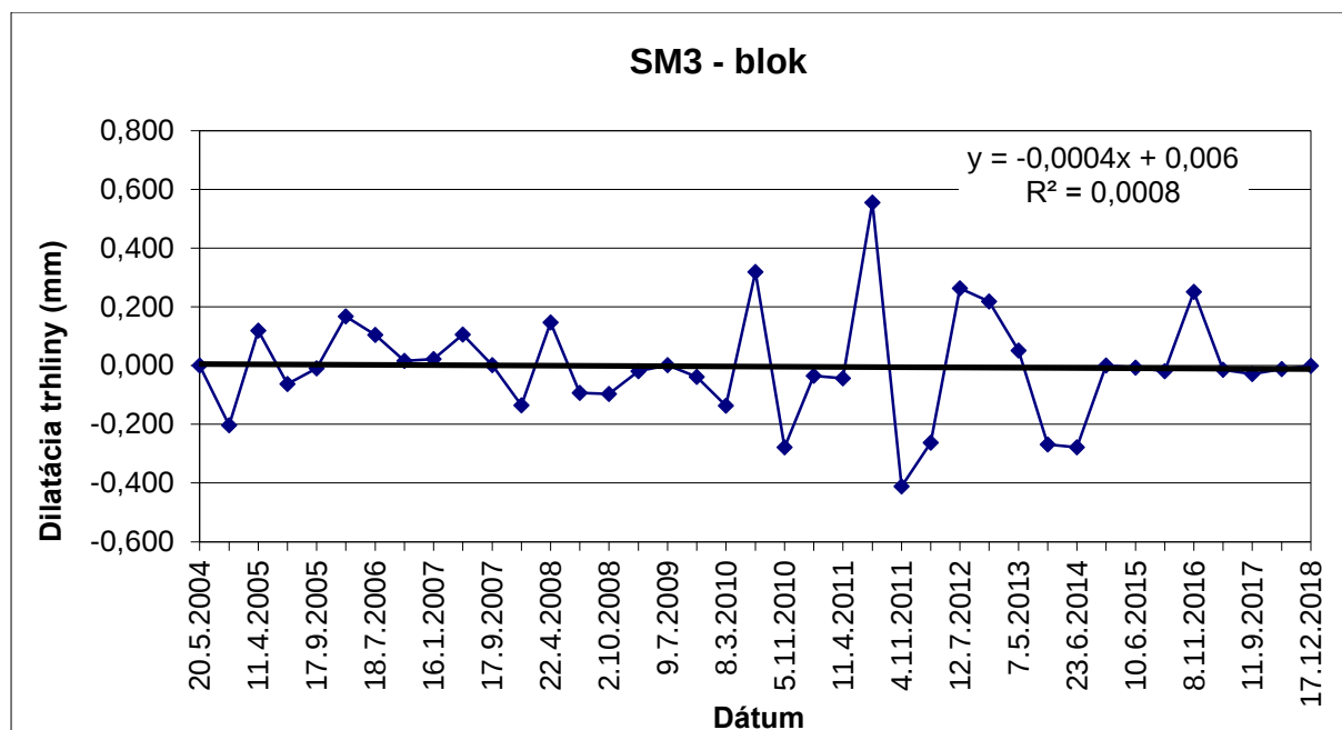
Obr. 41 Výsledky meraní pohybu blokov dilatometrom SM3 na Plaveckom hrade v rokoch 2004 – 2018.
