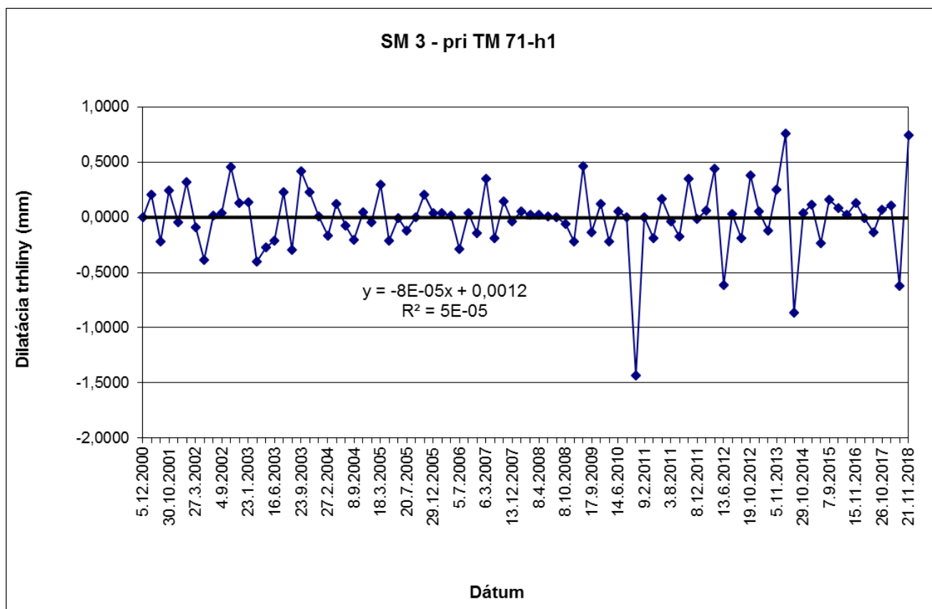
Obr. 7 Výsledky meraní pohybu blokov dilatometrom SM 3 na Spišskom hrade v období rokov 2000 – 2018
