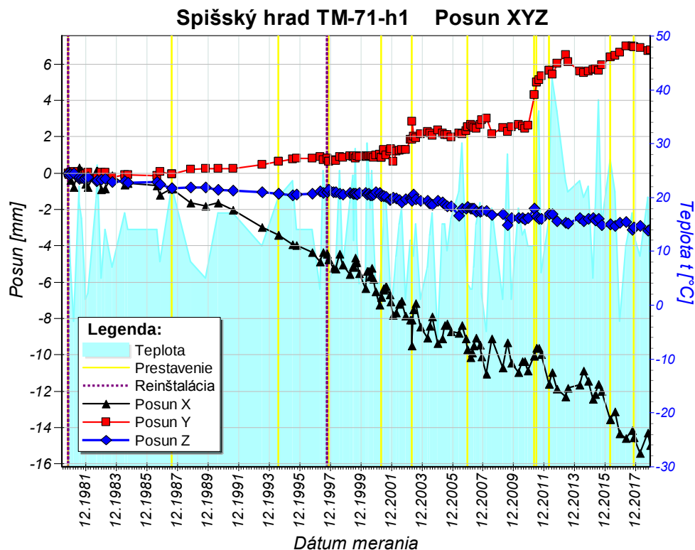
Obr. 6 Graf posunu travertínových blokov pozdĺž osí x, y a z zostavený na základe údajov z dilatometra TM- 71- h1 za monitorovacie obdobie 1980 – 2018.
