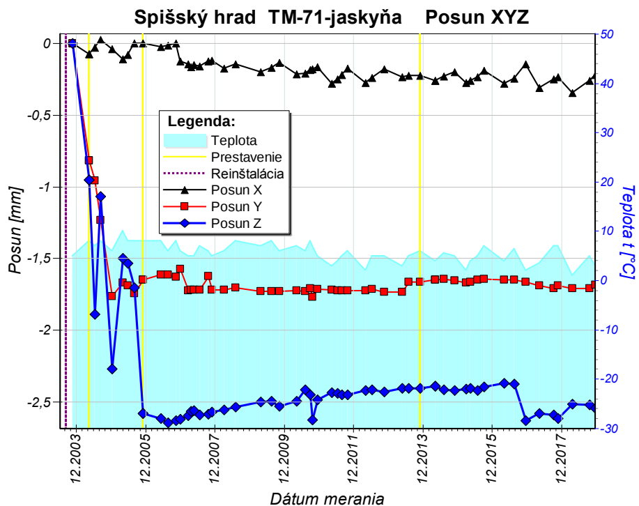
Obr. 17a Graf posunu travertínových blokov pozdĺž osí x , y a z zostavený na základe údajov z dilatometra TM- 71-jaskyňa za monitorovacie obdobie 2003 – 2018.
