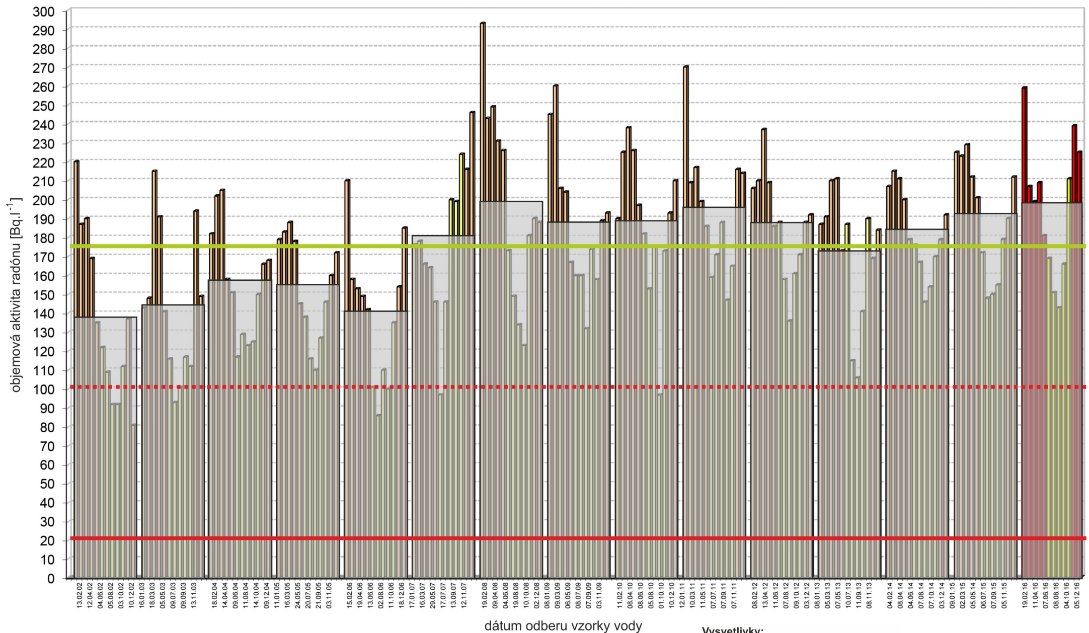
Obr. č. 6 Radón vo vodách: monitorovanie objemovej aktivity radónu v rokoch 2002 - 2016 Lokalita: Spišské Podhradie, prameň sv. Ondreja
