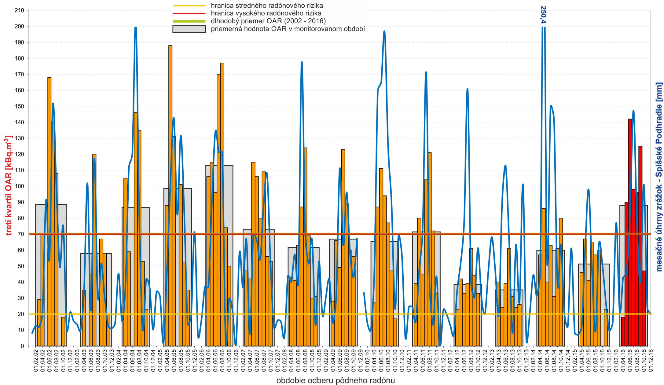
Obr. č. 2 Pôdny radón: monitorovanie objemovej aktivity radónu (OAR) v rokoch 2002 - 2016 Lokalita: Novoveská Huta
