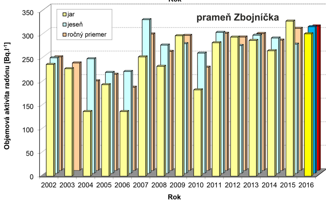
Obr. č. 8 Radón vo vodách: monitorovanie objemovej aktivity radónu v rokoch 2002 - 2016 Lokality: Bratislava - pramene Mária, Himligárka, Zbojnička; Oravice - pramenisko Jašterčie
