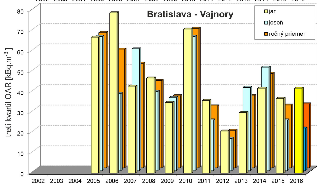
Obr. č. 4 Pôdny radón: monitorovanie objemovej aktivity radónu (OAR) v rokoch 2002 - 2016 Lokality: Hnilec, Bratislava - Vajnory, Banská Bystrica - Podlavice
