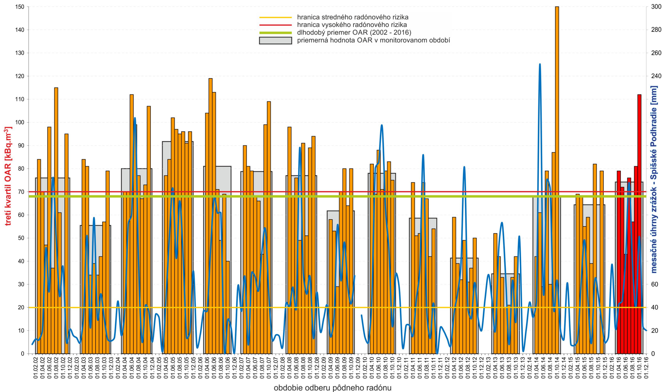
Obr. č. 3 Pôdny radón: monitorovanie objemovej aktivity radónu (OAR) v rokoch 2002 - 2016 Lokalita: Teplička
