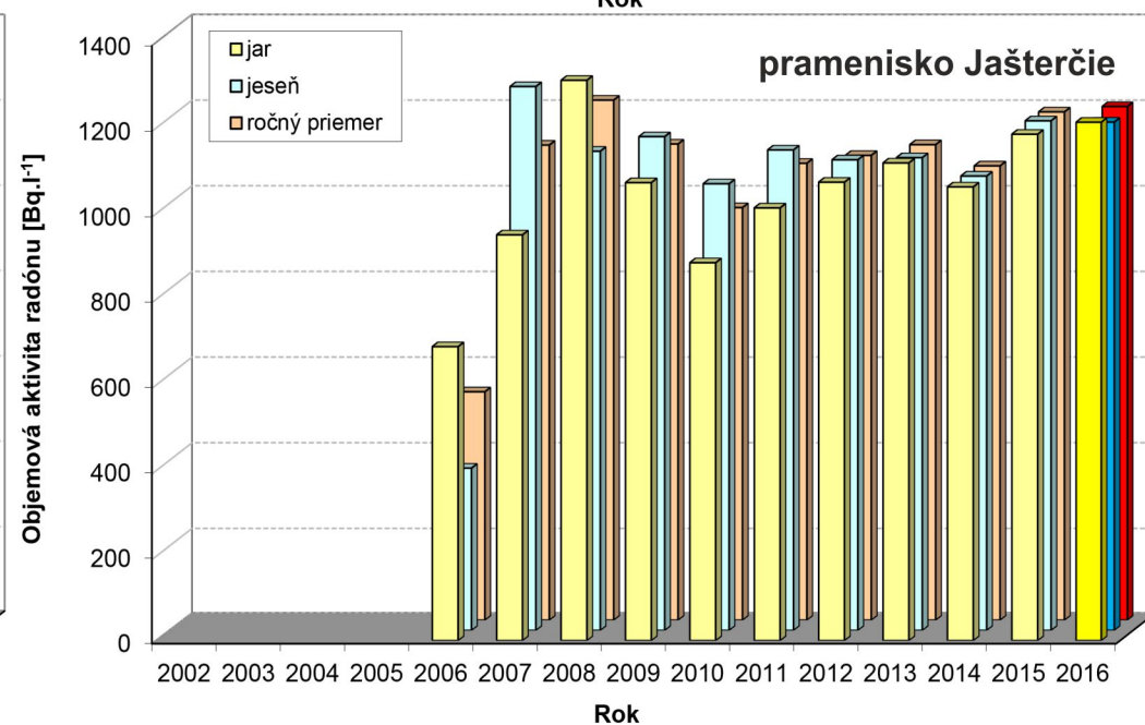
Obr. č. 8 Radón vo vodách: monitorovanie objemovej aktivity radónu v rokoch 2002 - 2016 Lokality: Bratislava - pramene Mária, Himligárka, Zbojnička; Oravice - pramenisko Jašterčie
